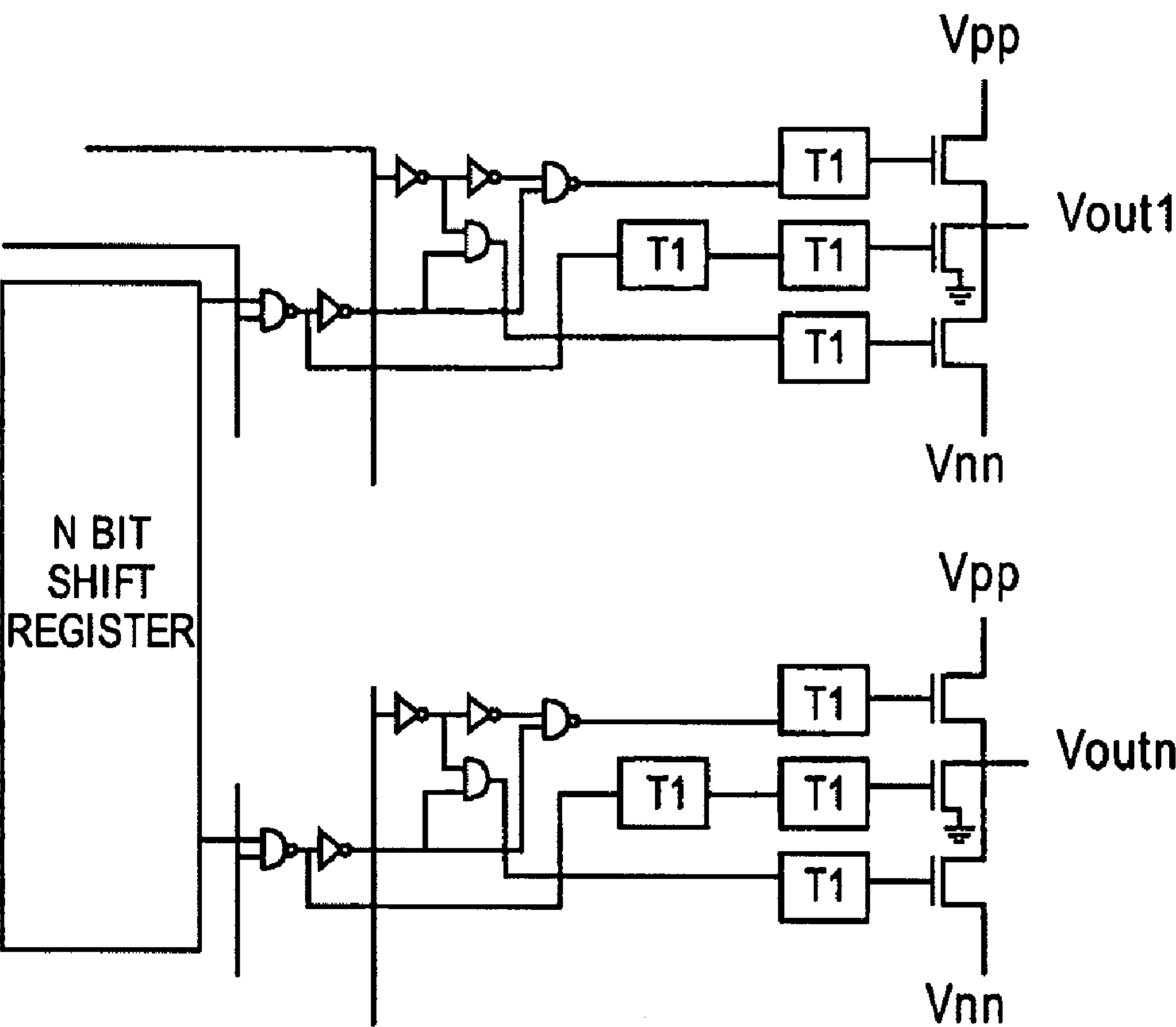
FIG. 10B
