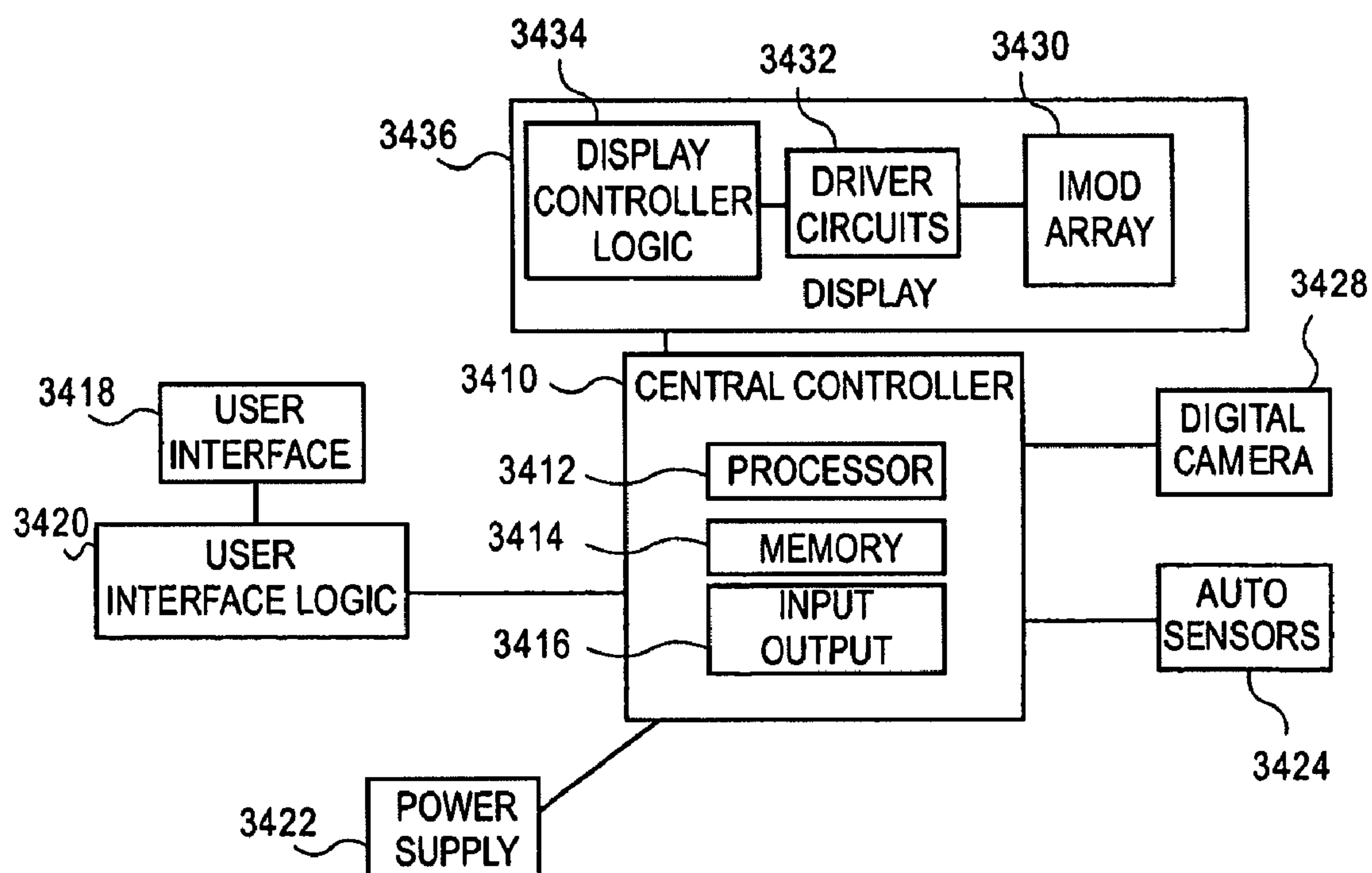
FIG. 34C
