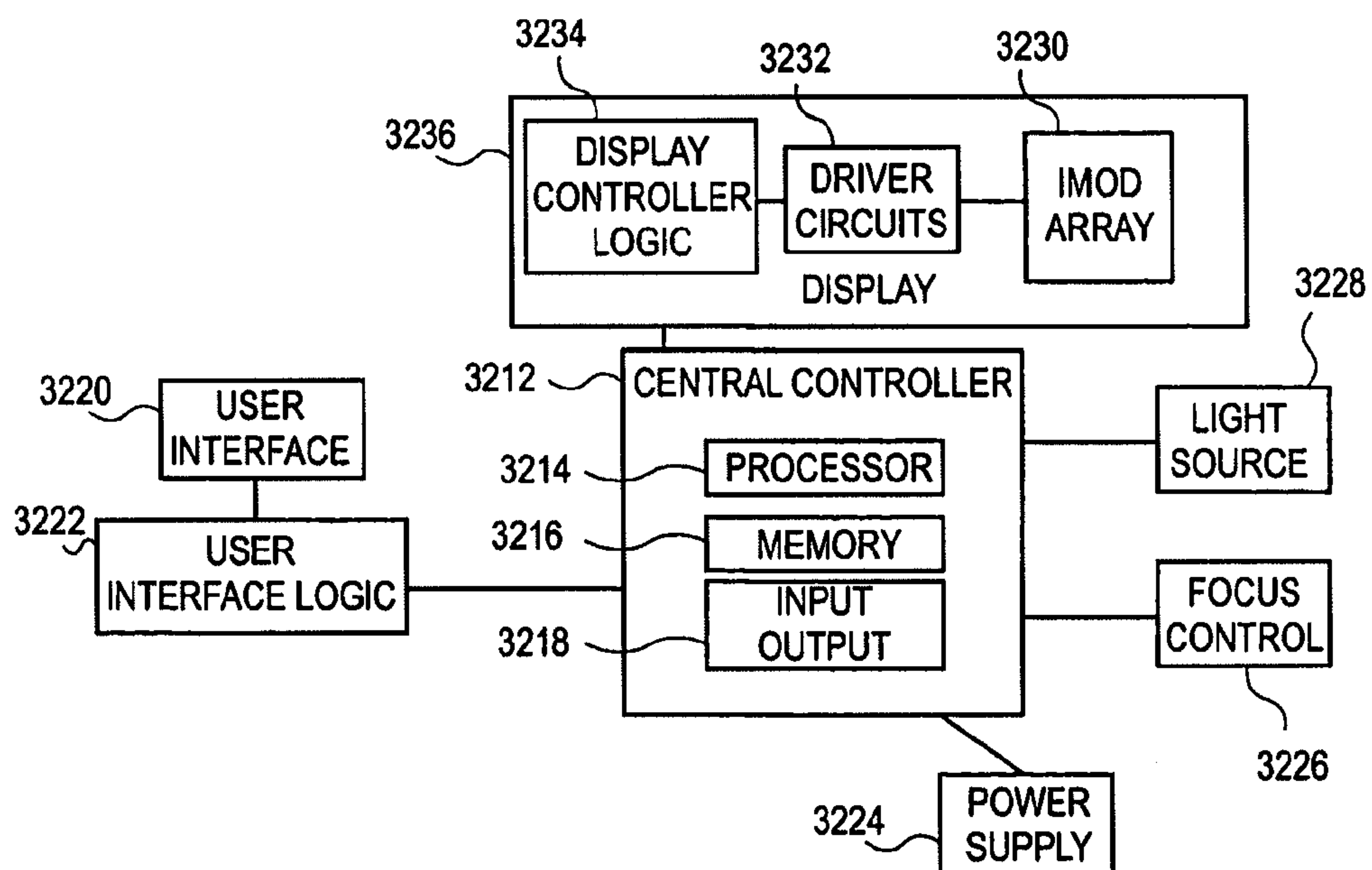
FIG. 32B
