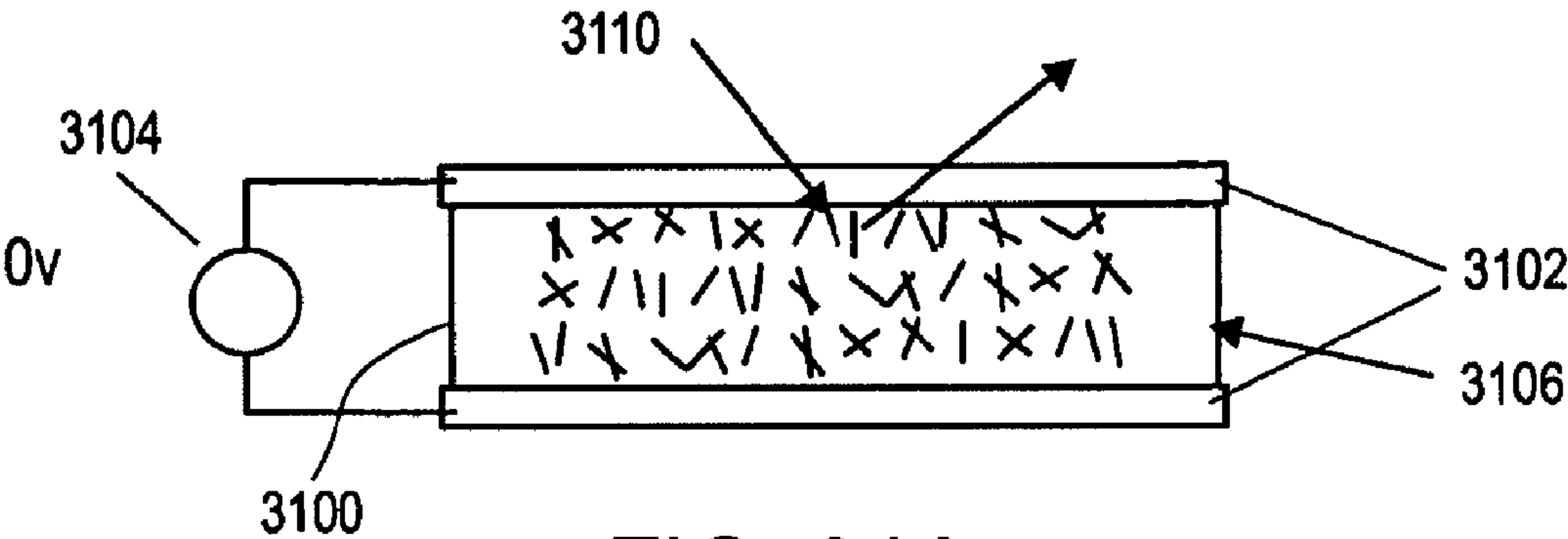
FIG. 31A
