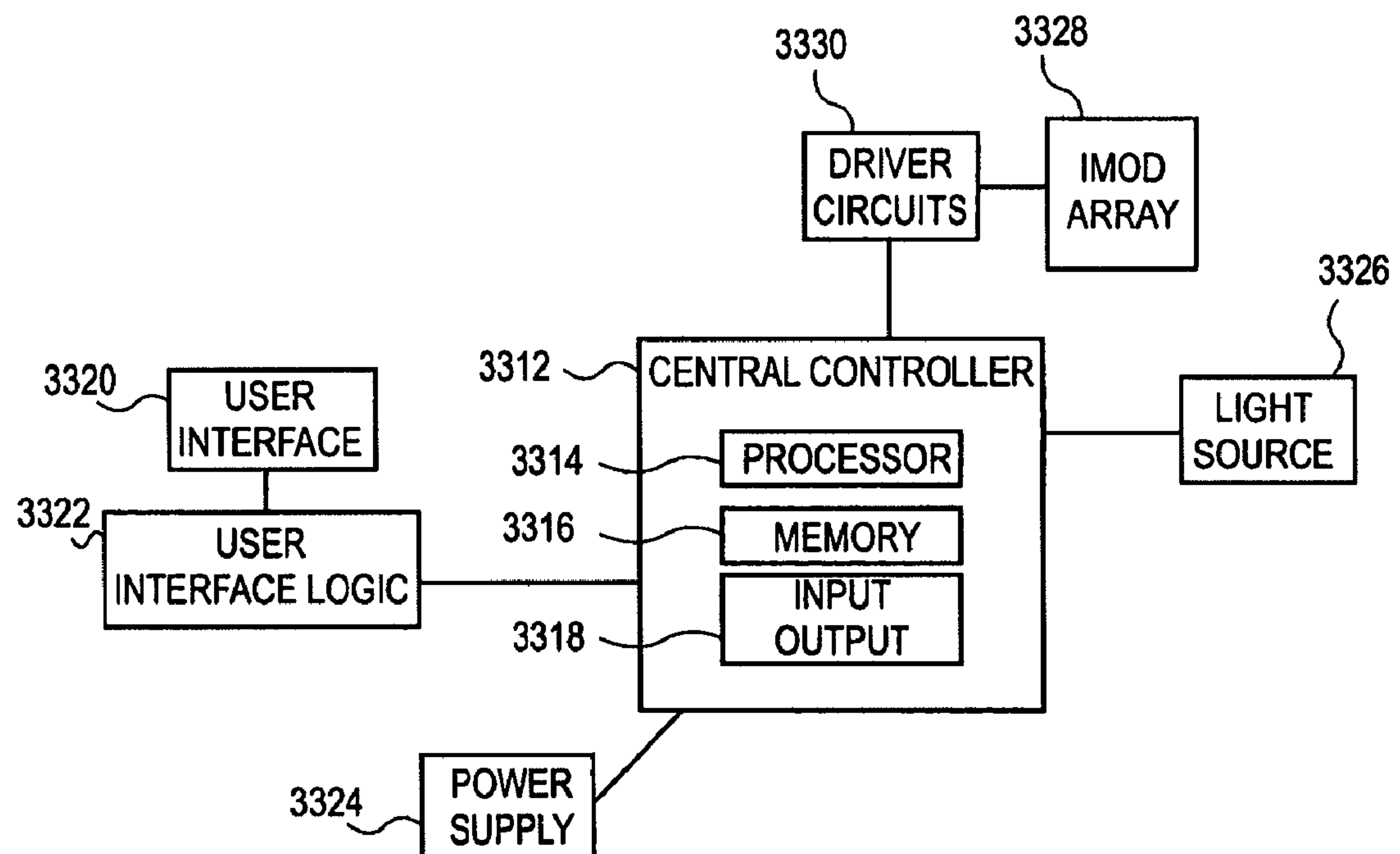
FIG. 33B
