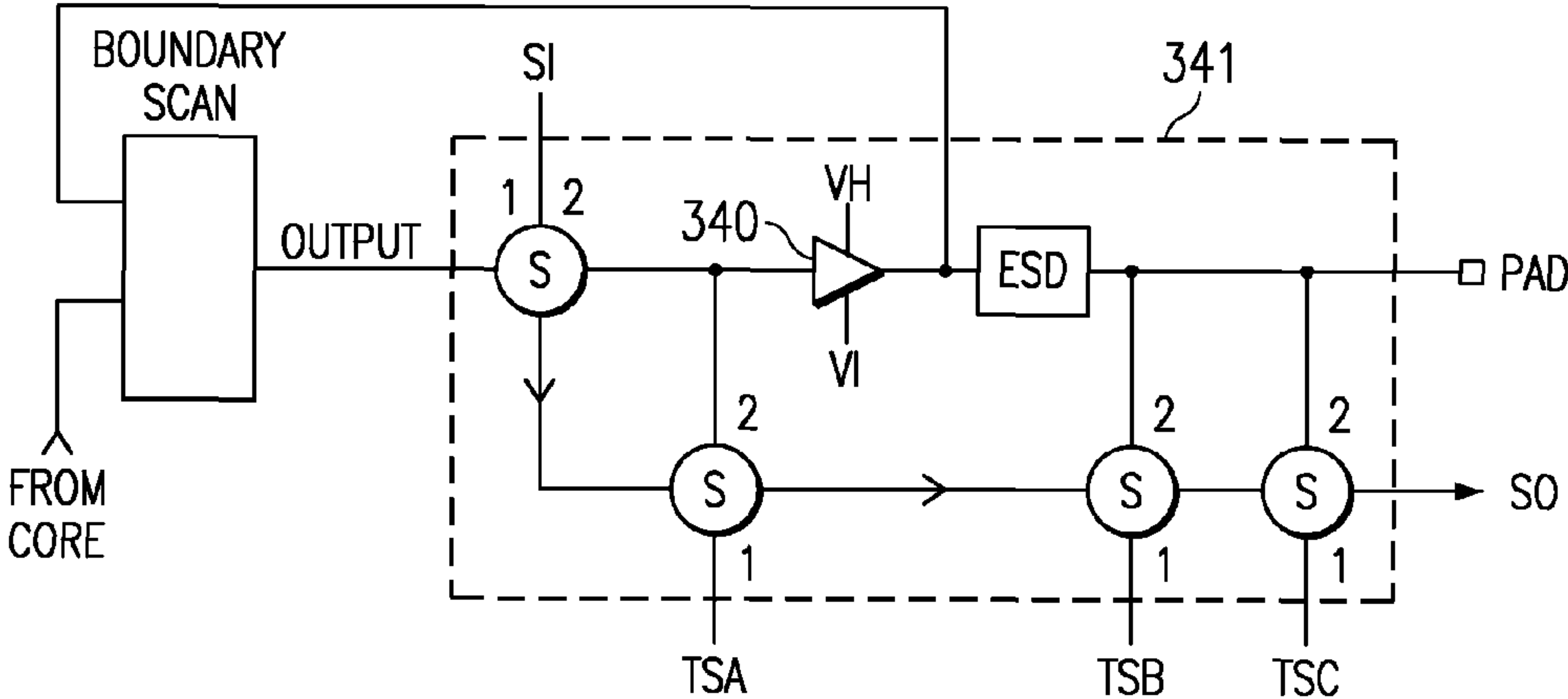
FIG. 34
