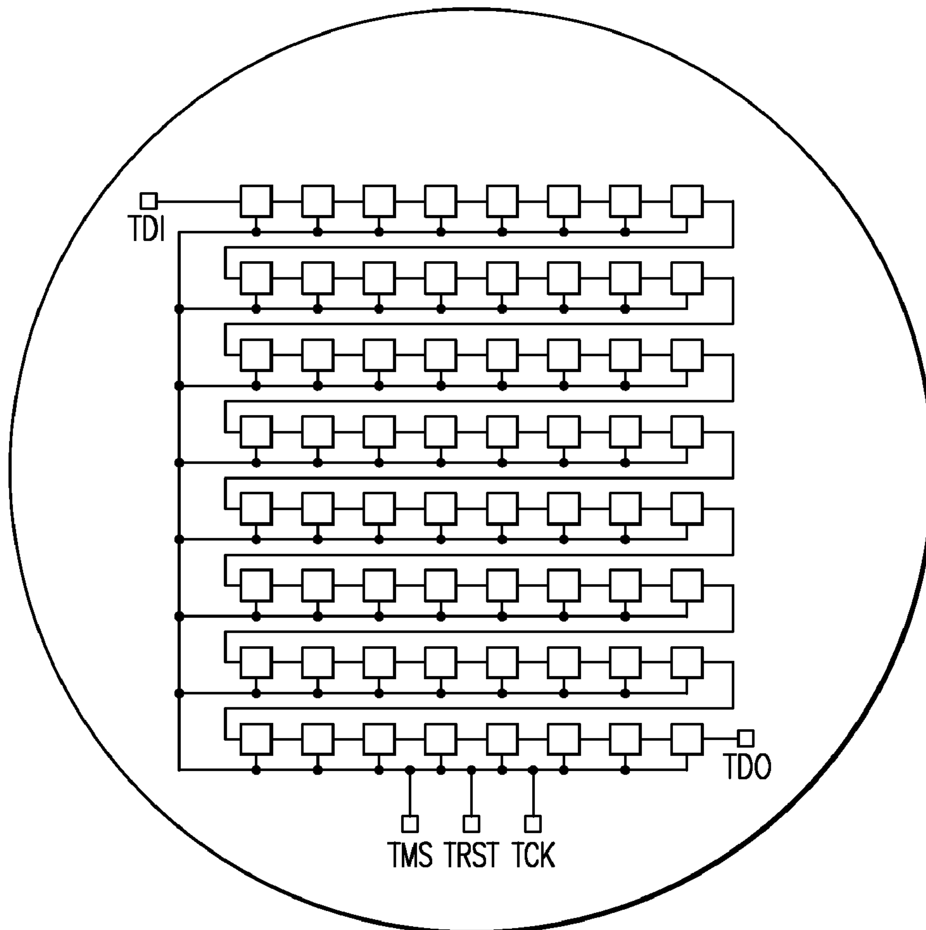
FIG. 26
