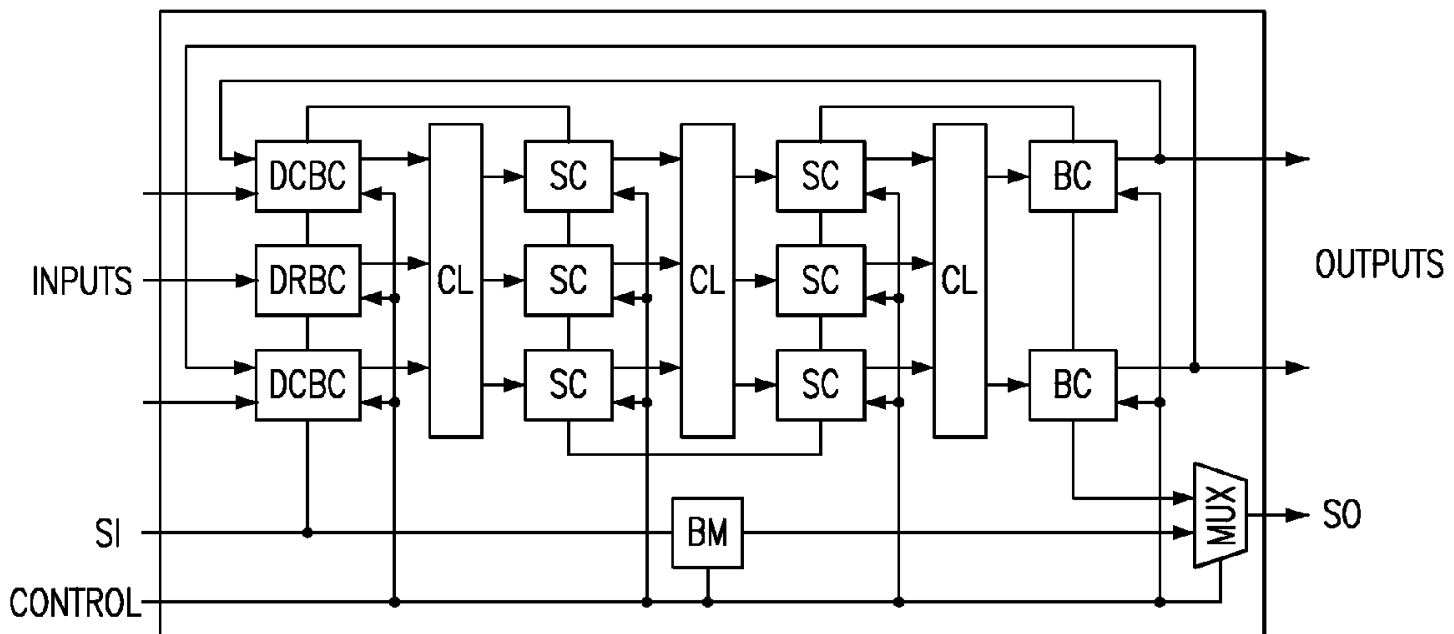
FIG. 18
