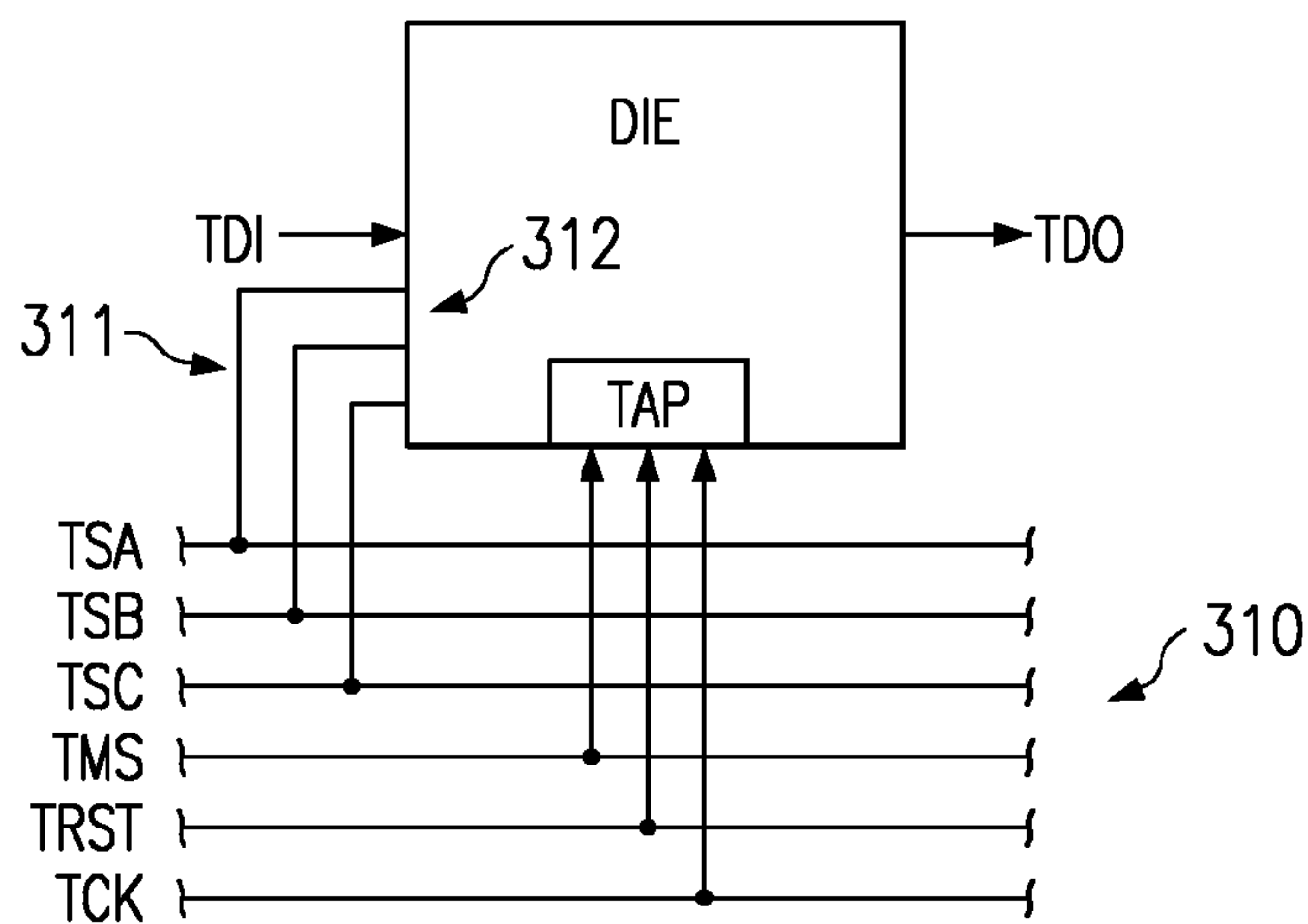
FIG. 32
