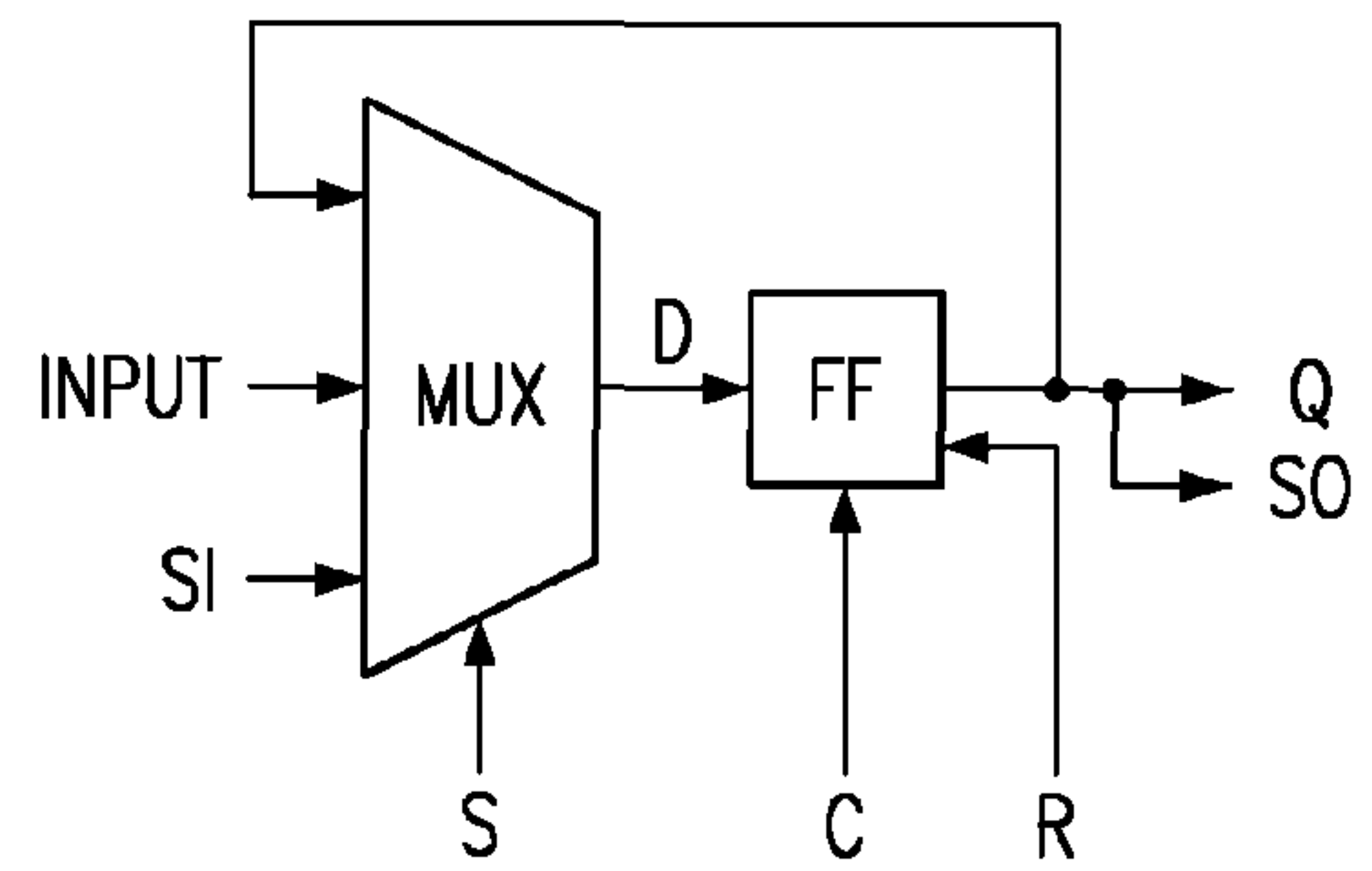
FIG. 15
