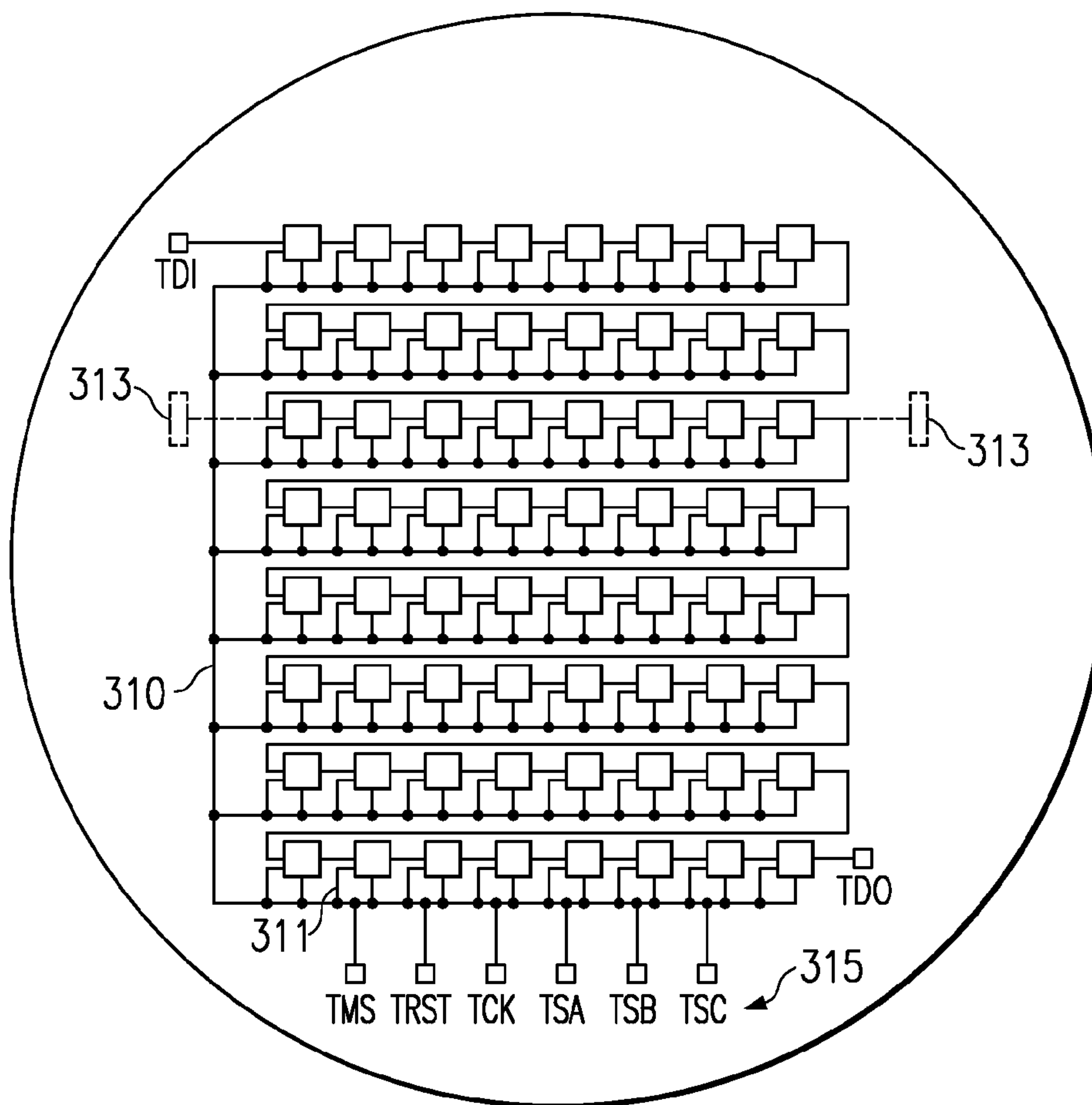
FIG. 31
