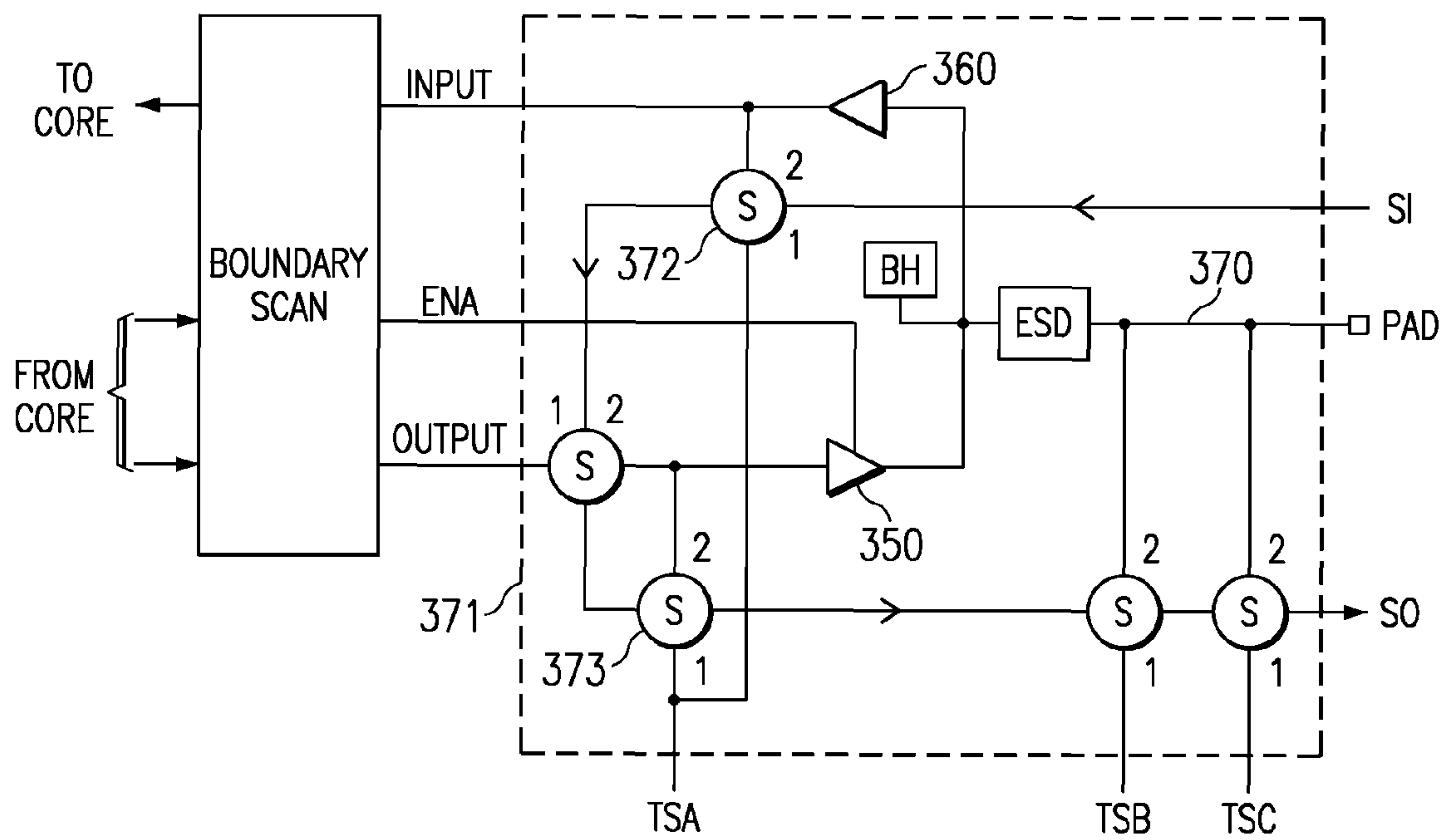
FIG. 37
