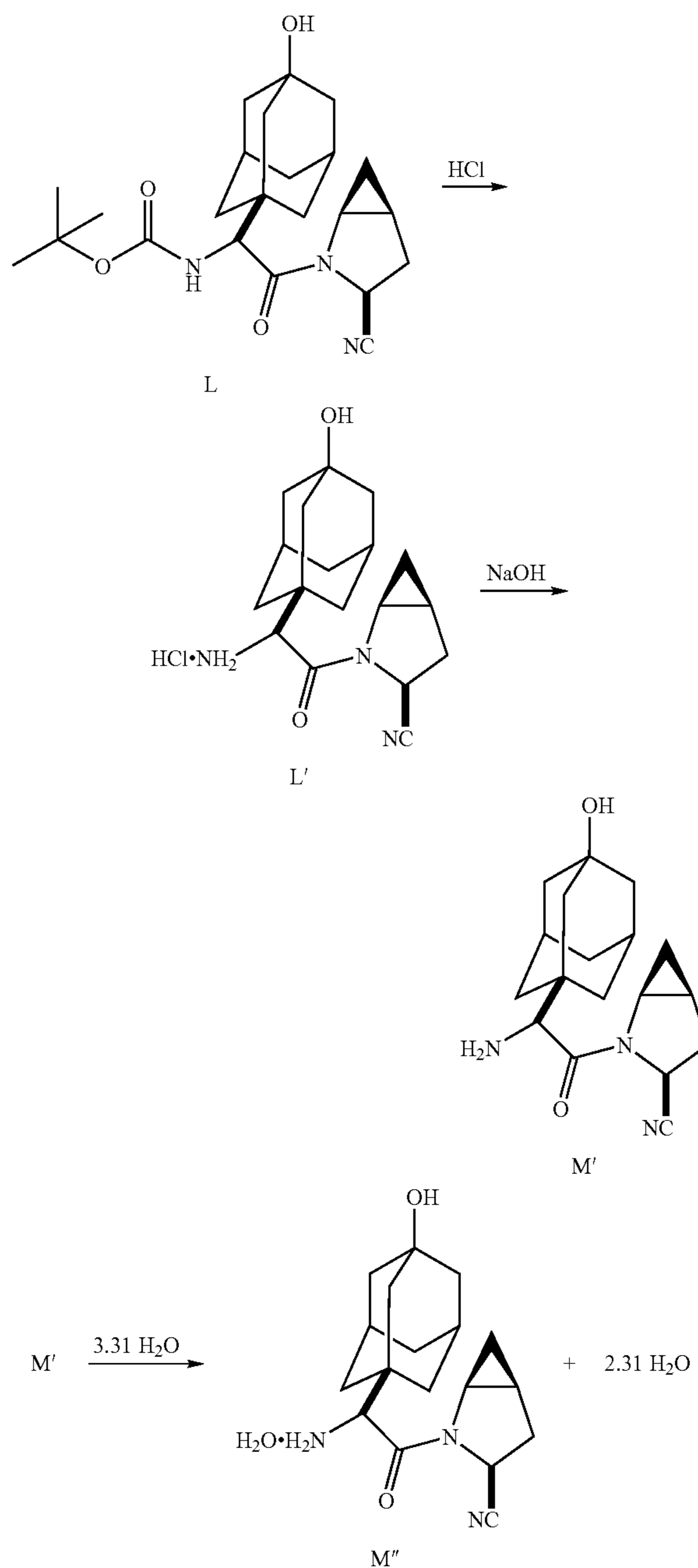
SCHEME VIIB
