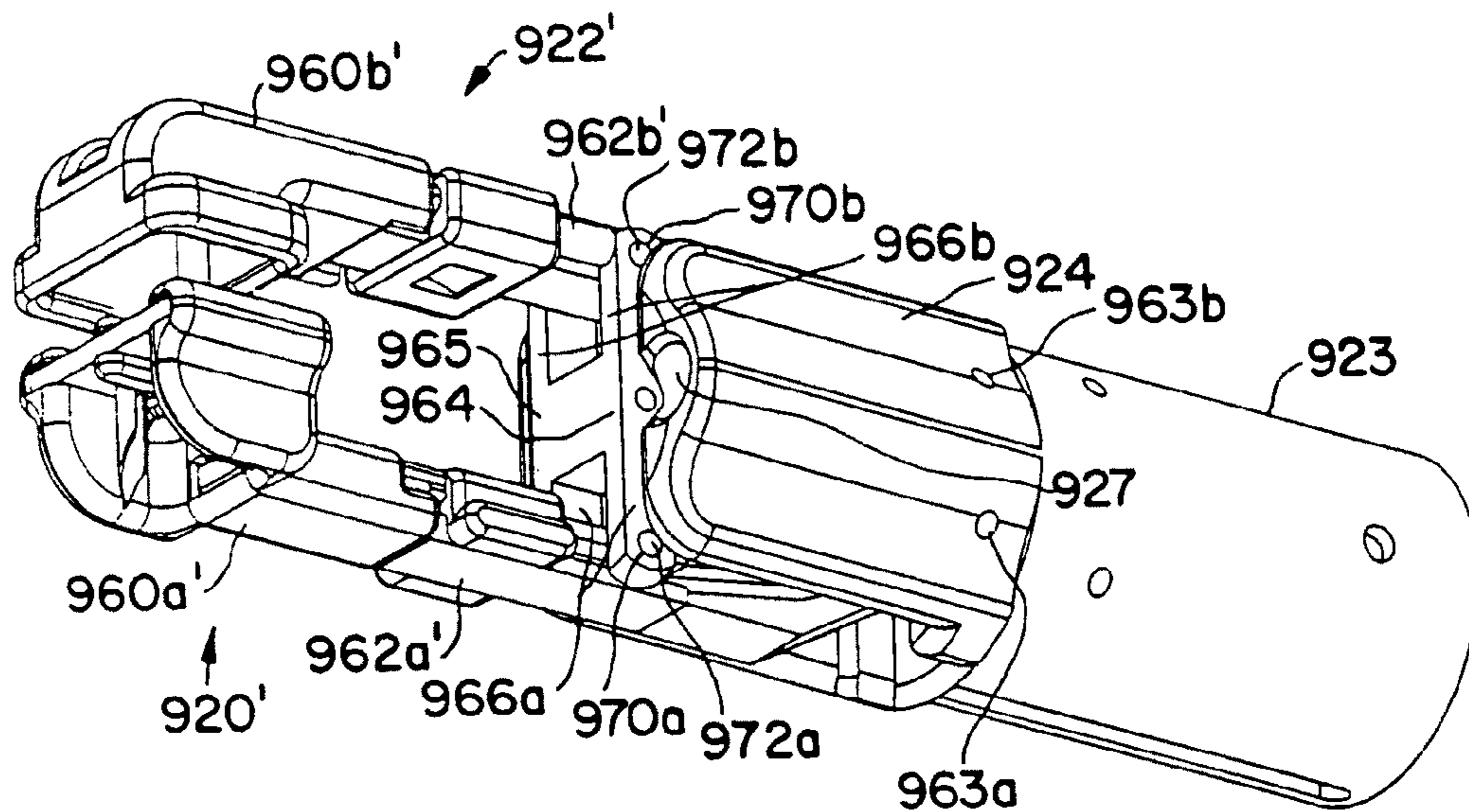
FIG. 41A
