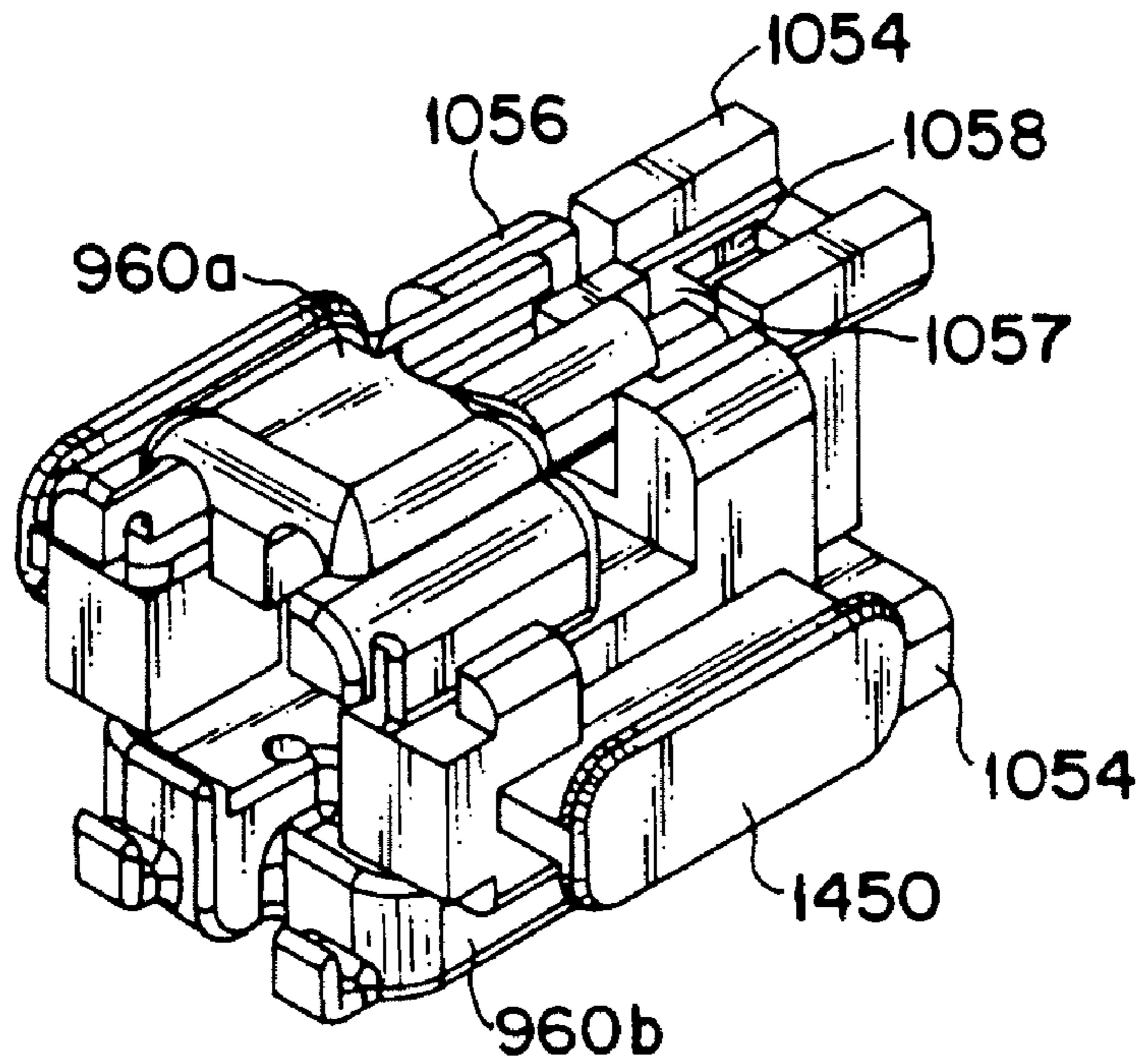
FIG. 46A
