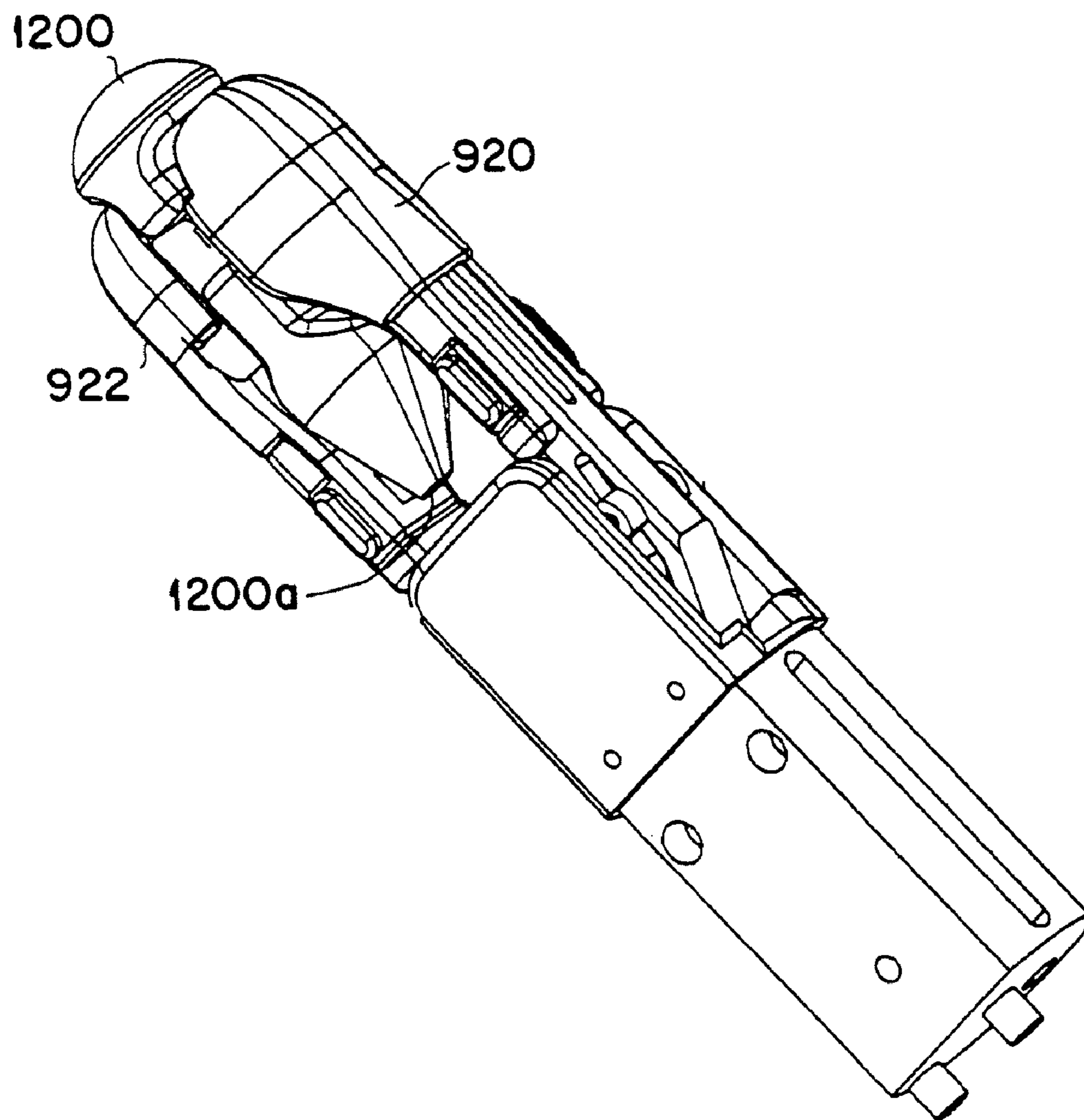
FIG. 37
