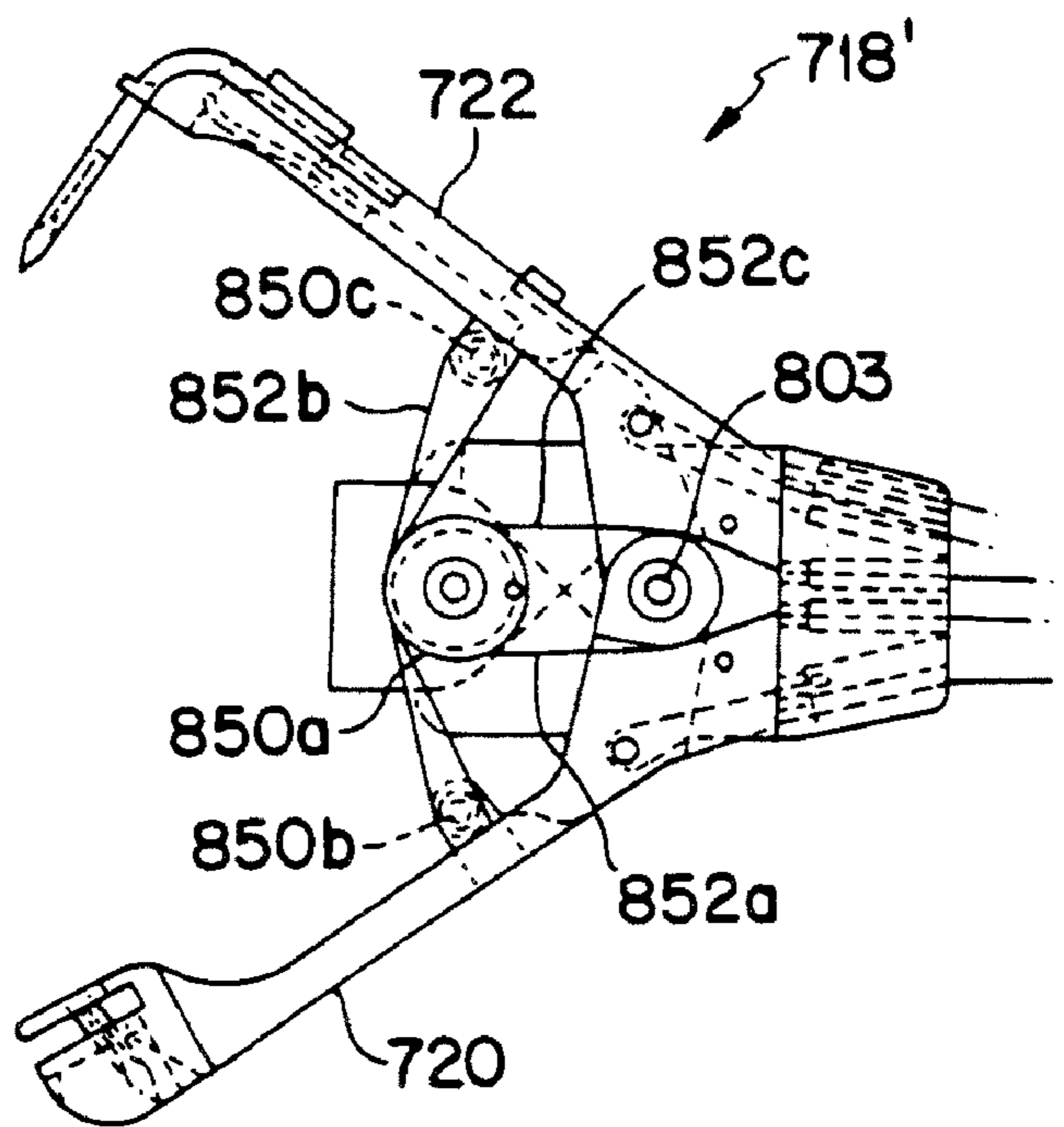
FIG. 11B
