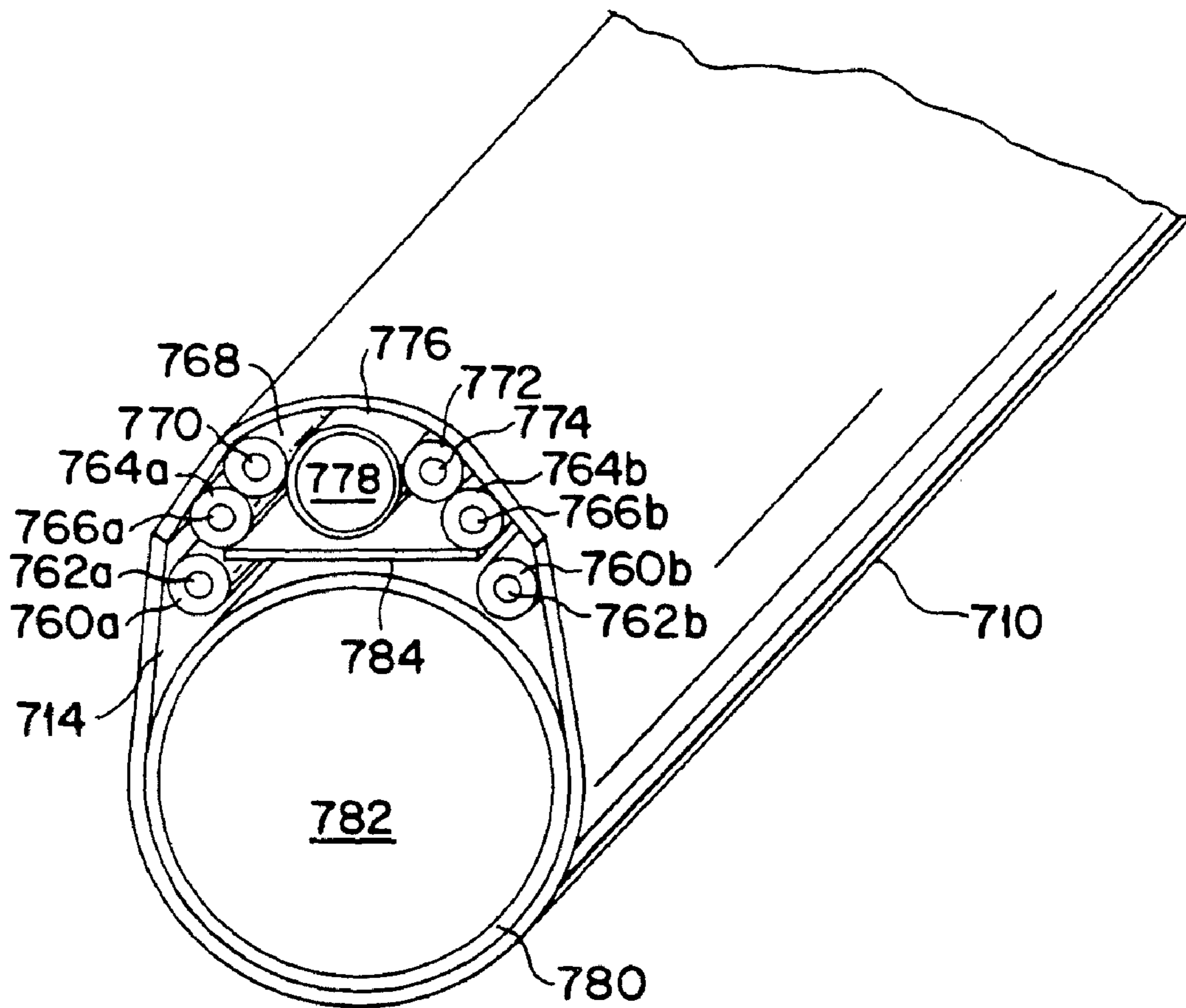
FIG. 3C
