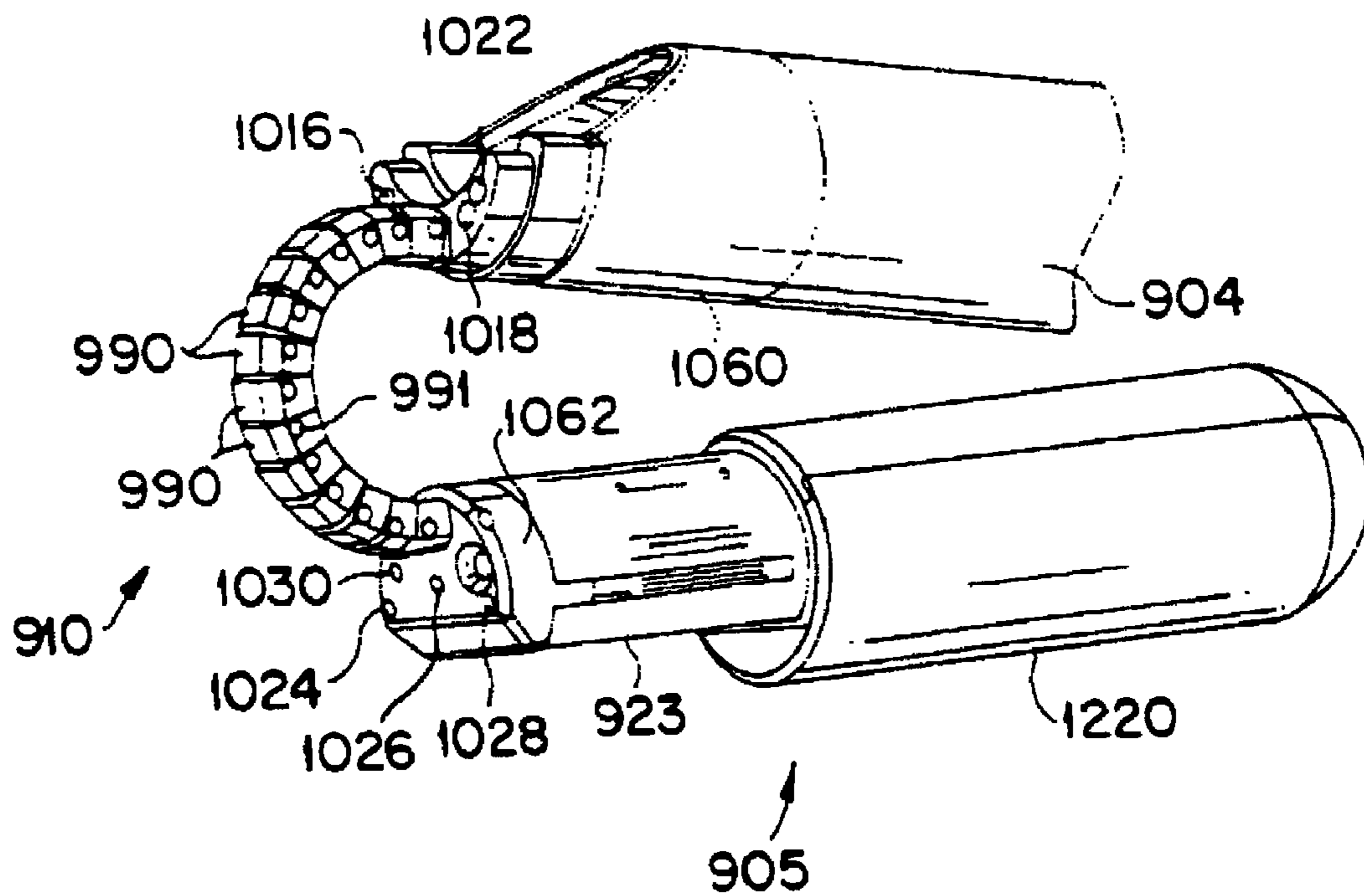
FIG. 24A
