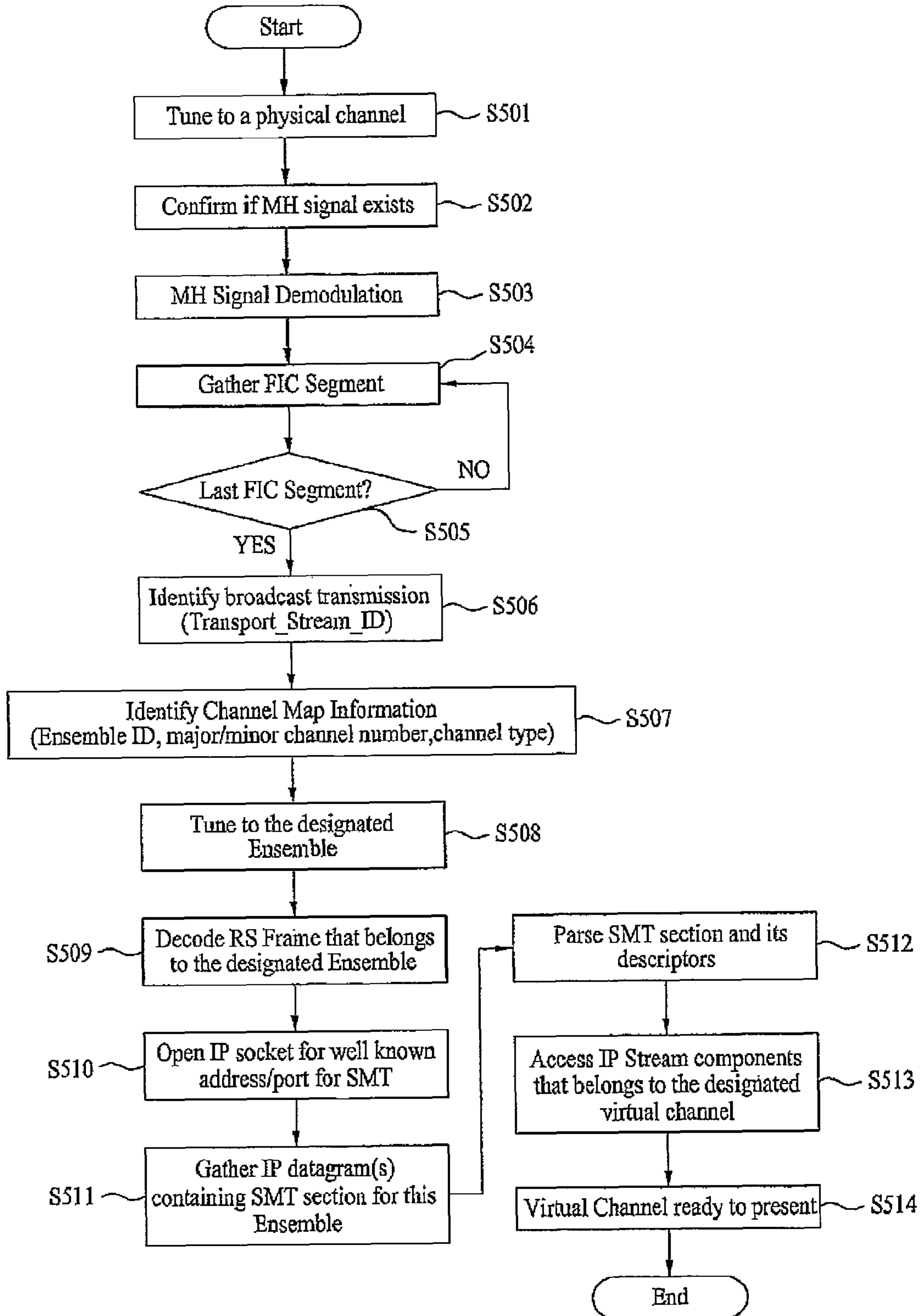
FIG. 28
