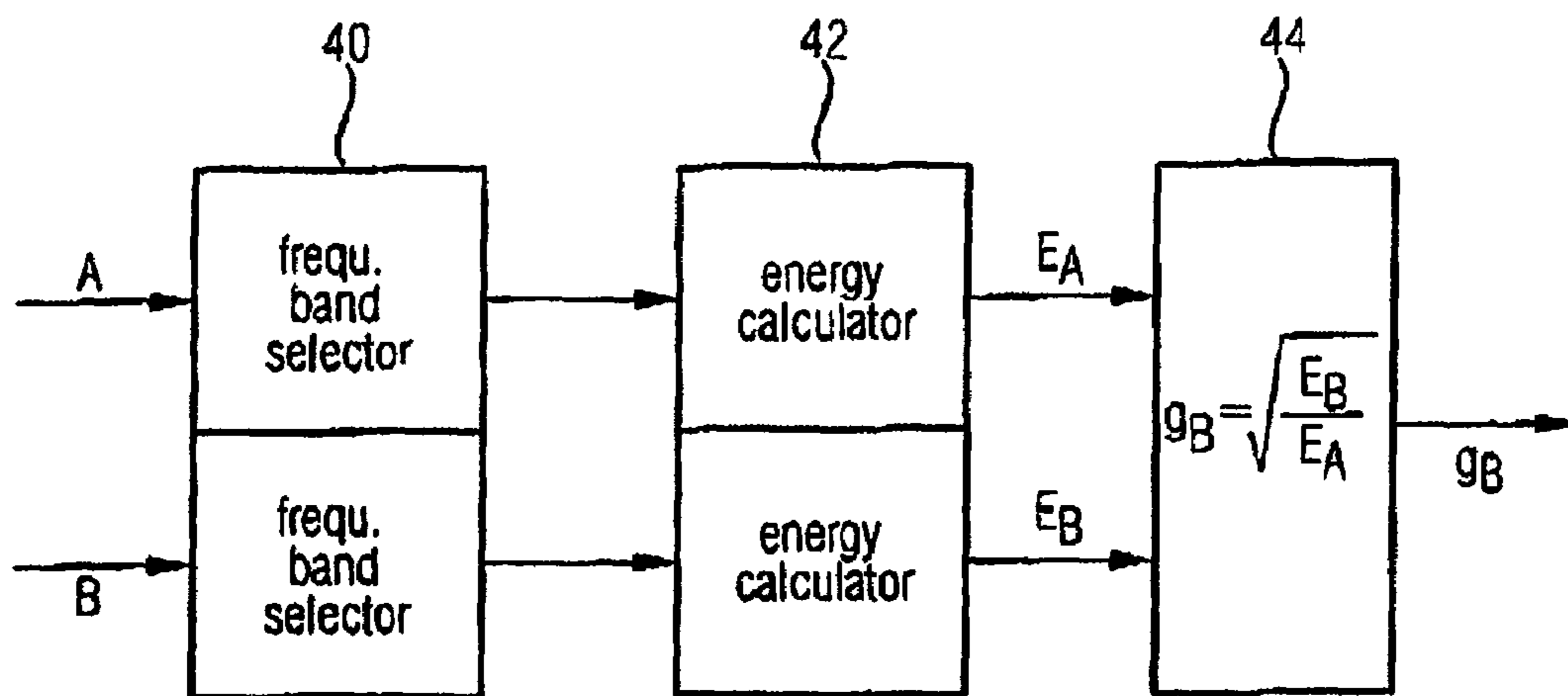
FIG 4 (encoder side)
