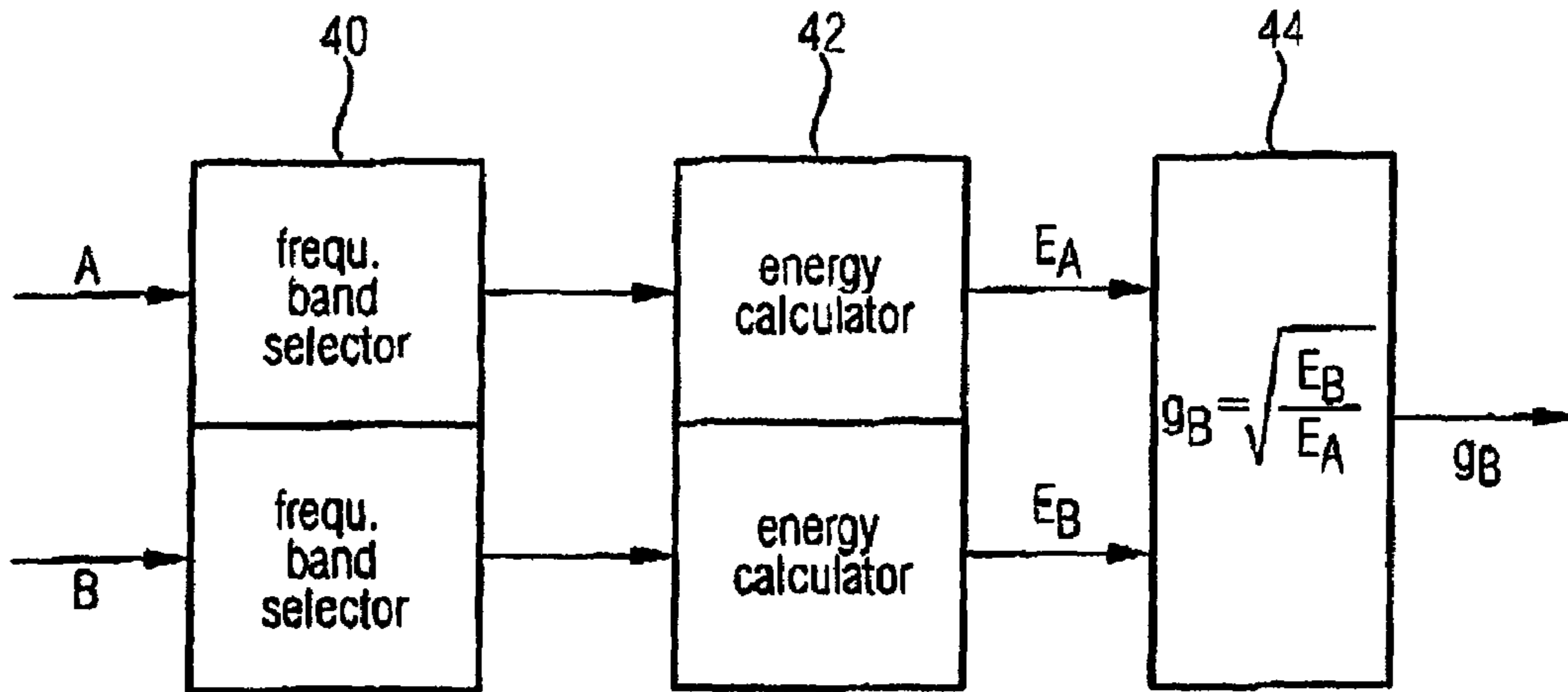
FIG 4 (encoder side)
