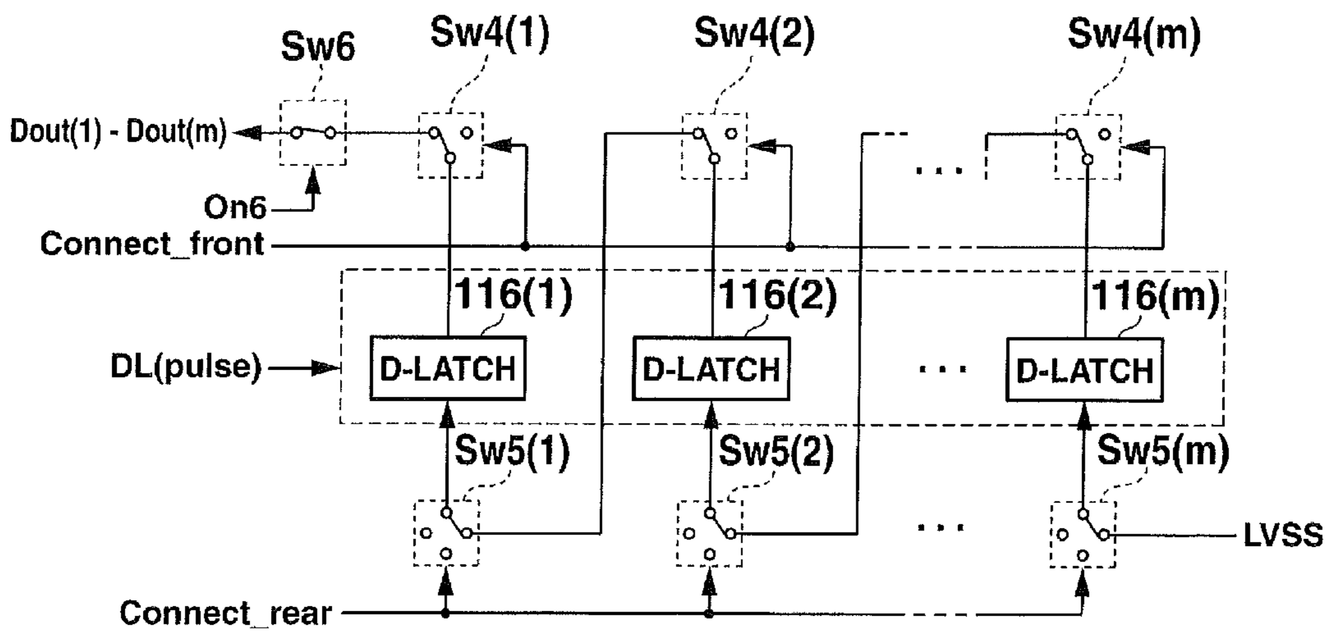
FIG.12B
