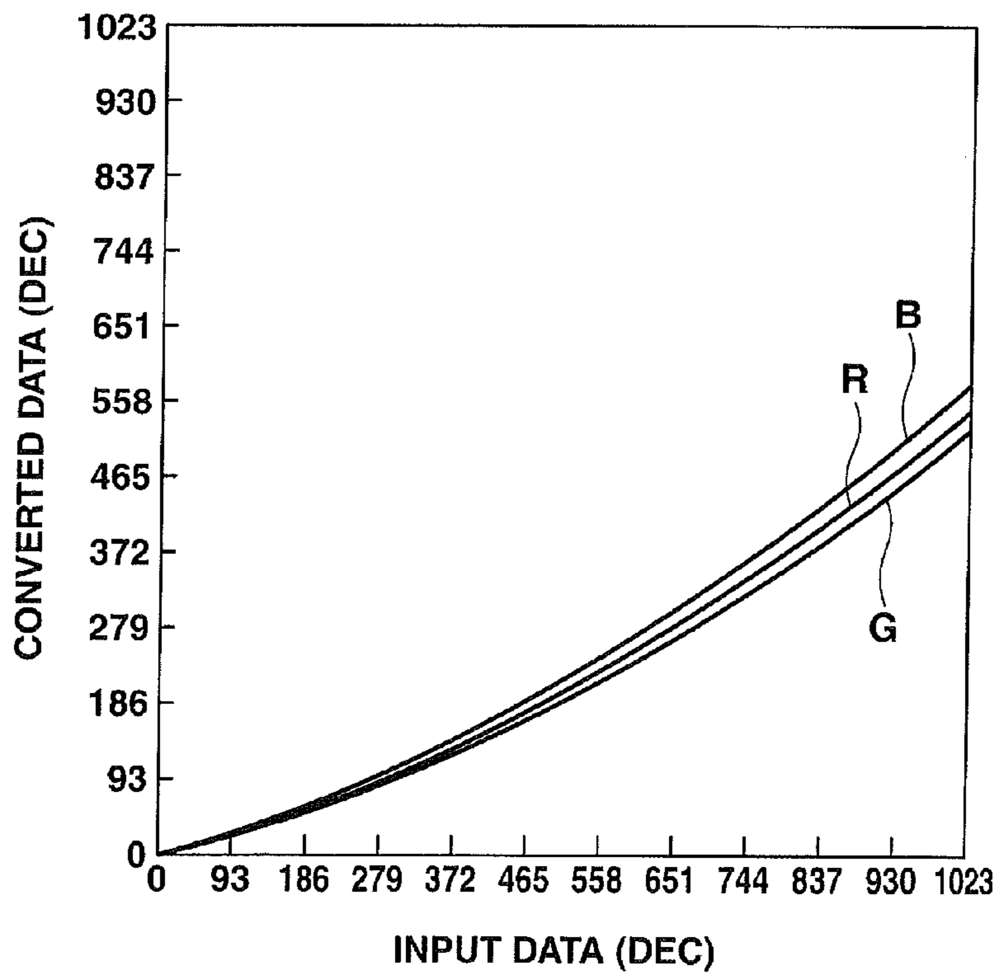
FIG.9B
