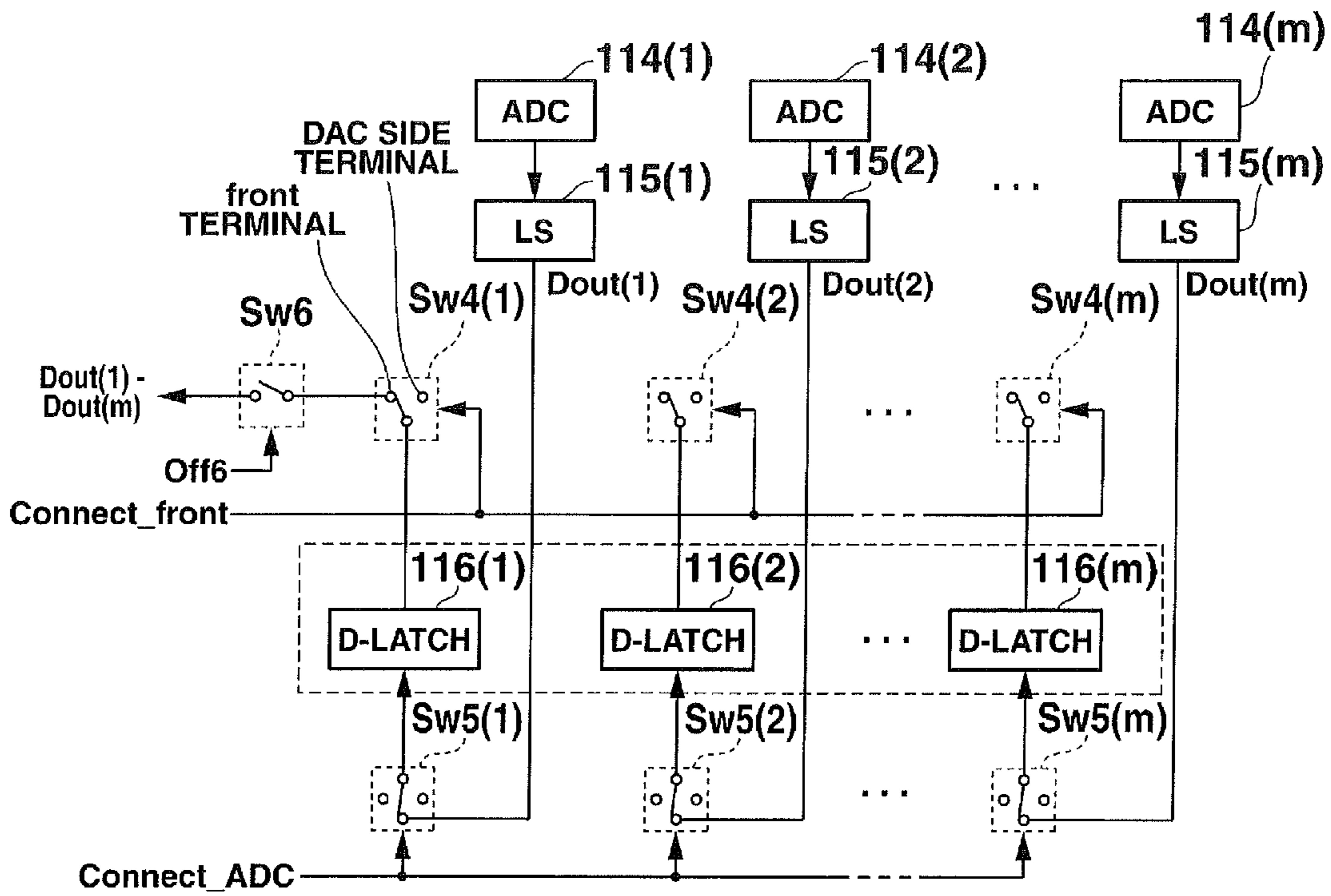
FIG.12A
