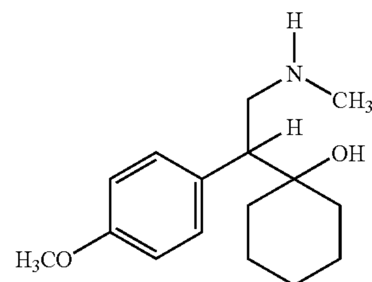
N-desmethylvenlafaxine
