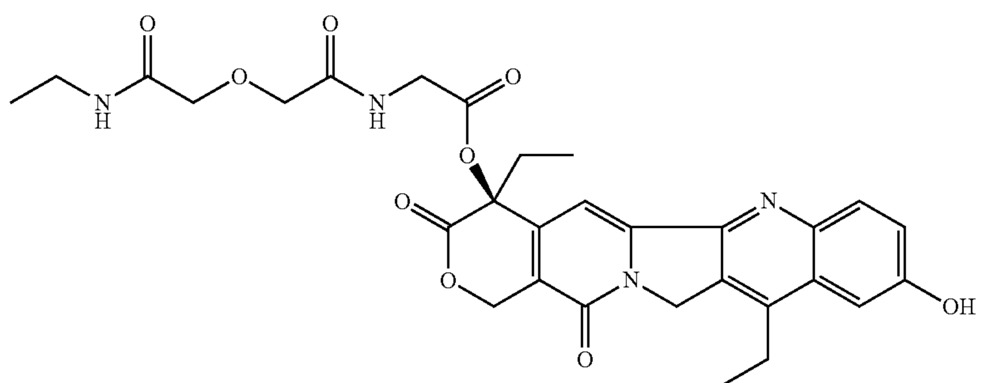
MAb-CL1-SN-38
