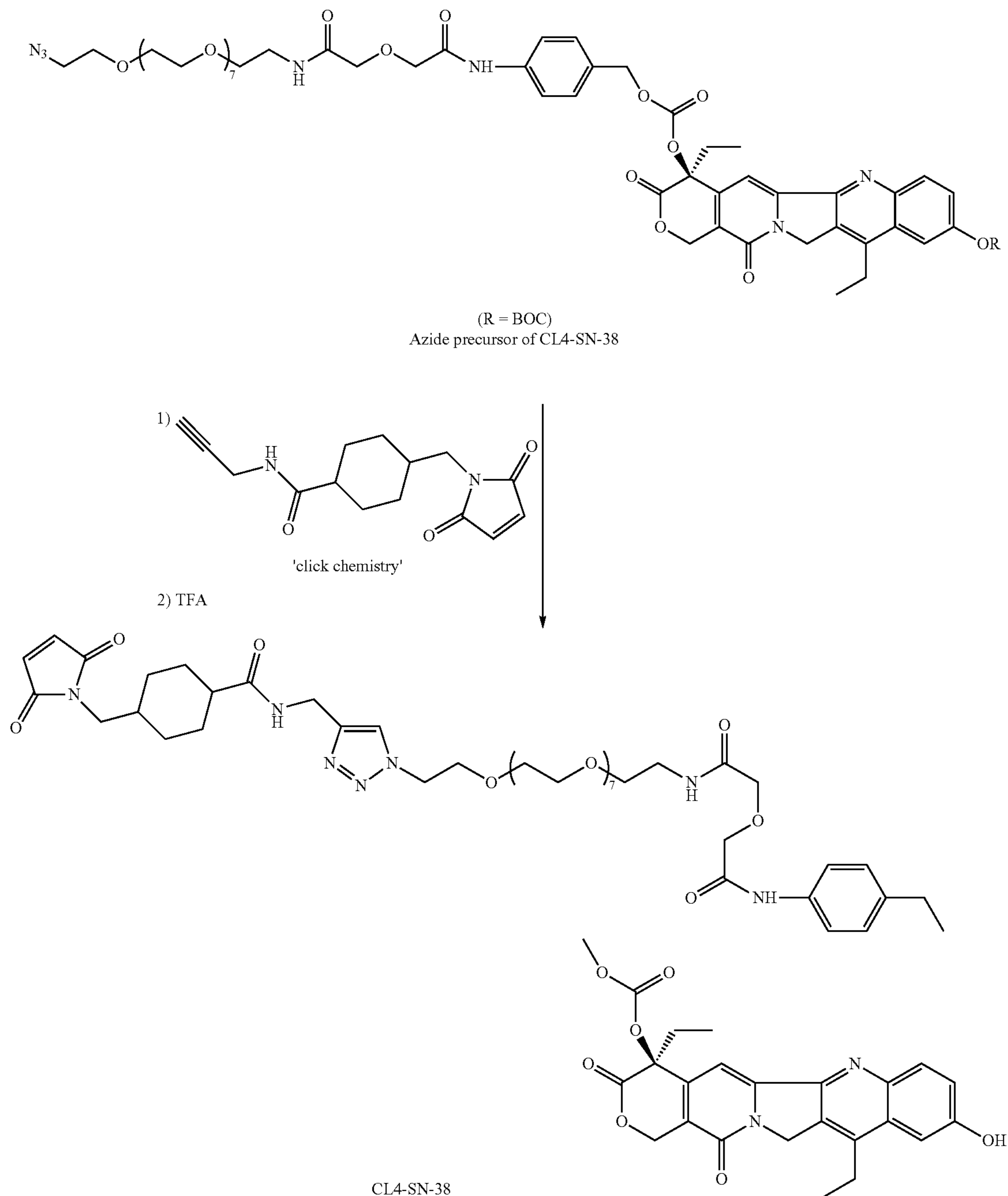
Scheme-4
