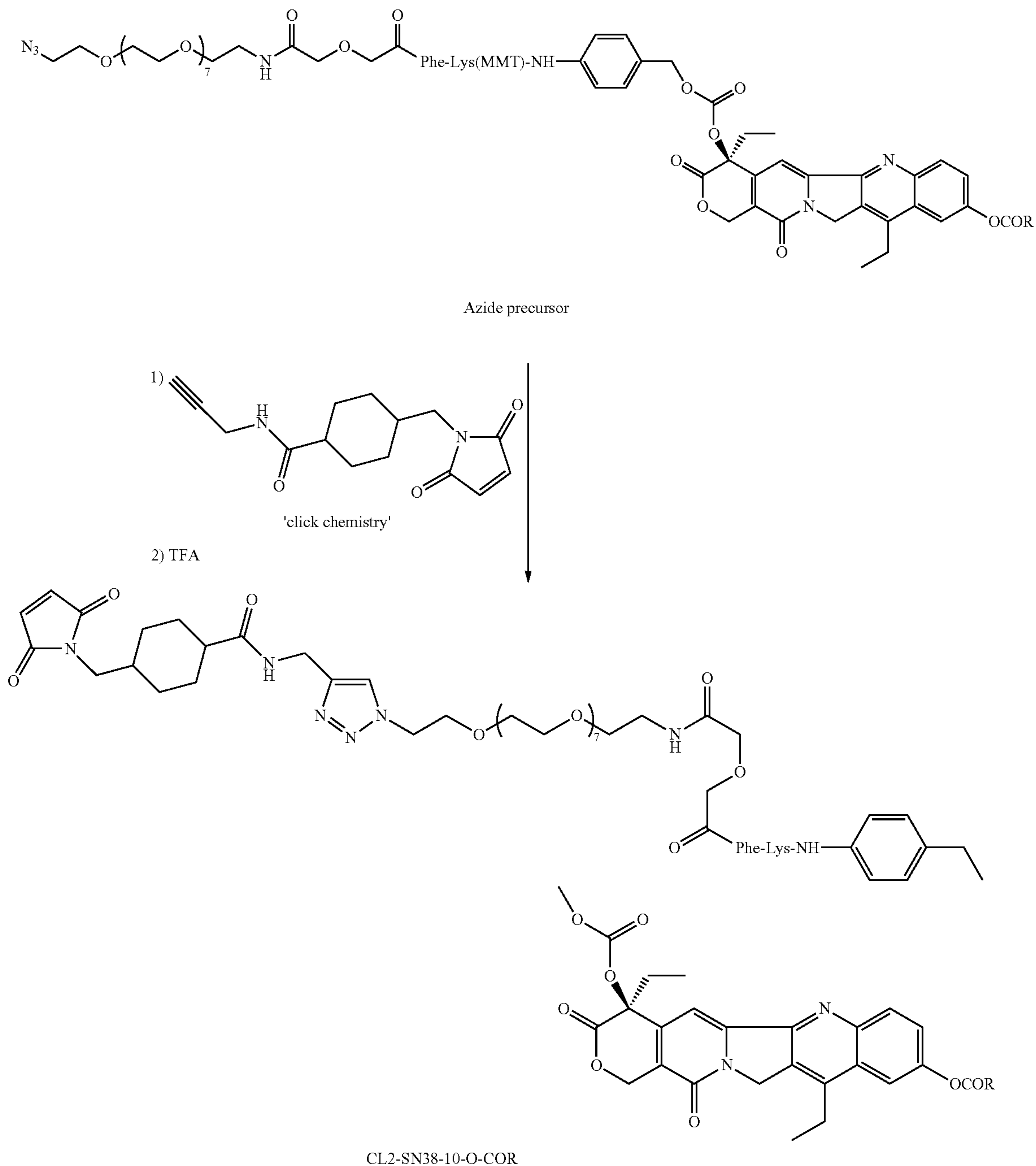
Scheme-6
