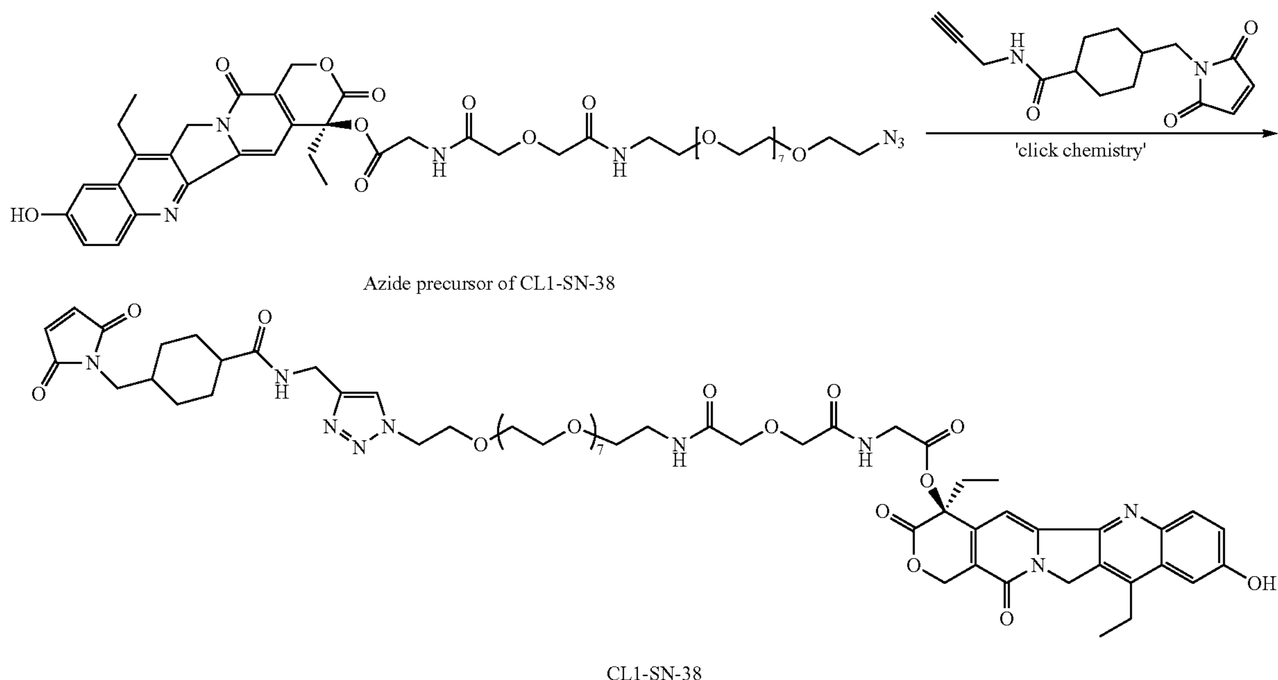
Scheme-1
