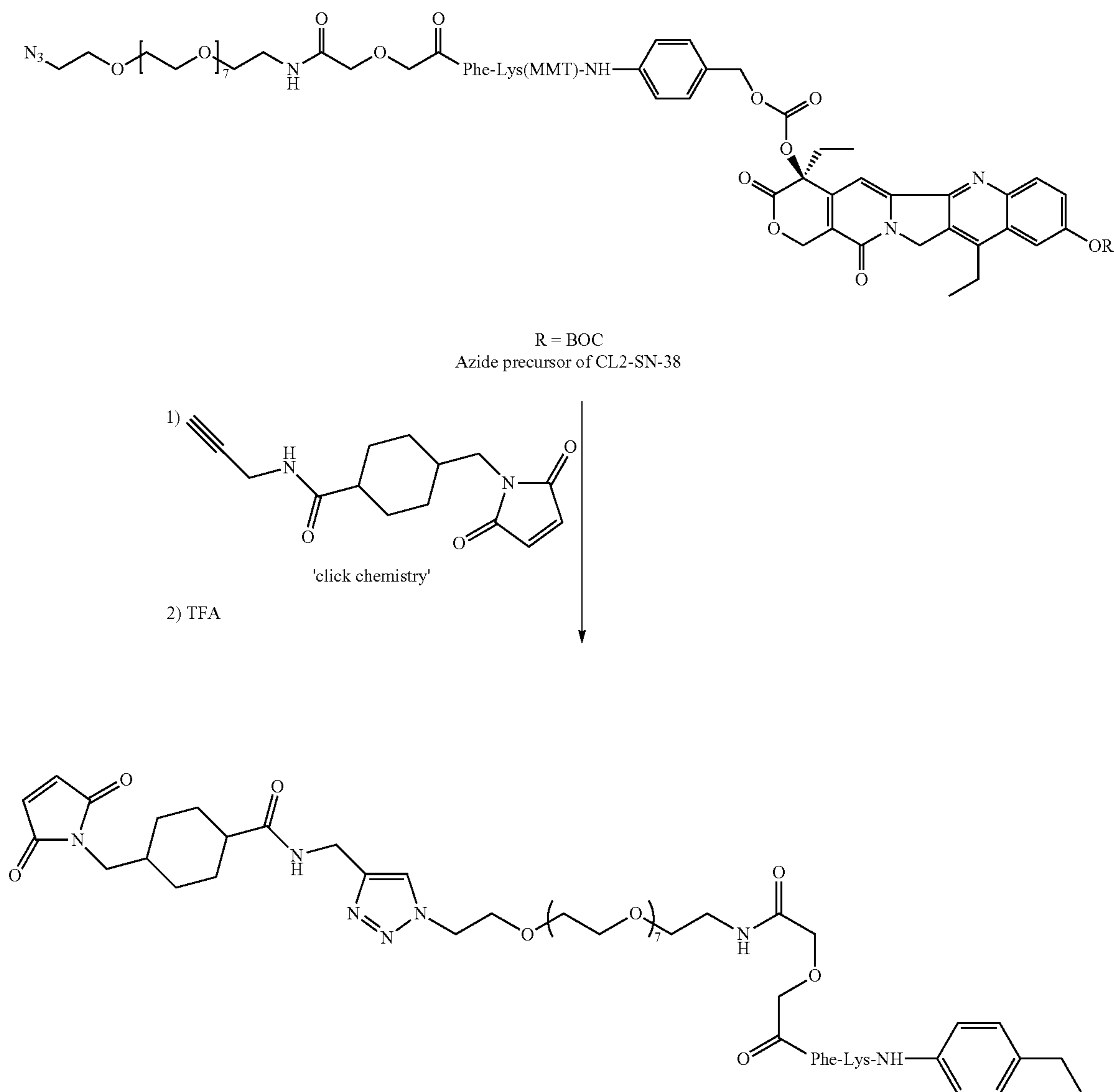
Scheme-2
