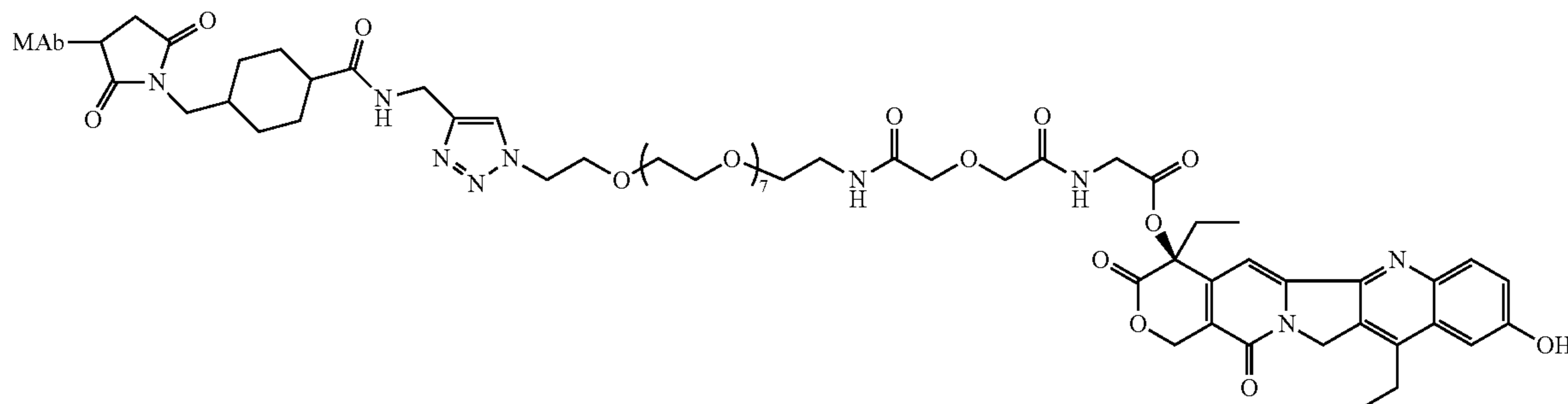
MAb-CL1-SN-38
