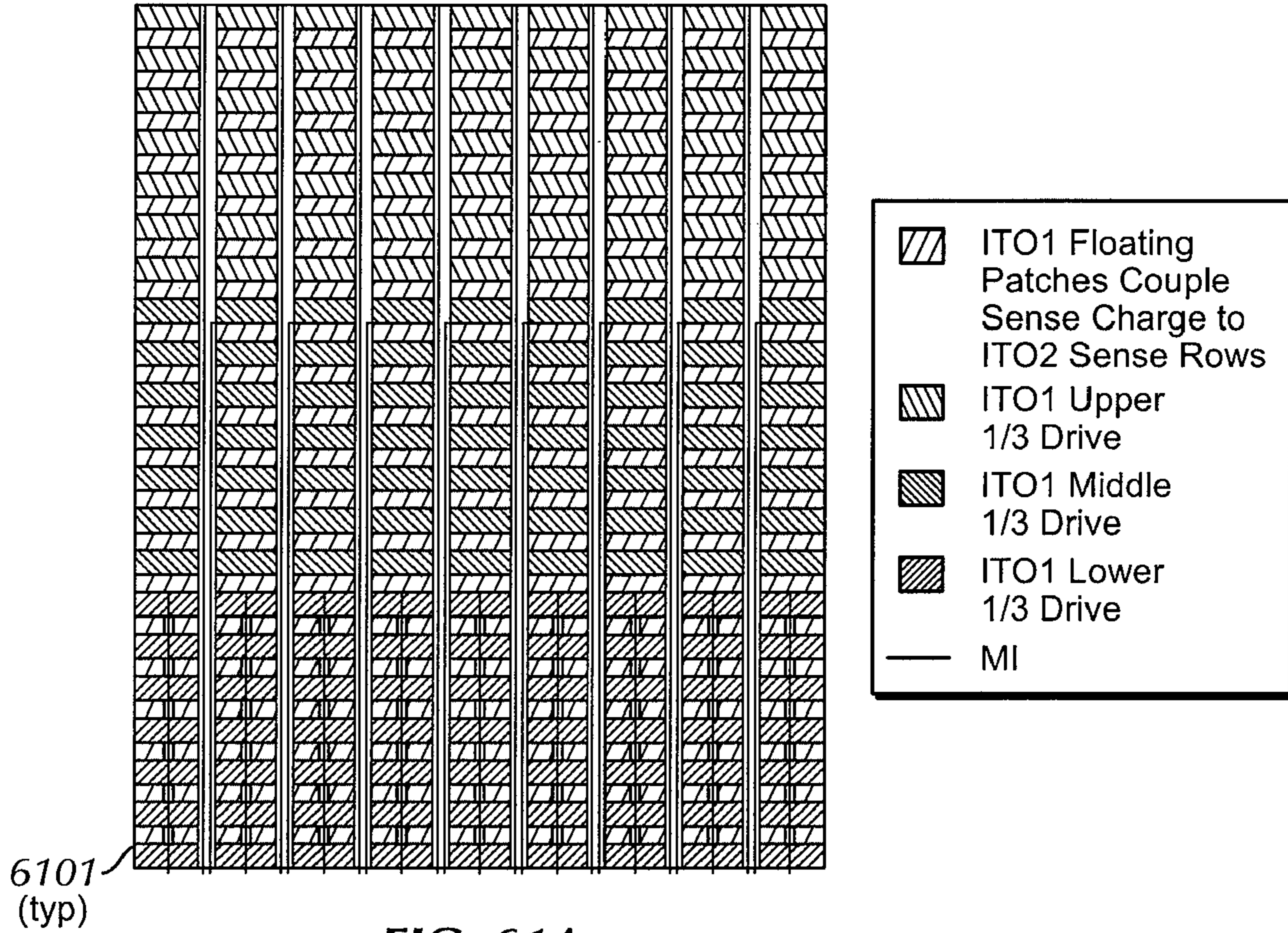
ITO1 & M1 Layout
