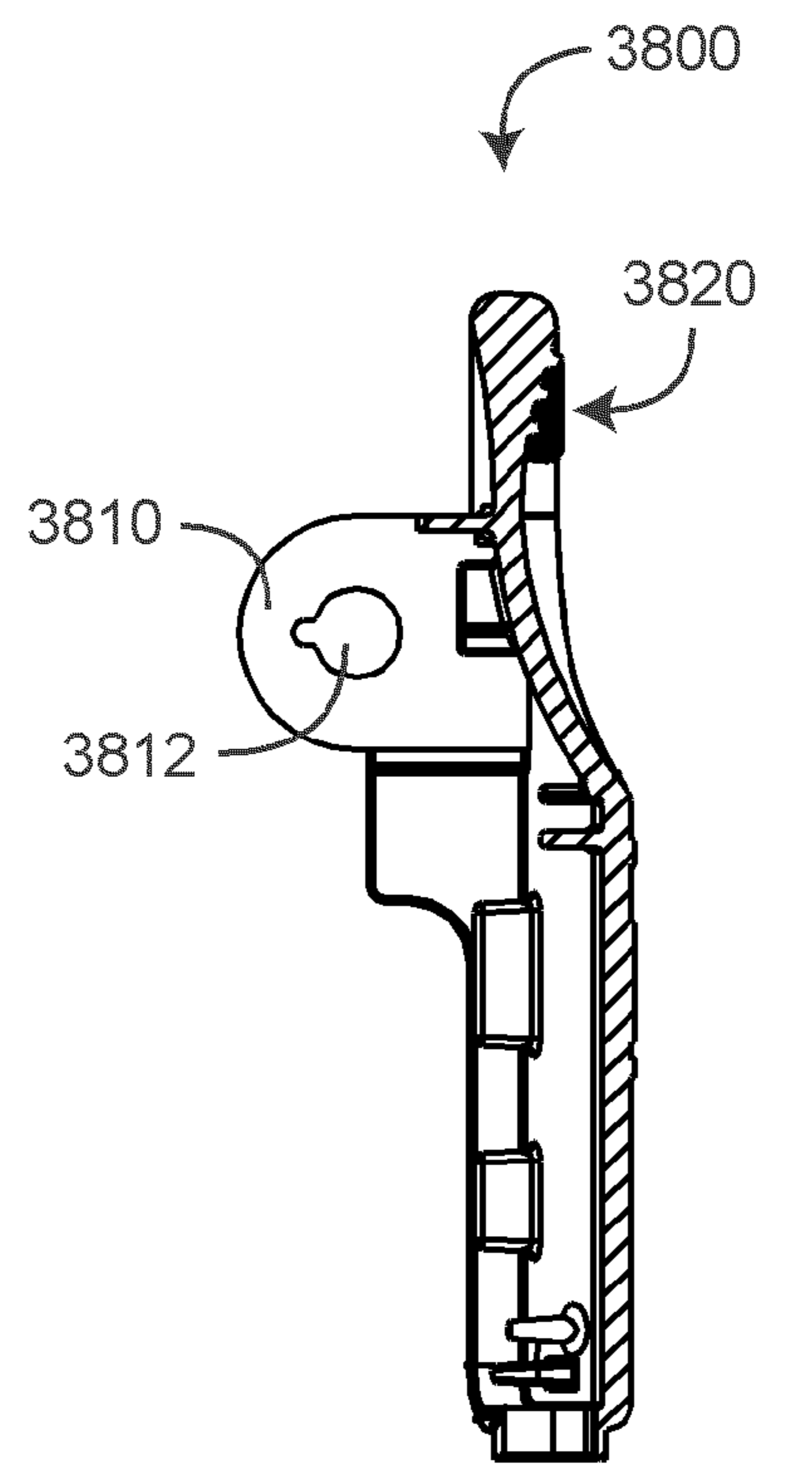
SECTION A-A FIG. 38D
