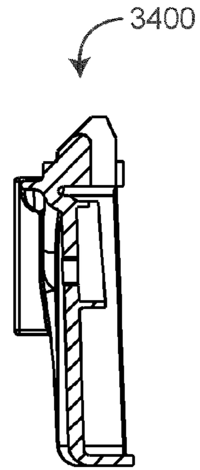
SECTION A-A
