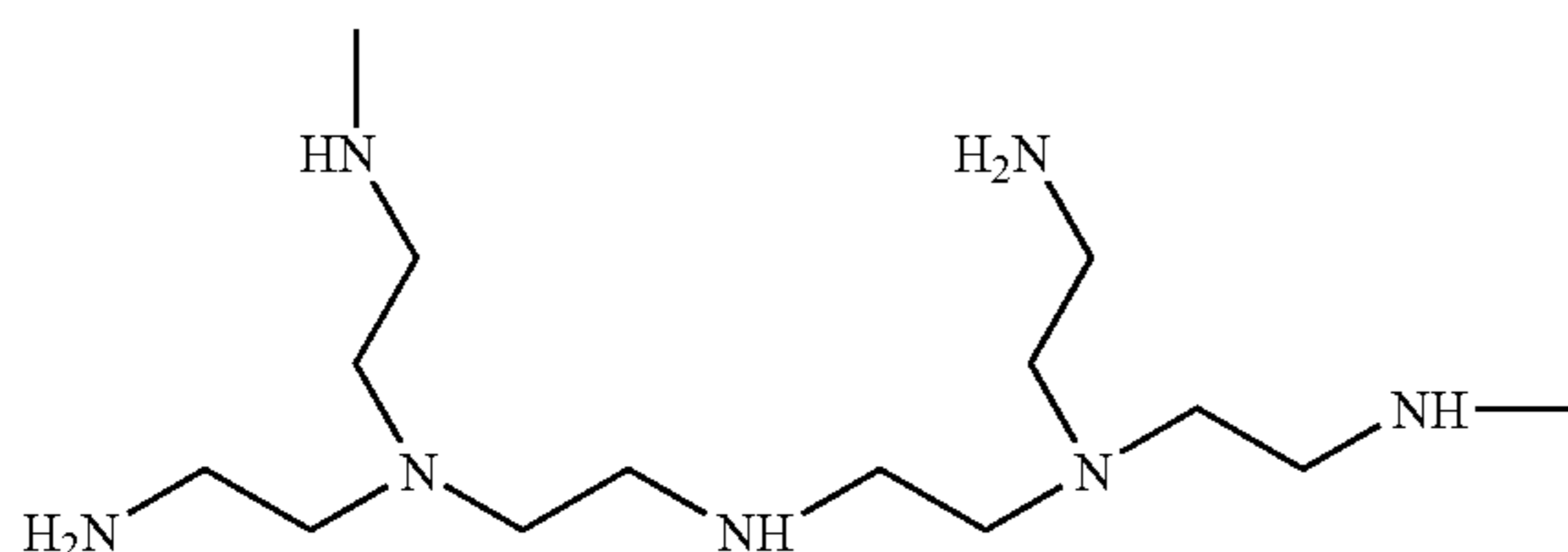
Polyethyleneimine
