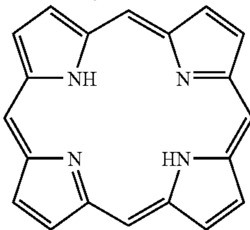
Porphyrin
