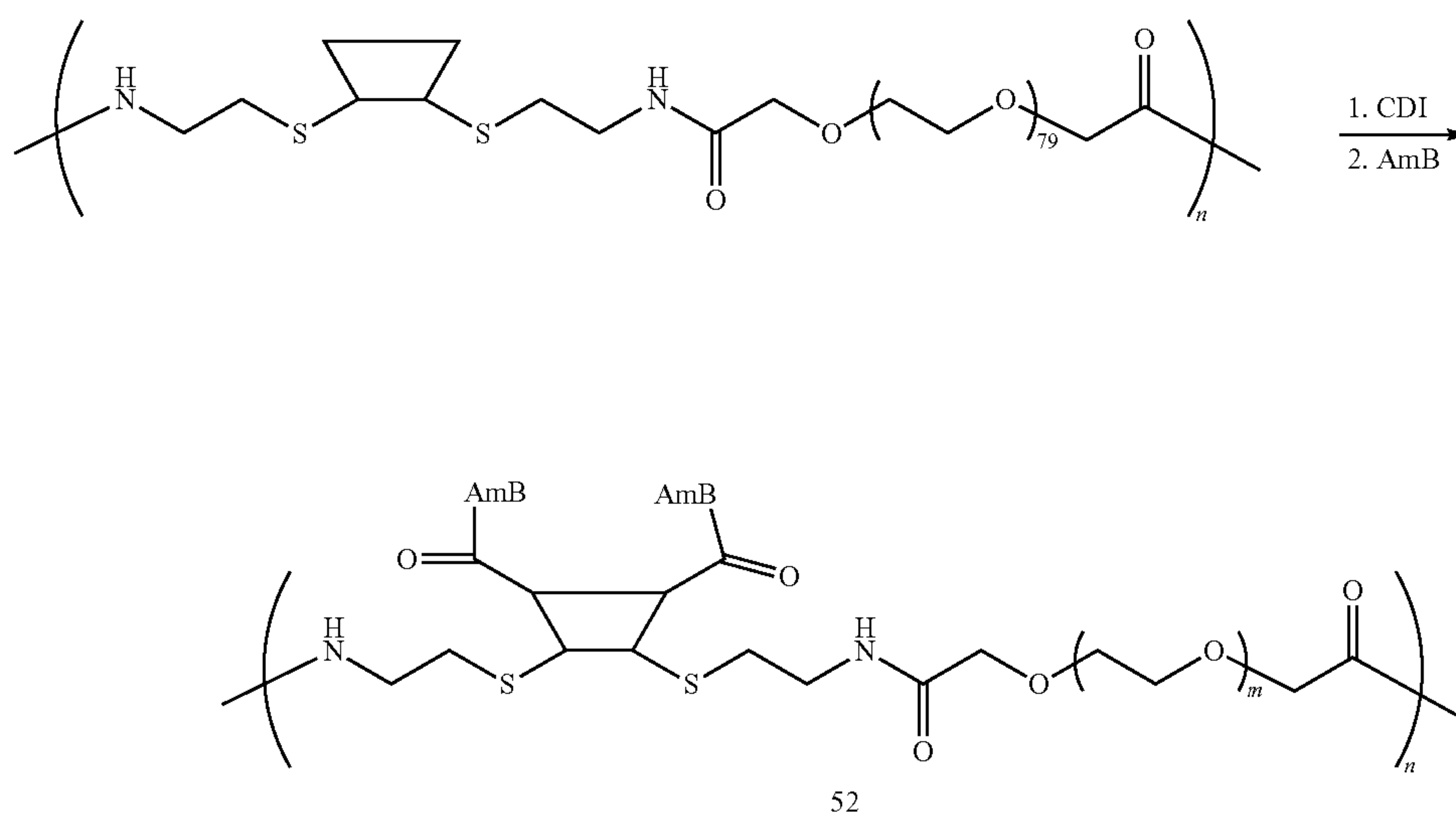
Scheme LII
