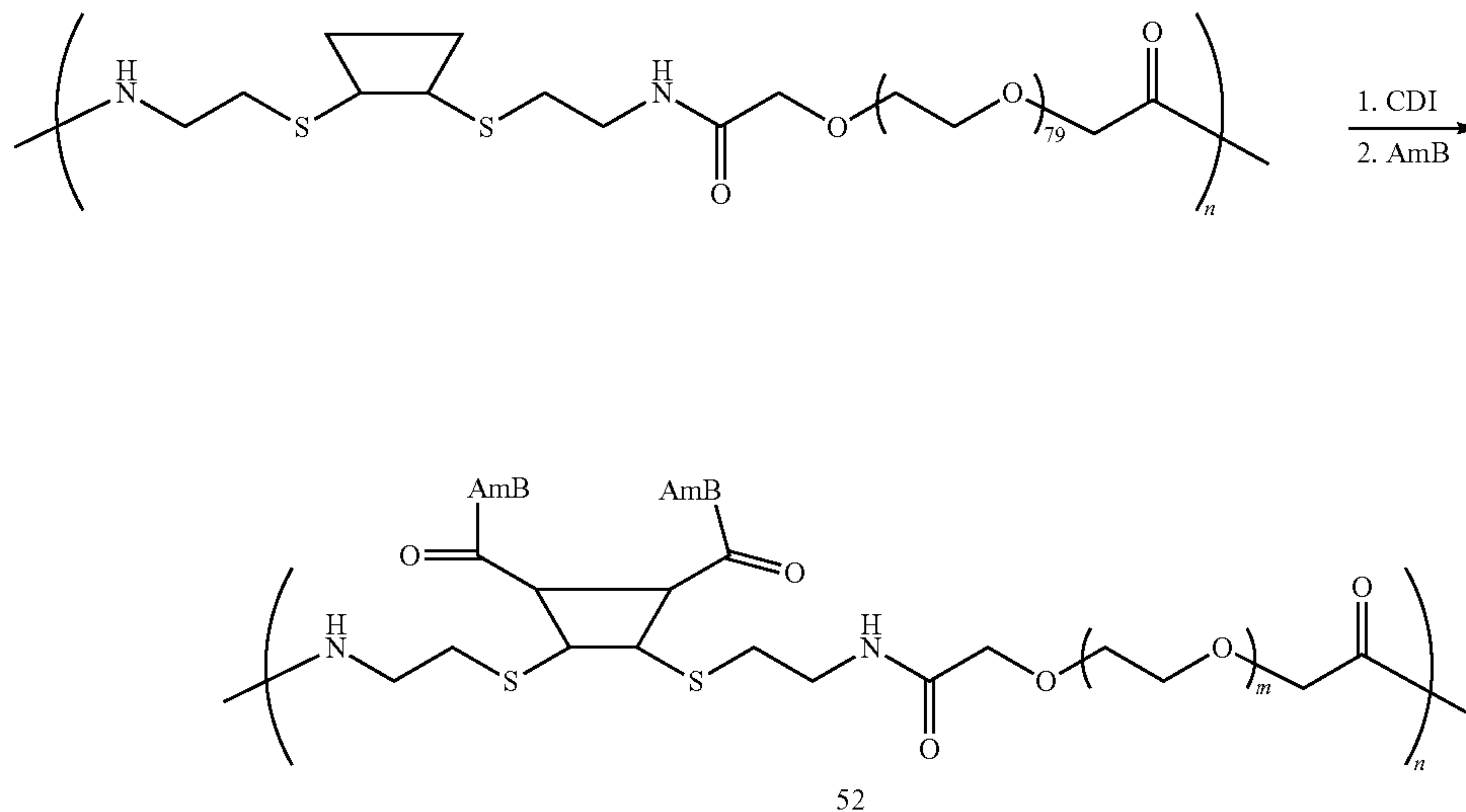
Scheme LII
