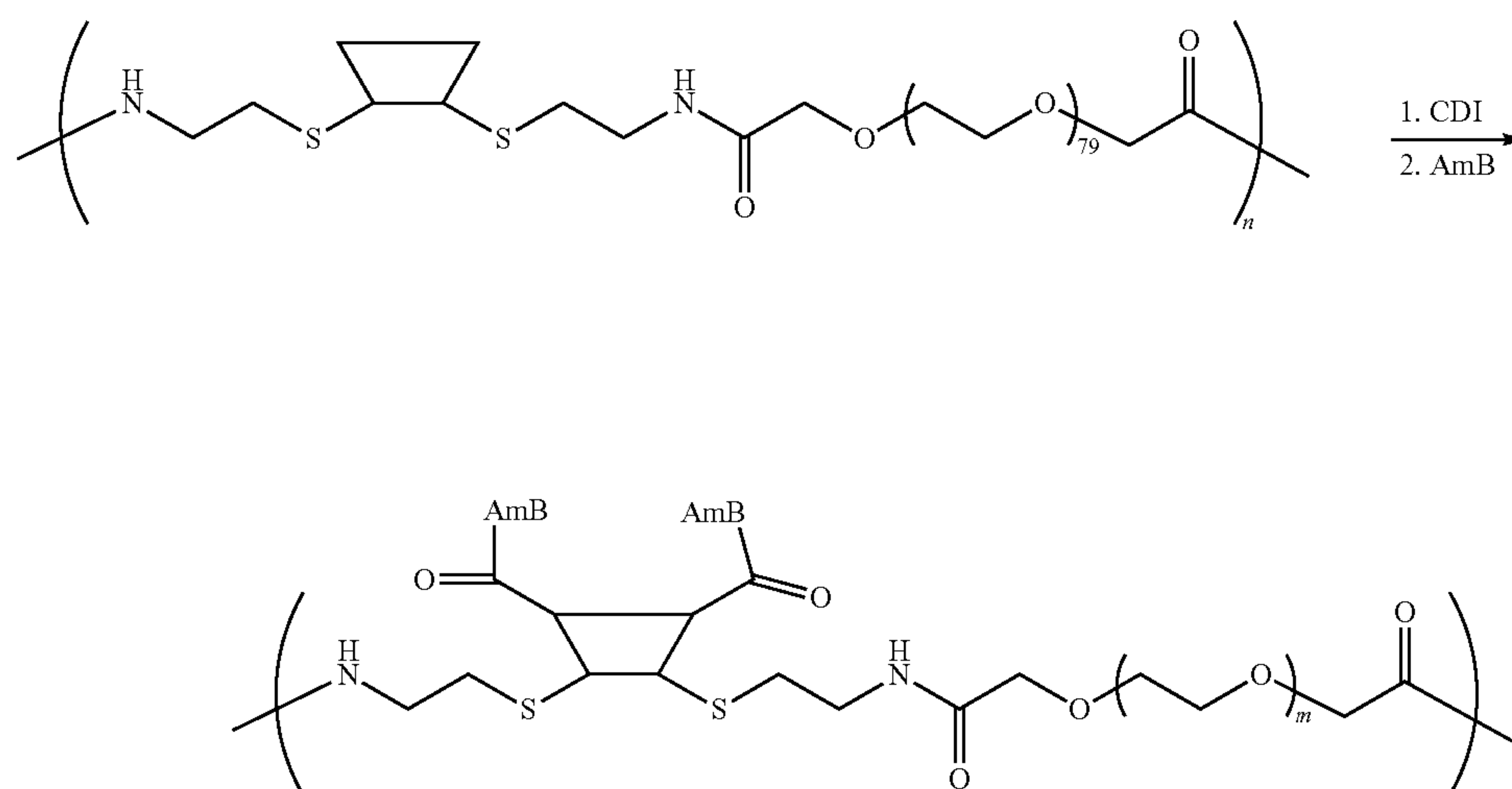
Scheme LII
