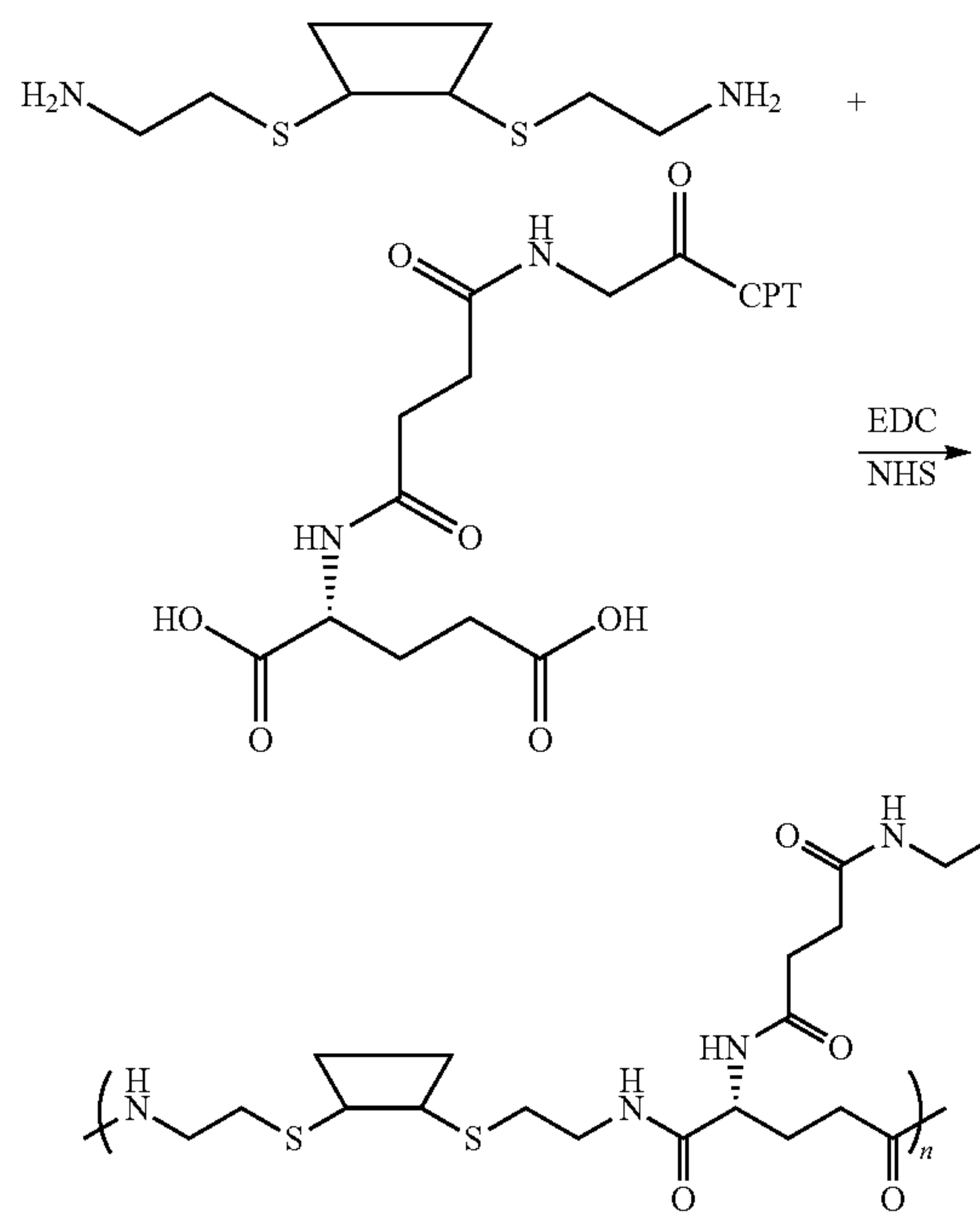
Scheme VI
