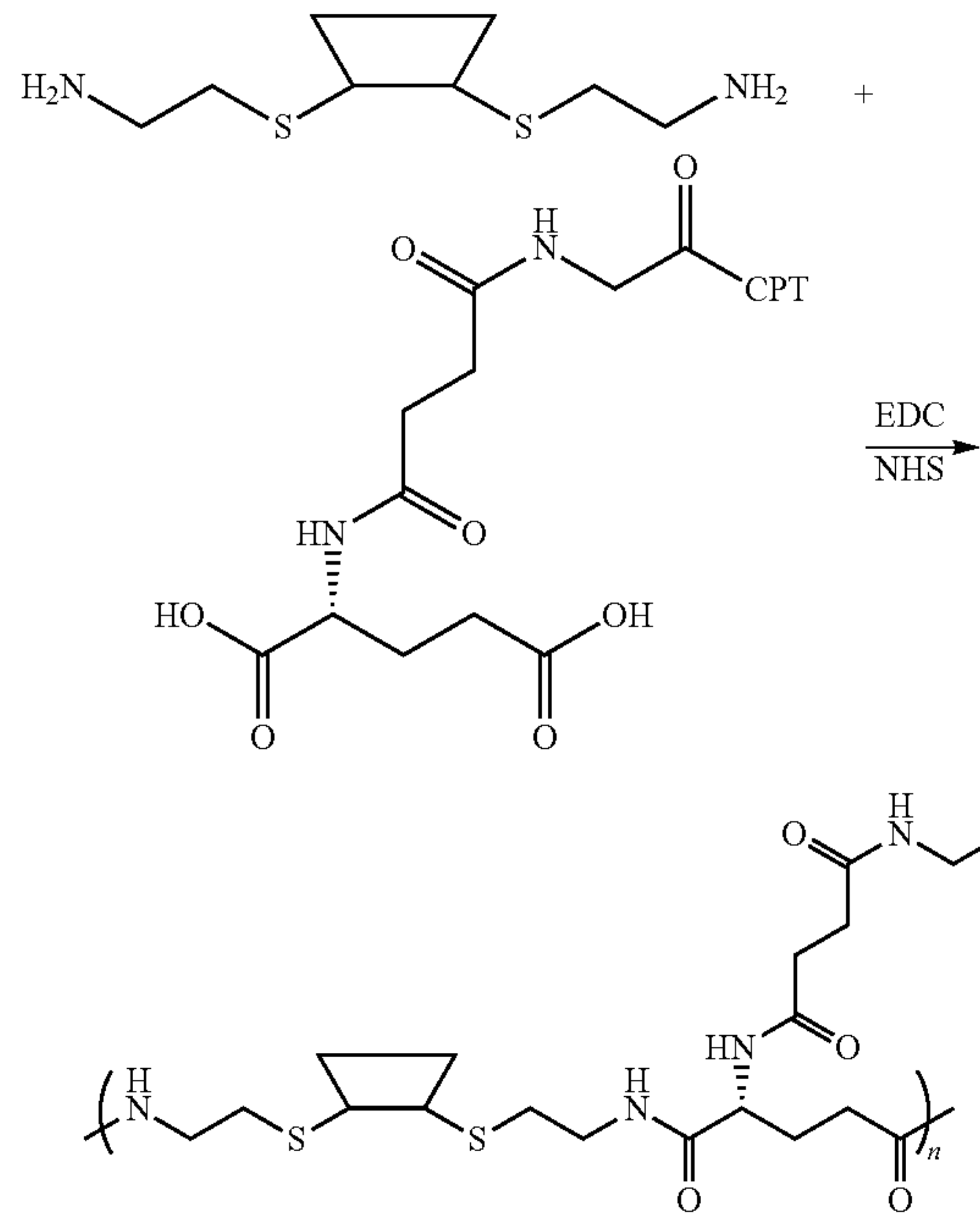
Scheme VI
