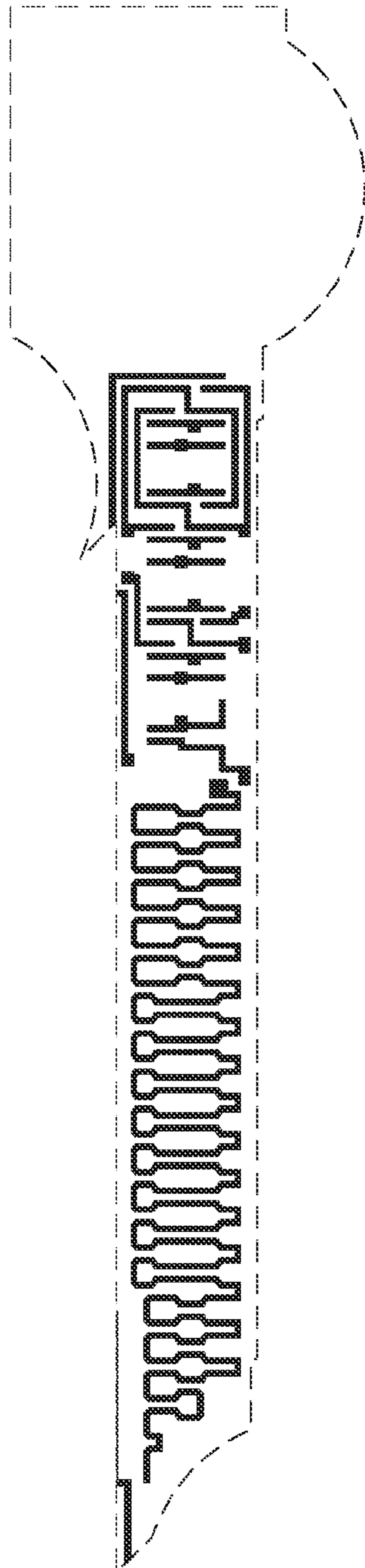
Poly mask
