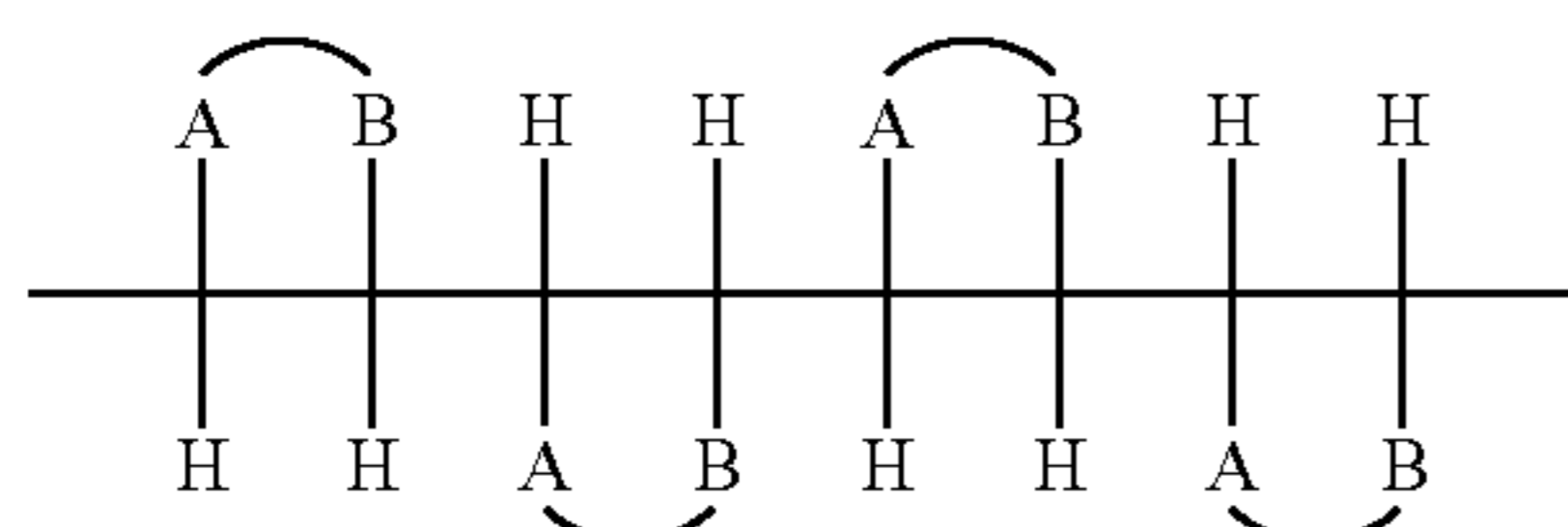
erythrodisyndiotactic homopolymer
