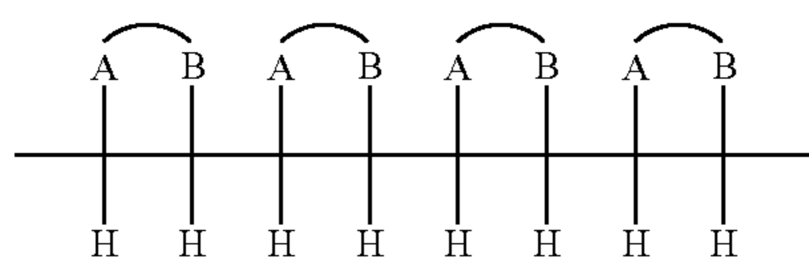
erythrodiisotactic homopolymer
