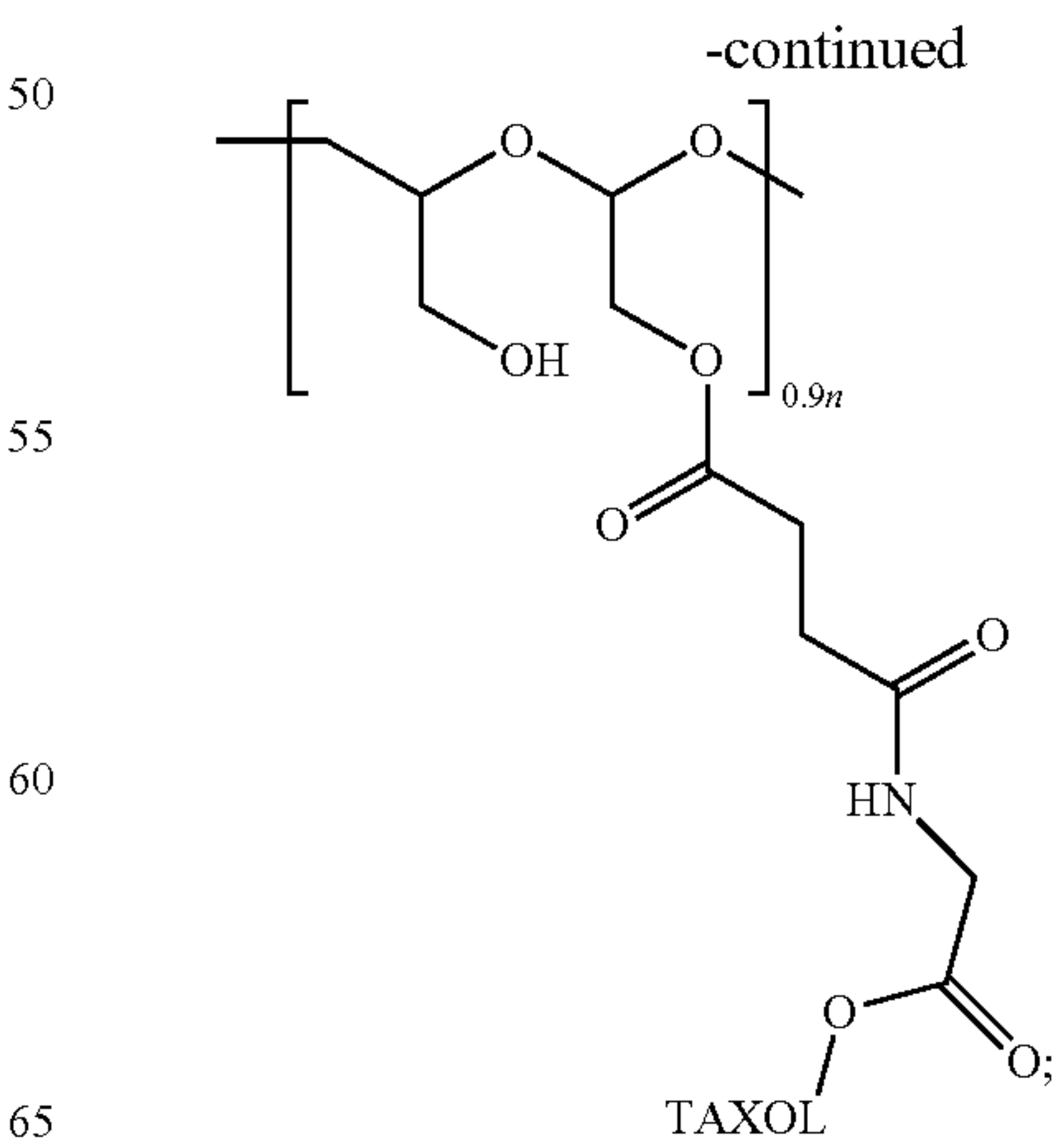
(IIa)
