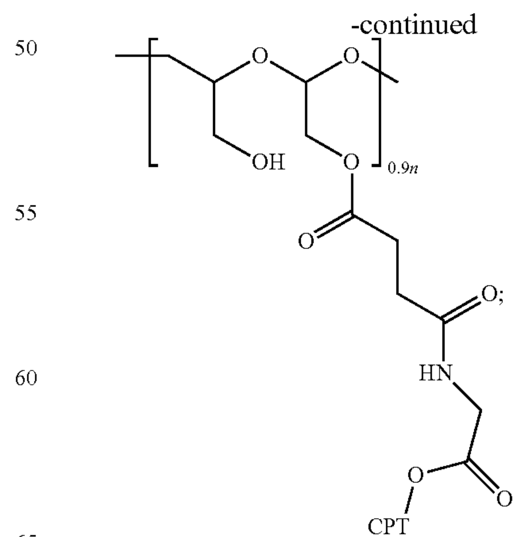
(Ia)
