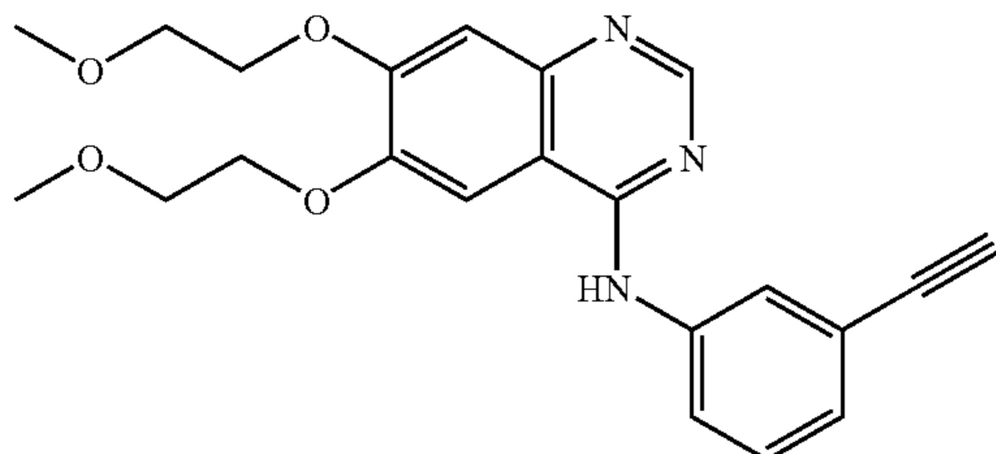
N-(3-ethynylphenyl)-6,7-bis(2-methoxyethoxy)quinazolin-4-amine
