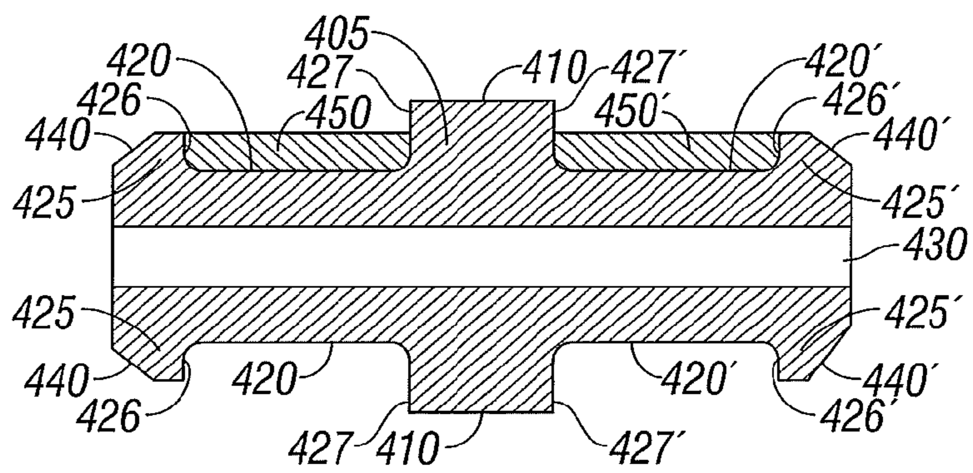
Section A-A
