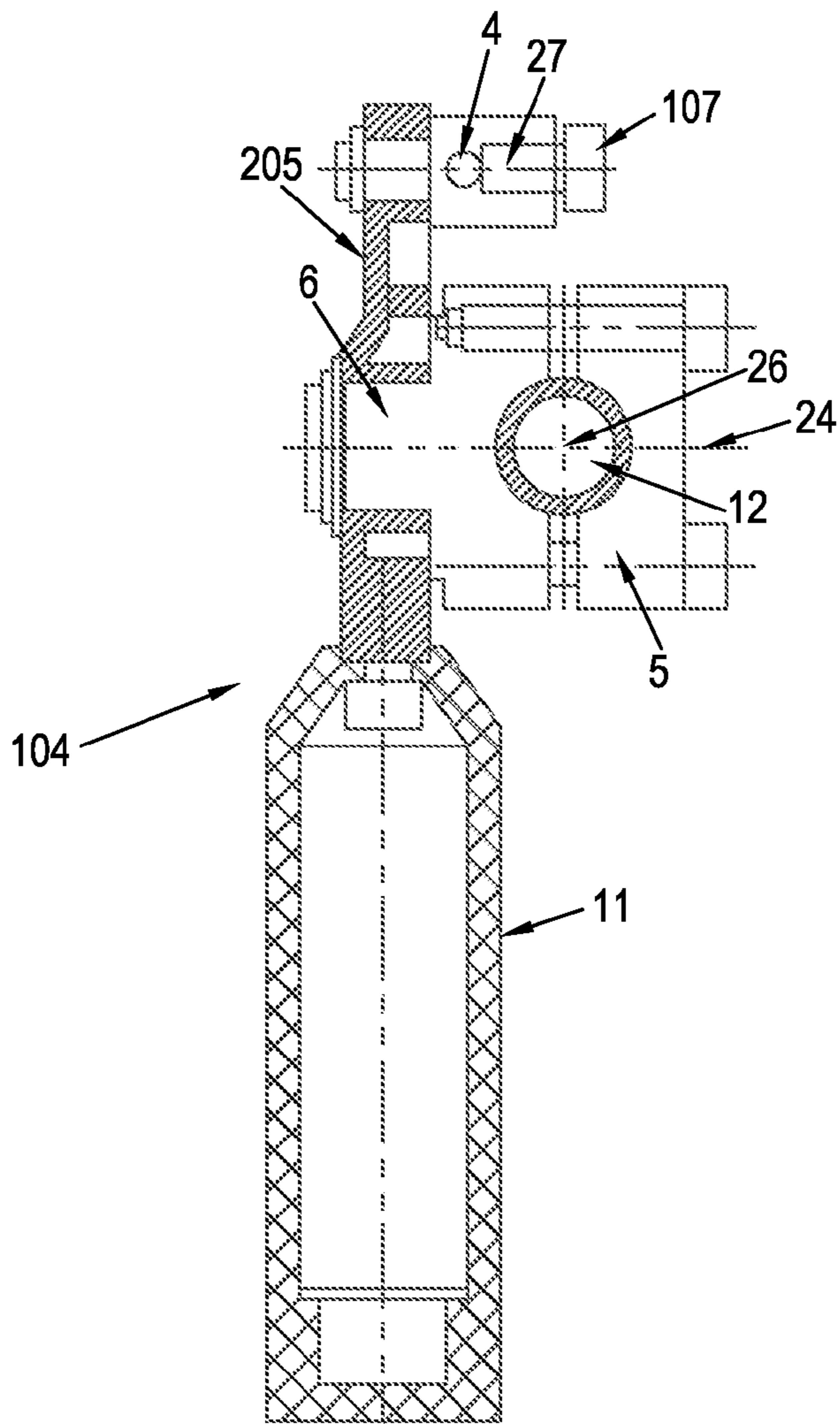
FIG. 2 SECTION A-A
