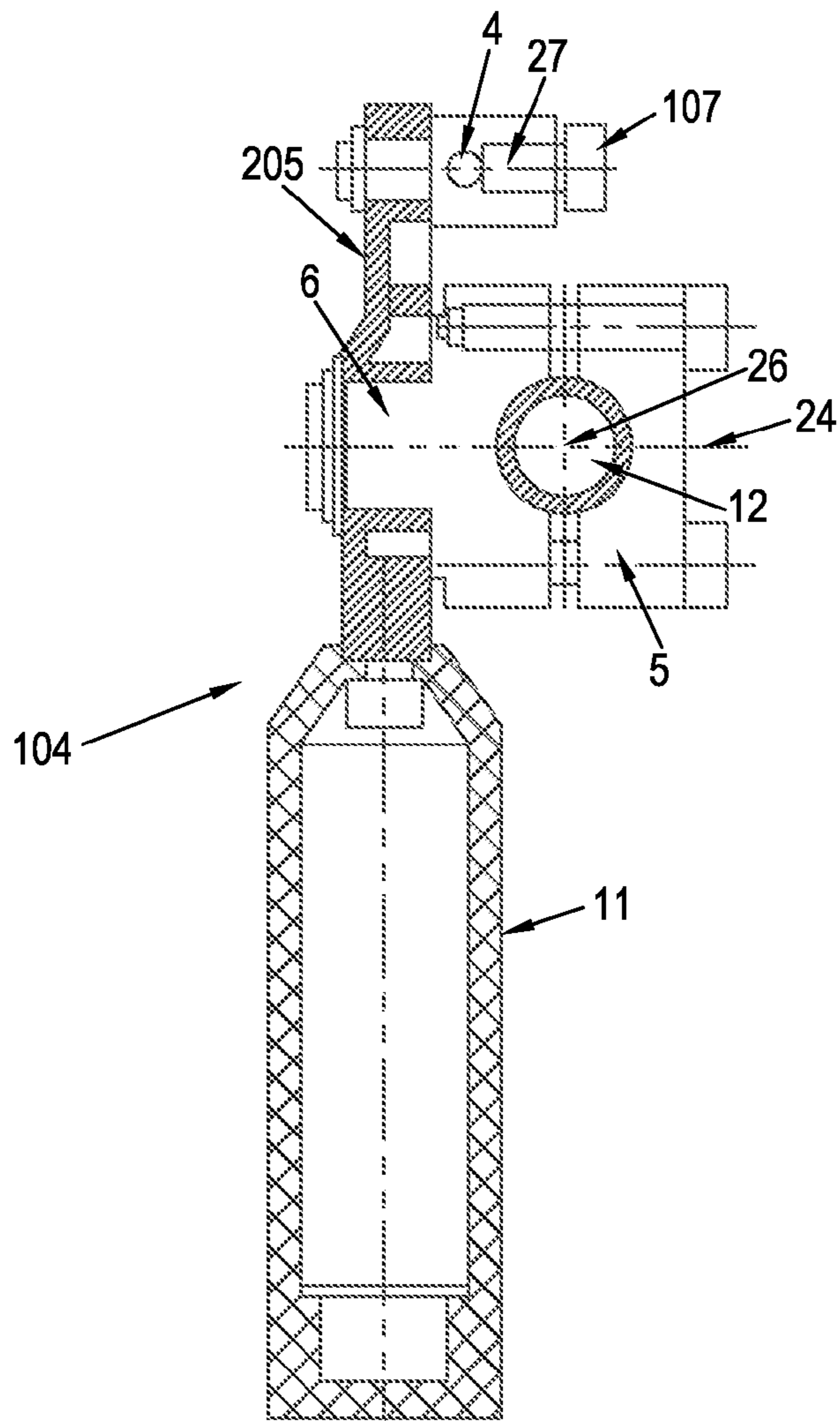
FIG. 2 SECTION A-A
