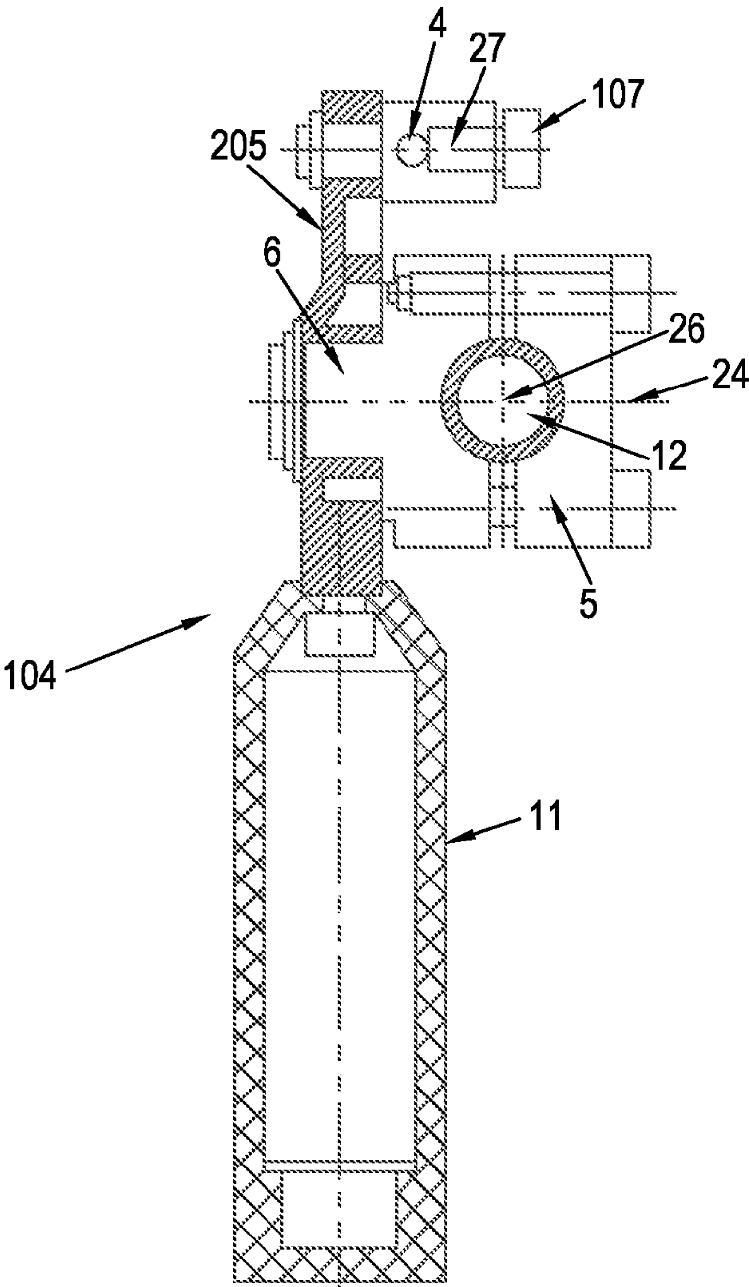
FIG. 2 SECTION A-A
