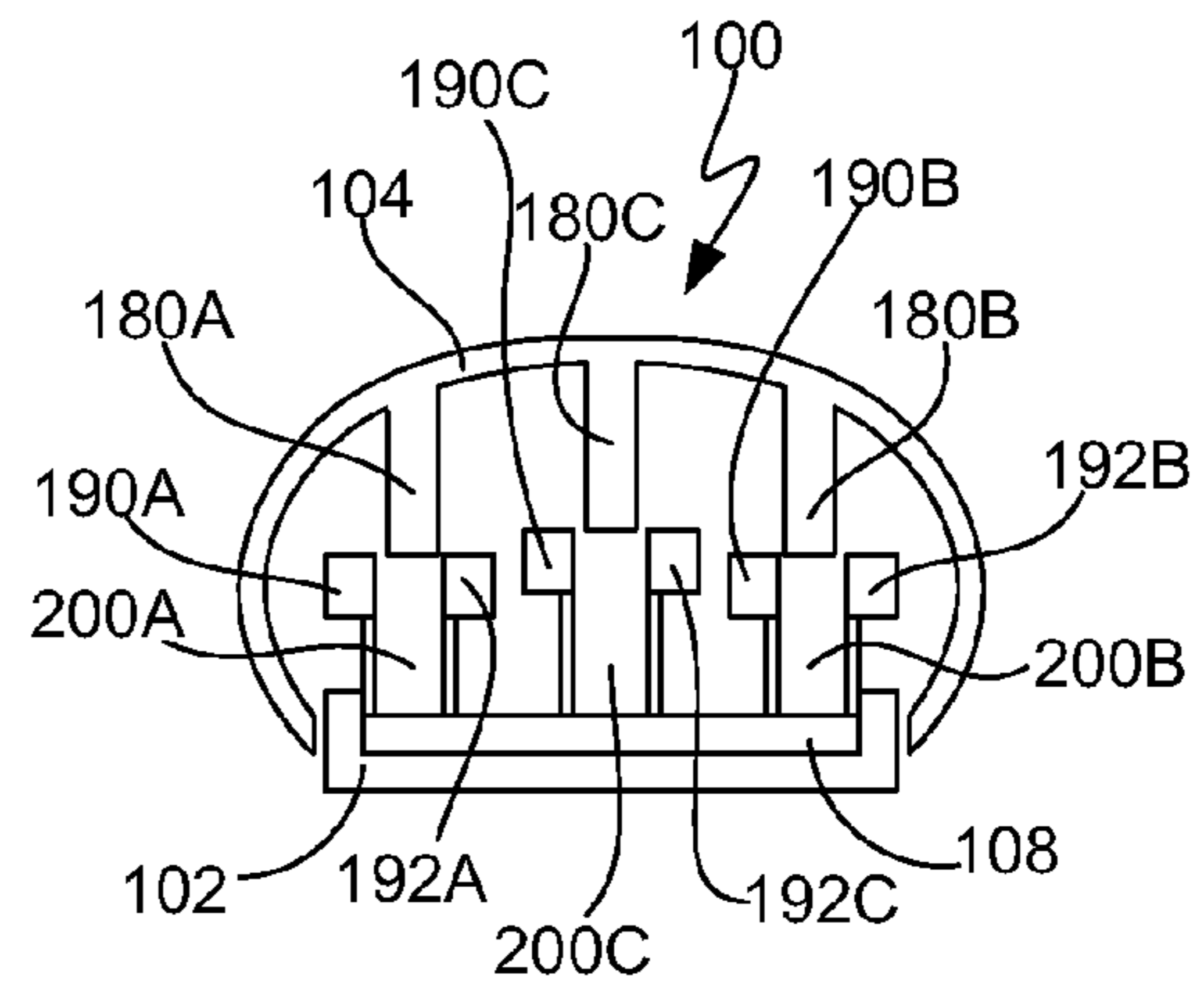
FIG. 10B
