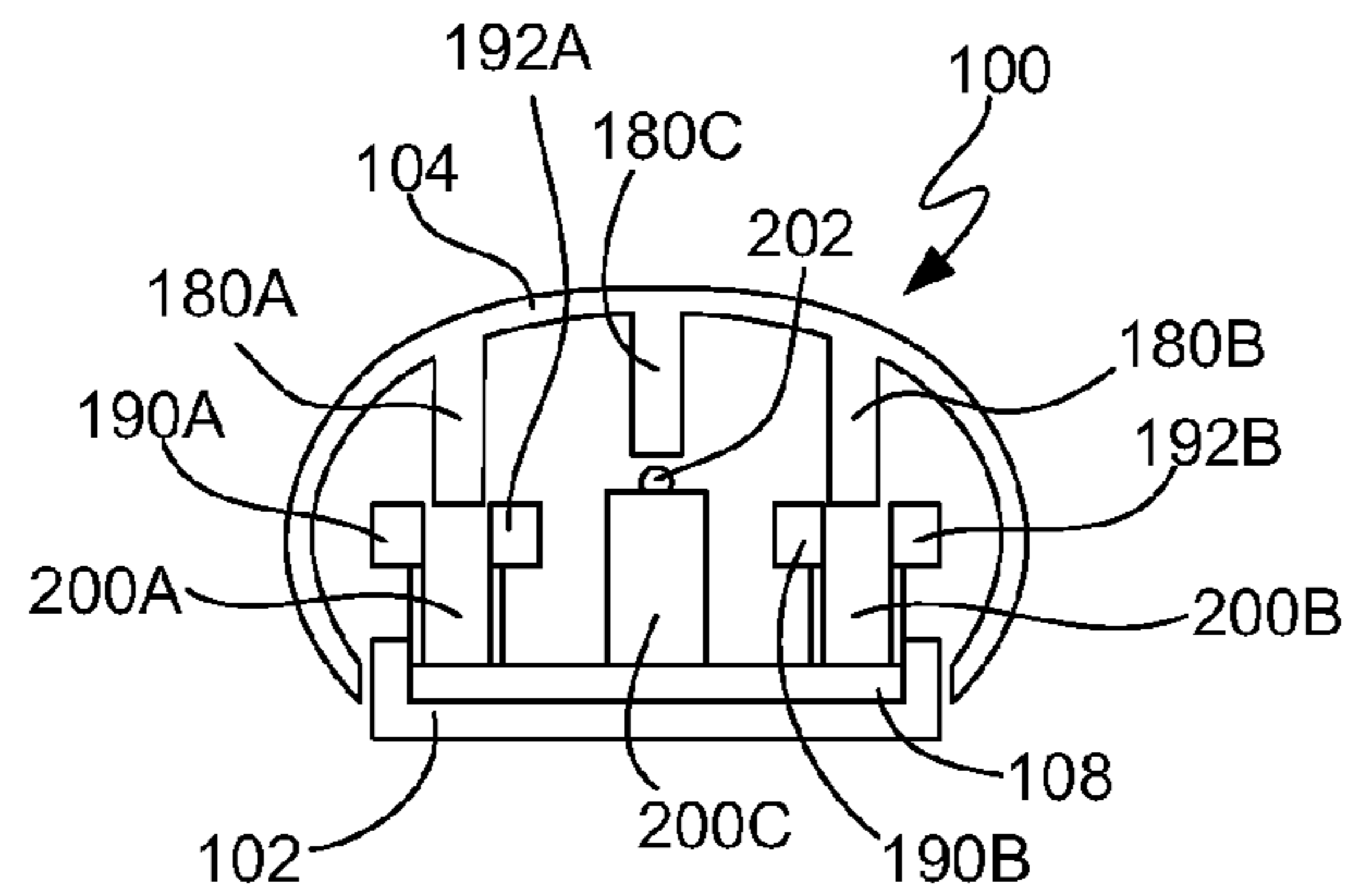
FIG. 10A
