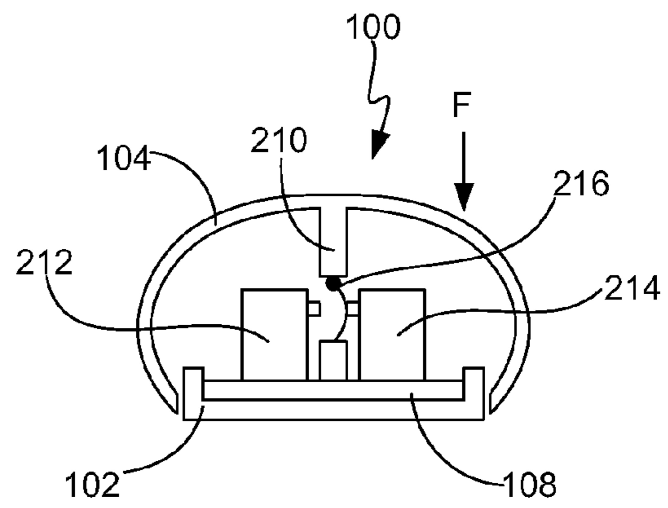
FIG. 11B
