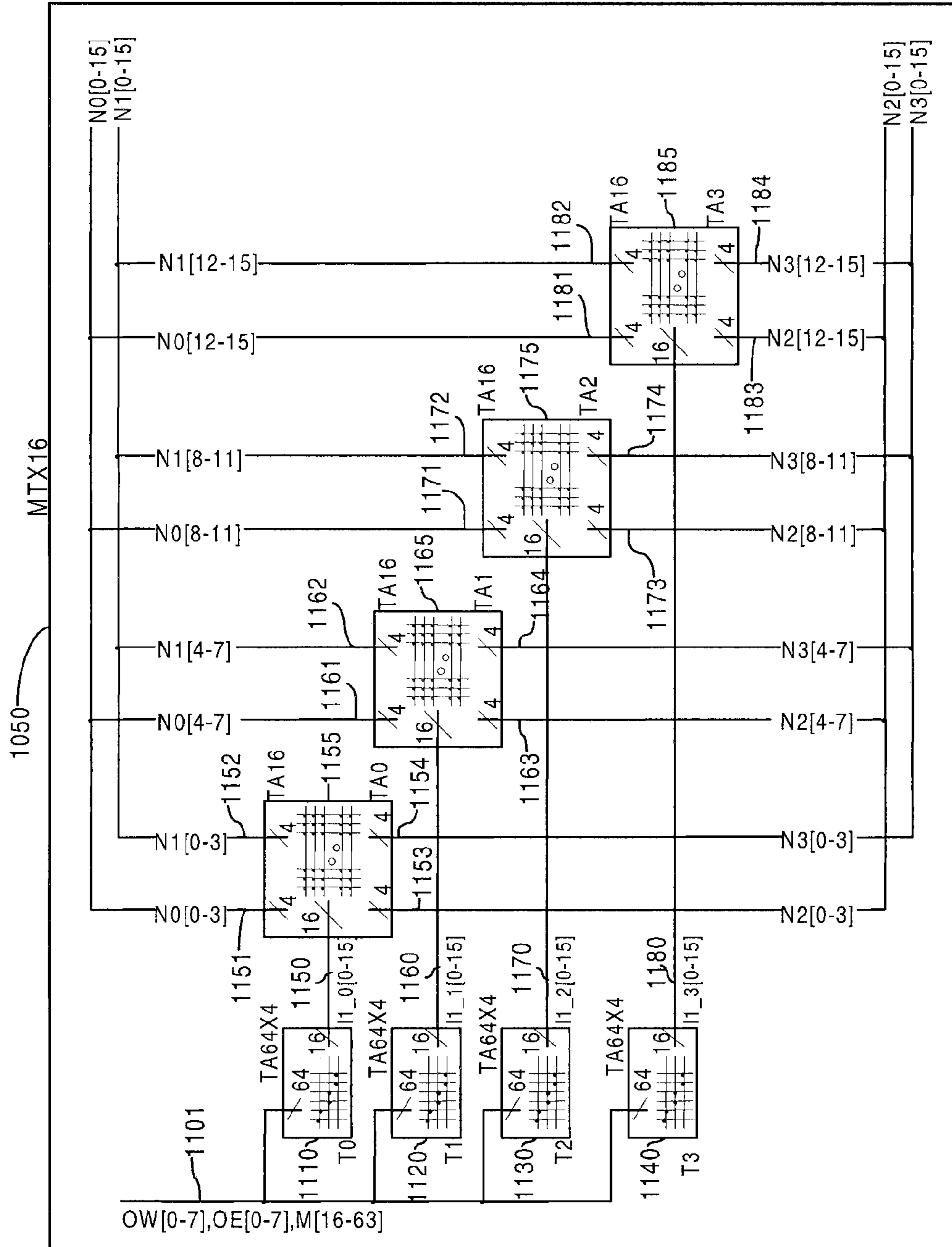
FIG. 11A
