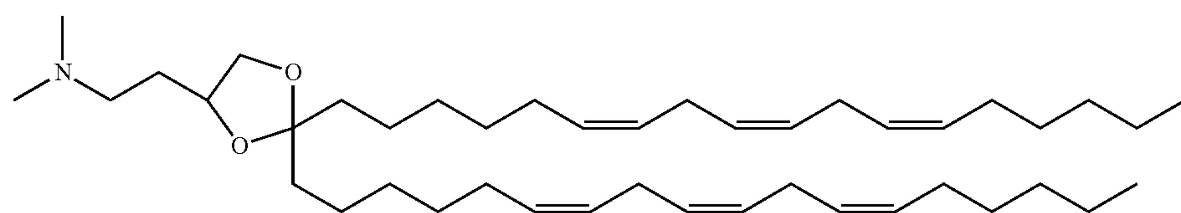
\gamma -DLen-C2K-DMA
