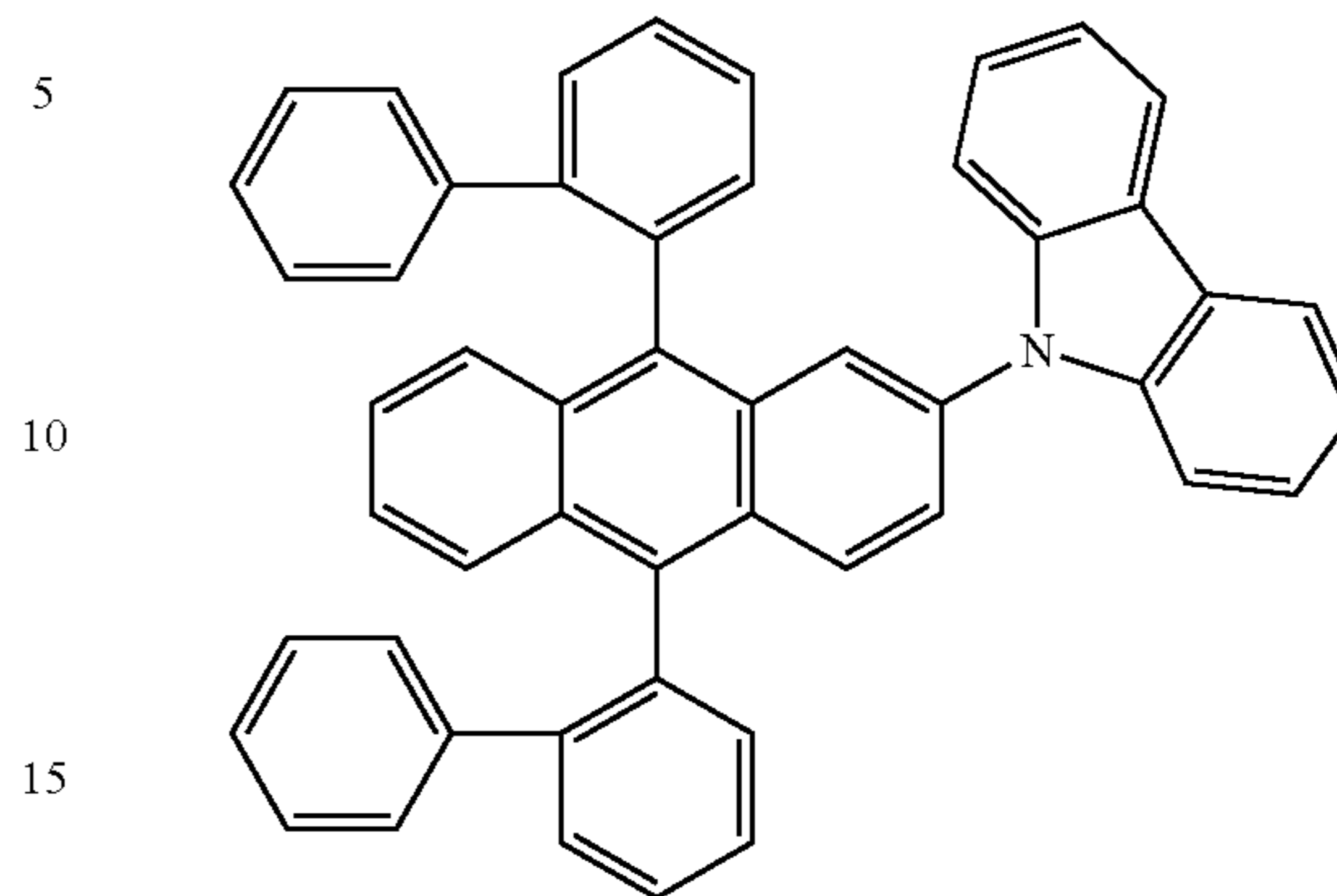
PCzBPhA
