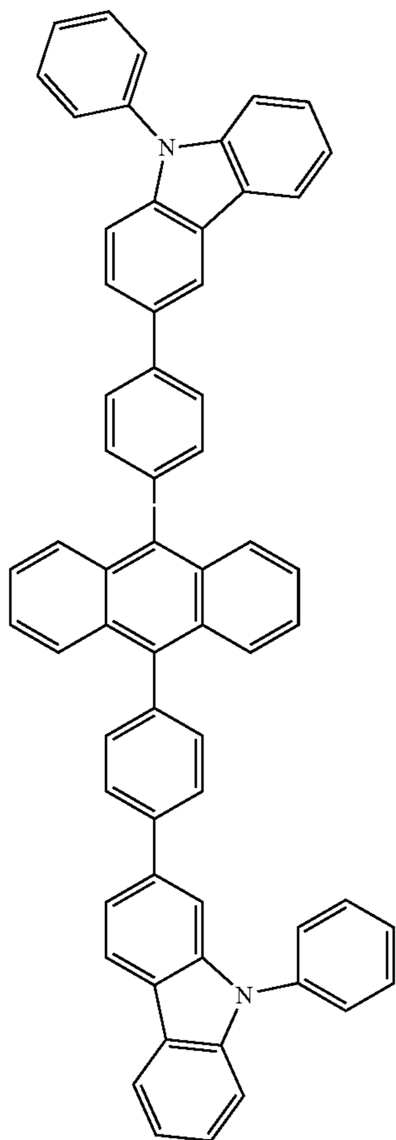
PCzBPA
