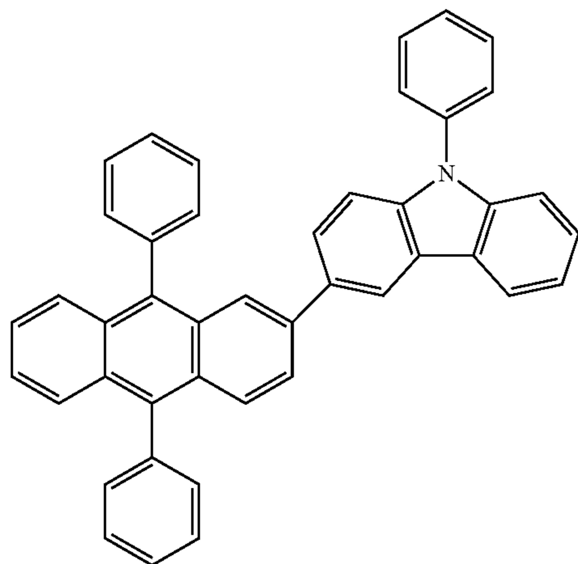
2PCzPA
