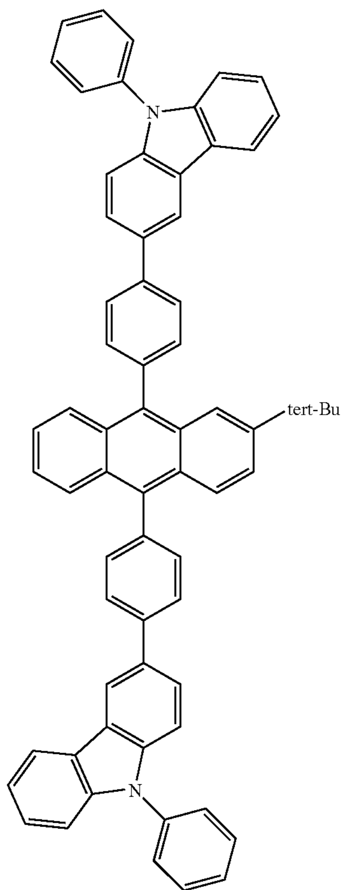
PCzBPA
