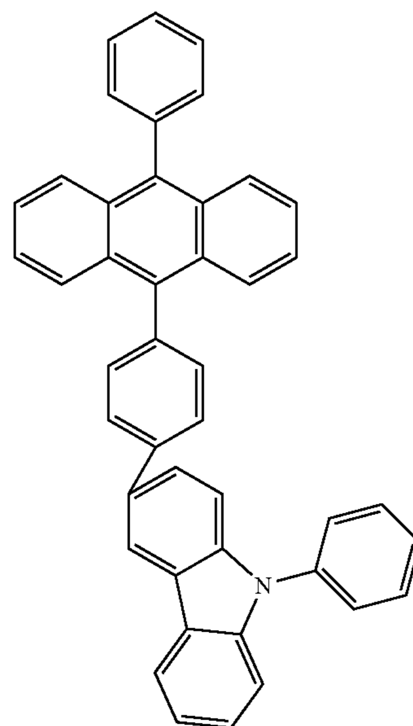
PCzPA
