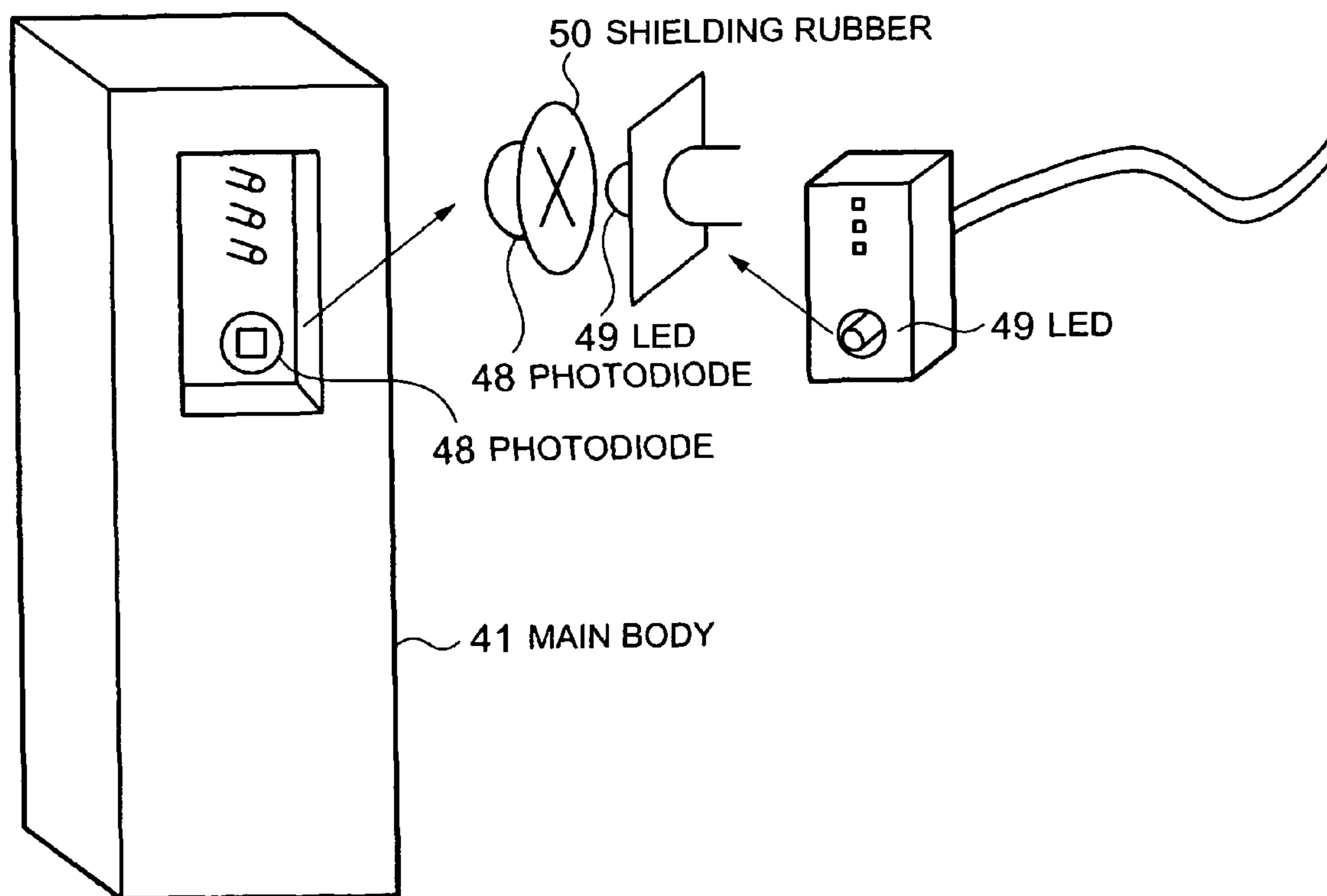
FIG. 18
