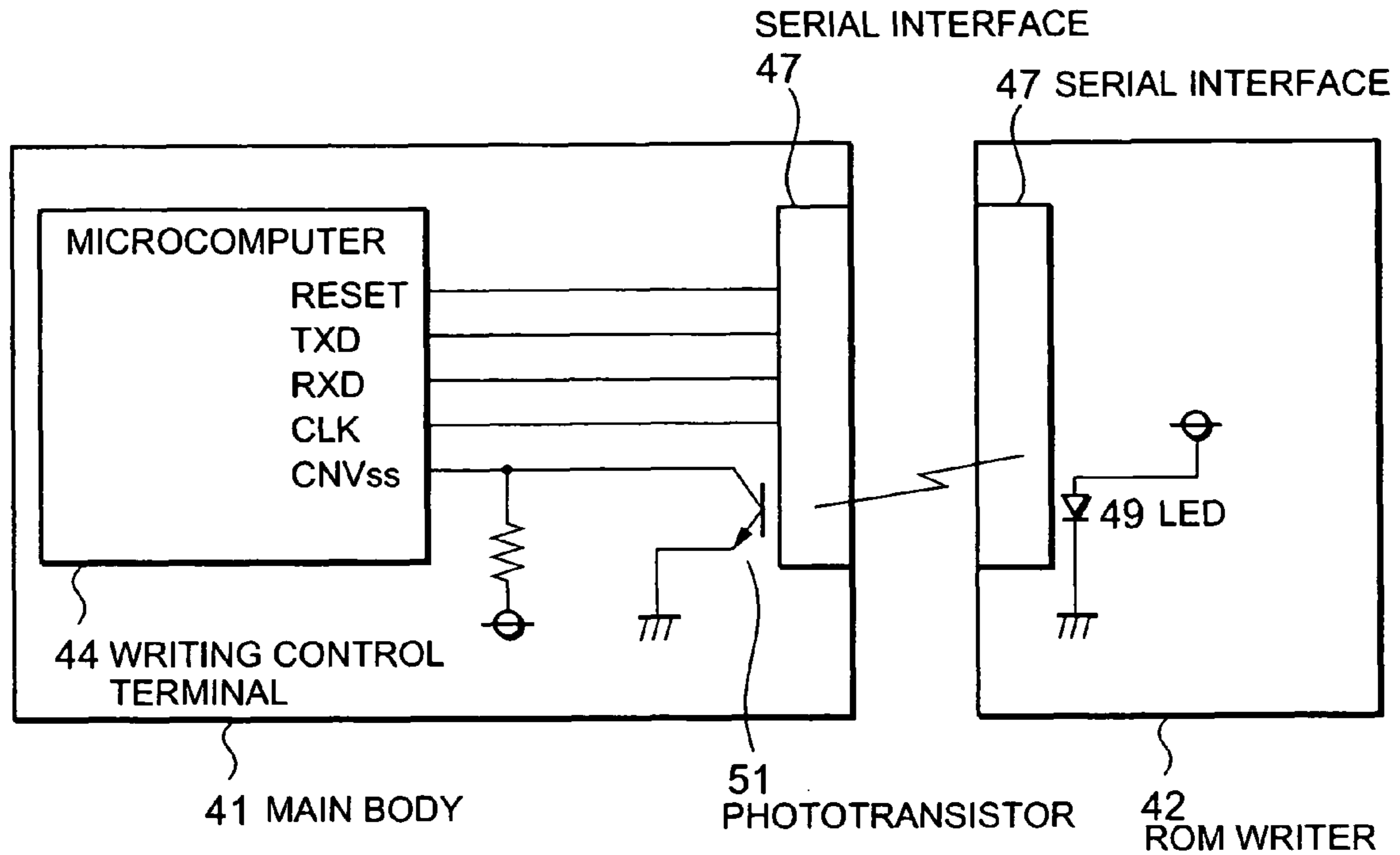
FIG. 19
