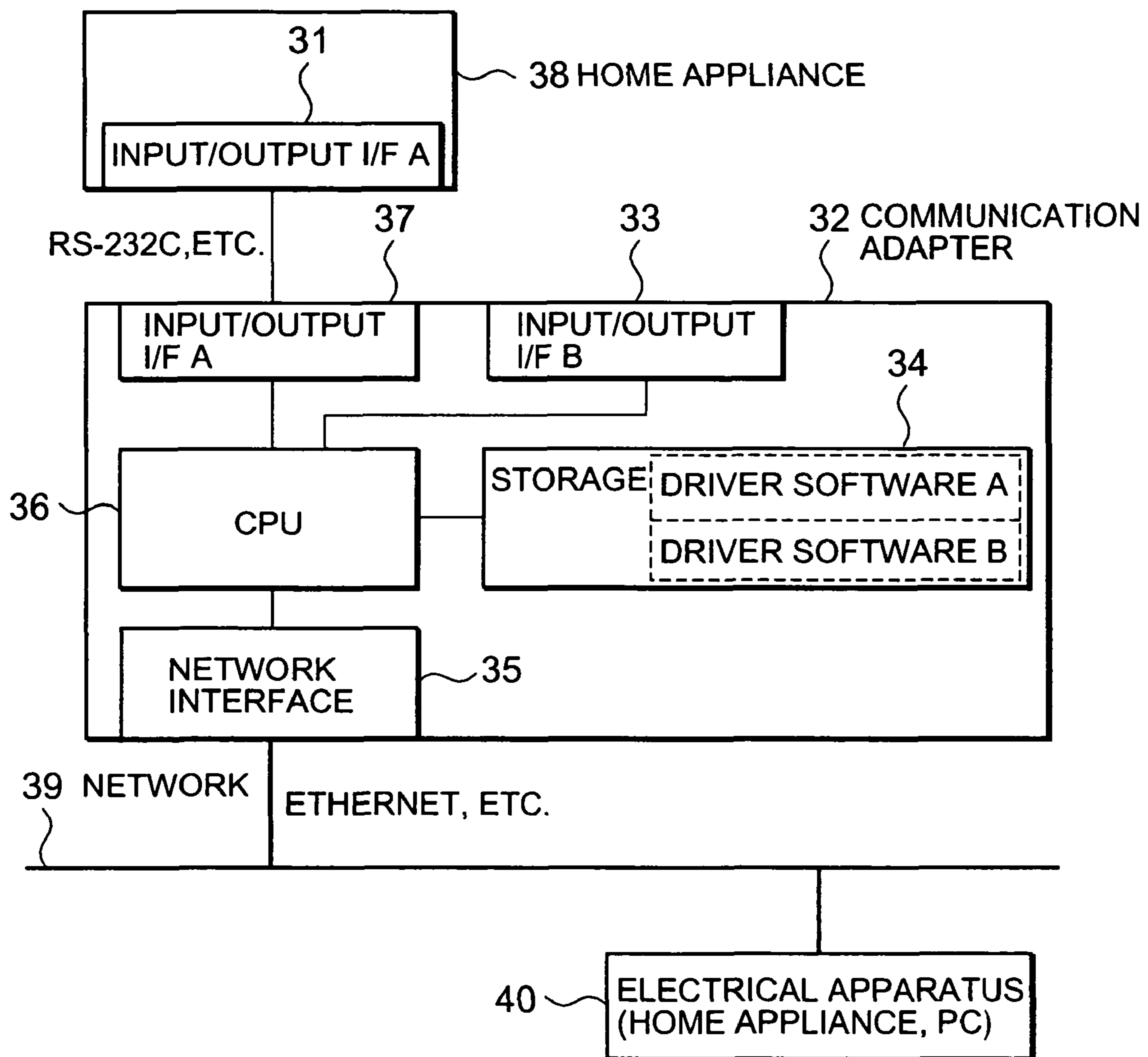
FIG. 10
