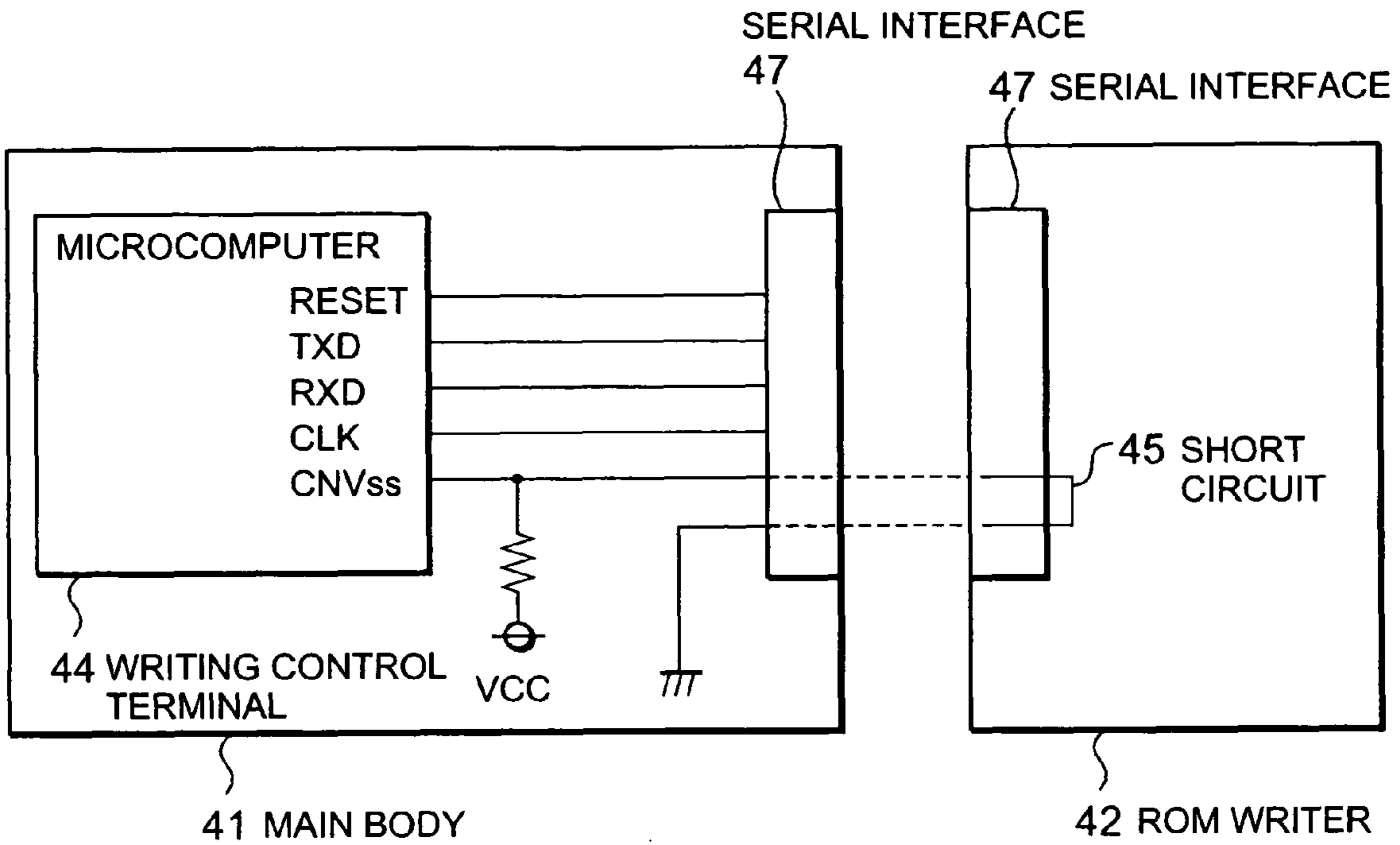
FIG. 15
