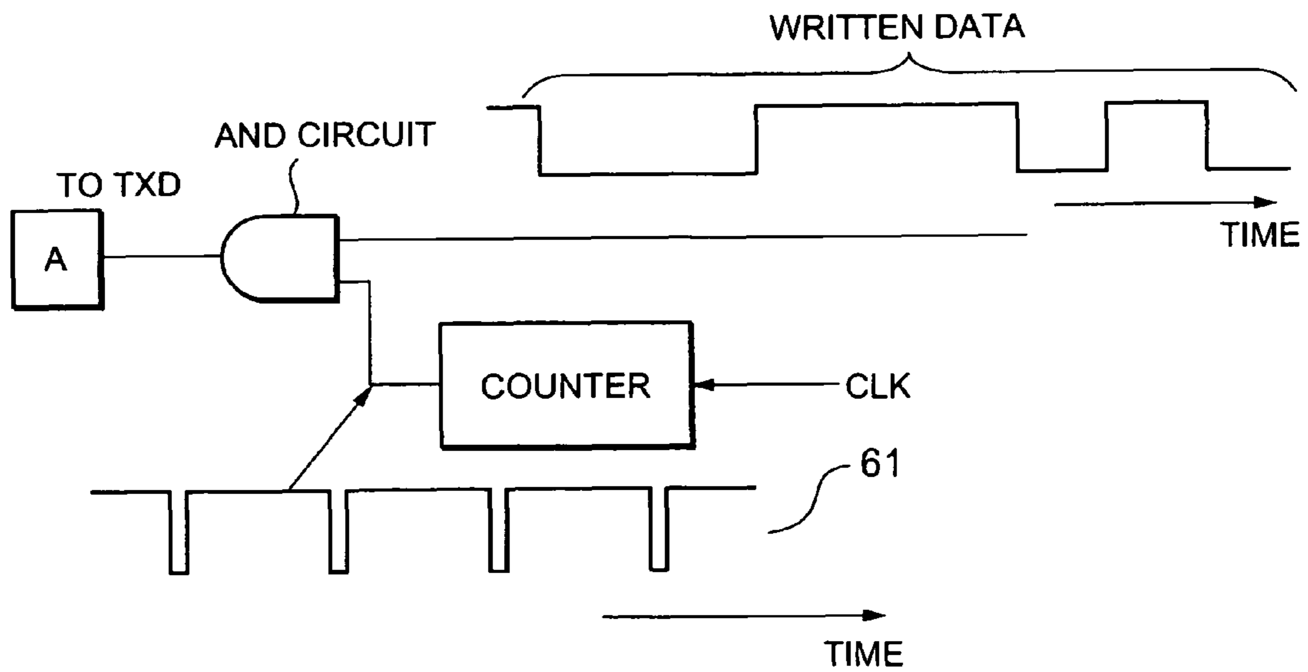
FIG. 24
