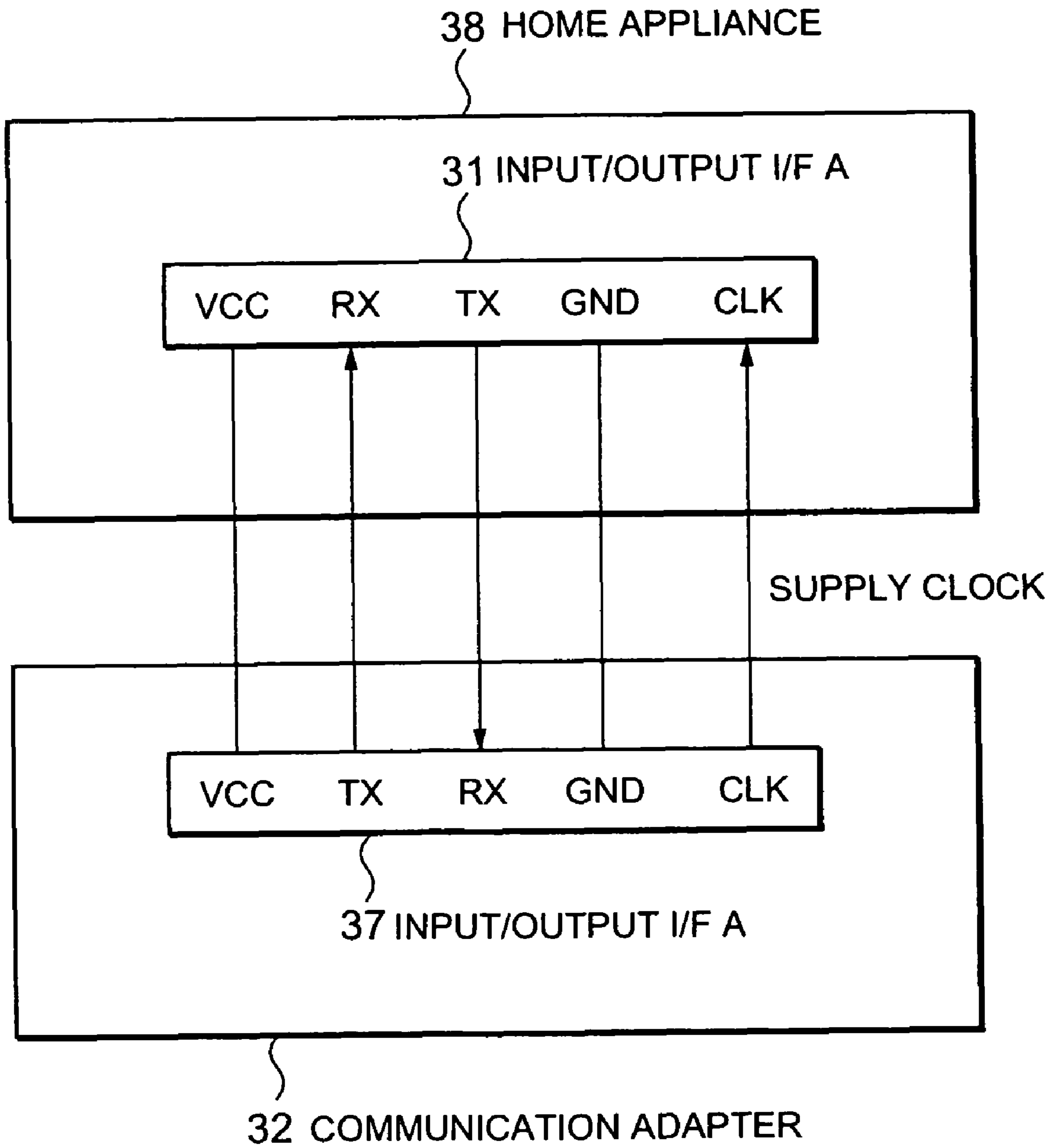
FIG. 12
