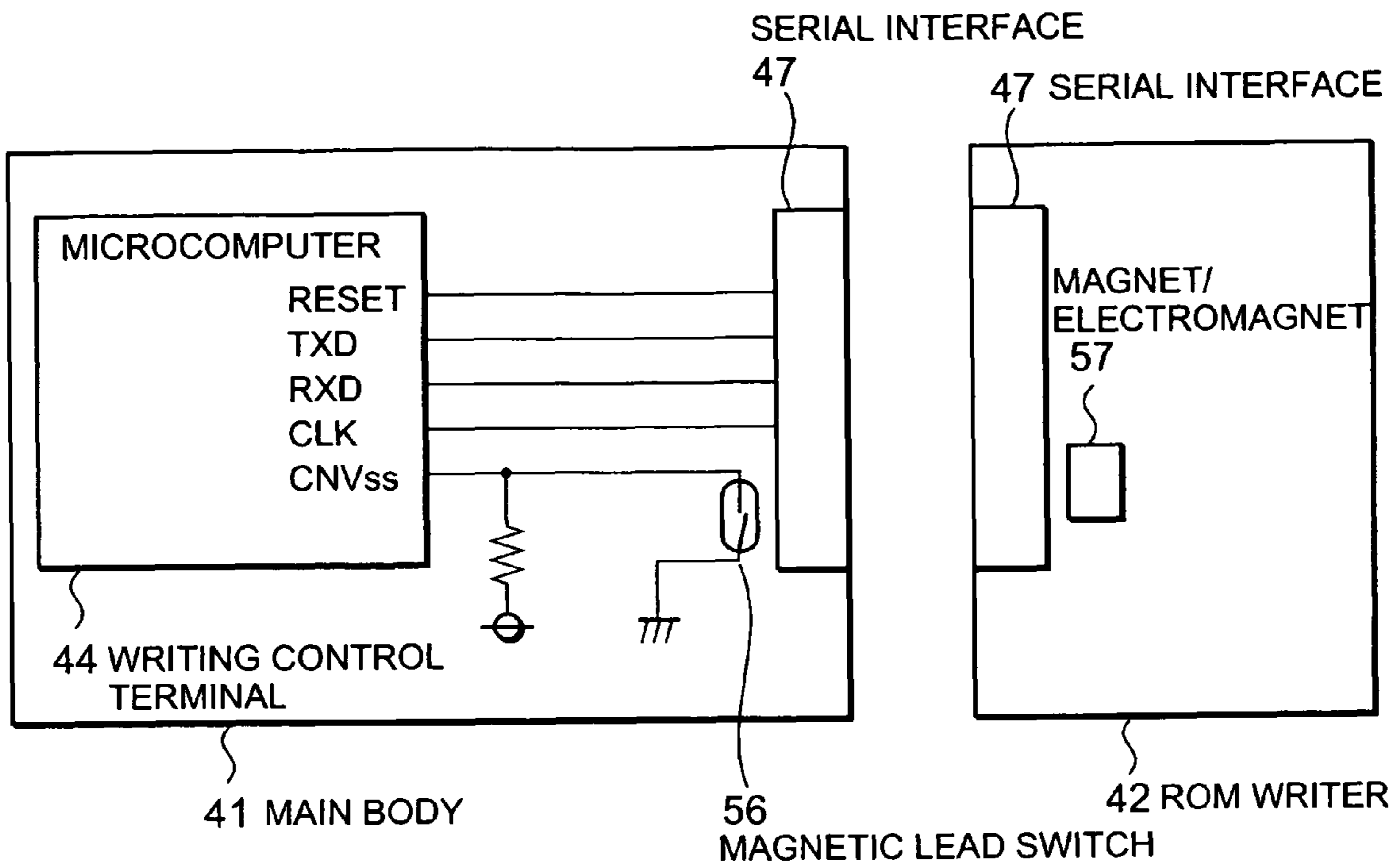
FIG. 23
