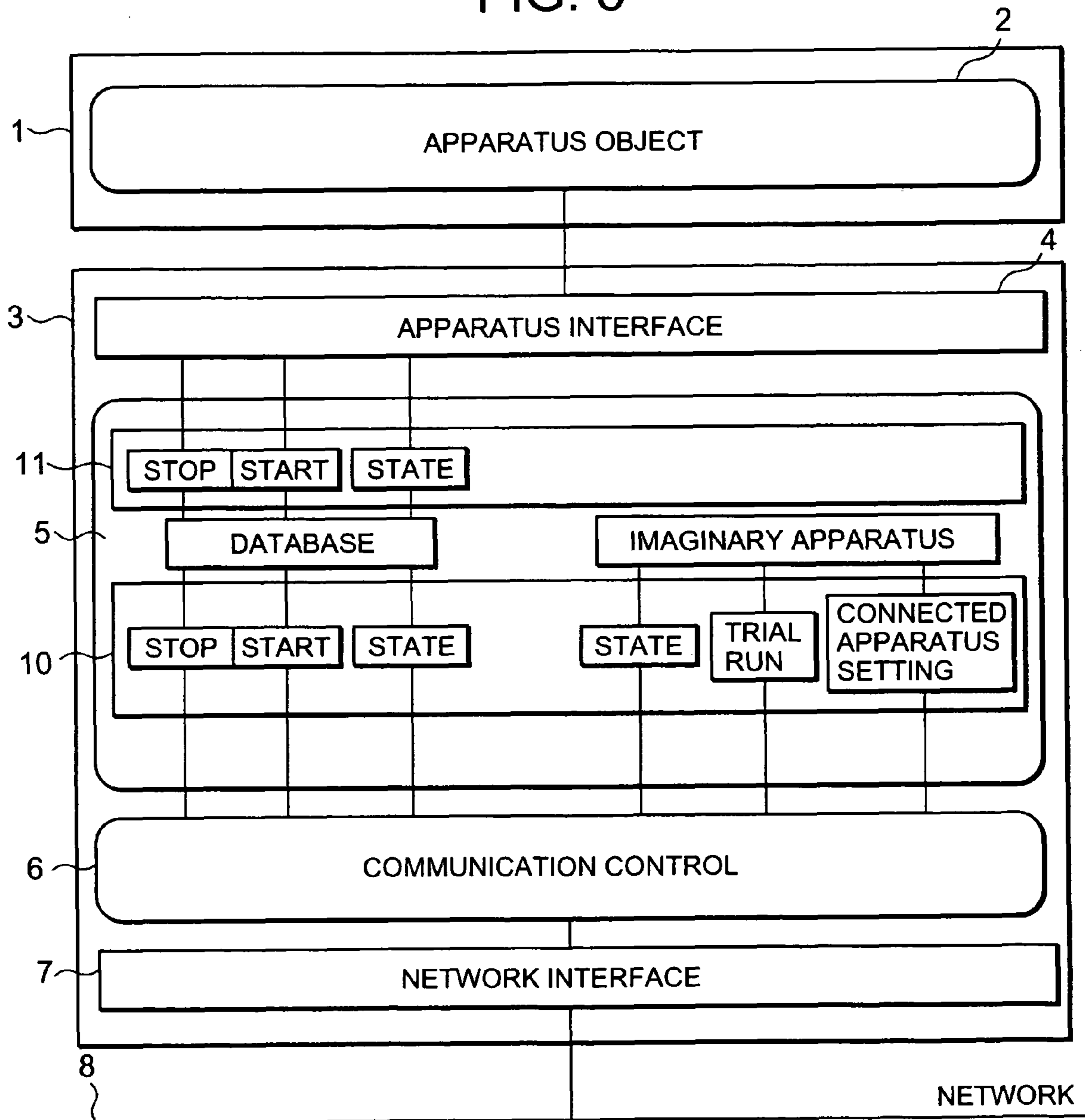
FIG. 5
