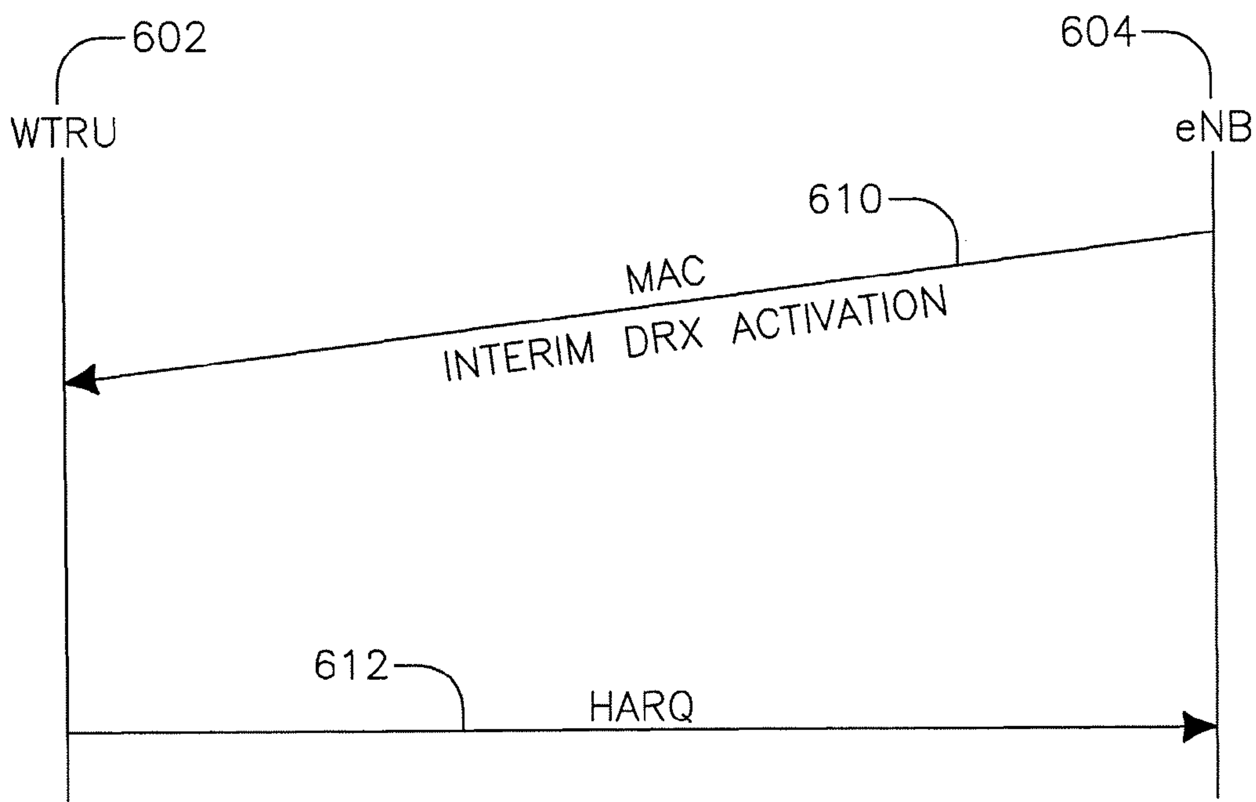
FIG.6B
