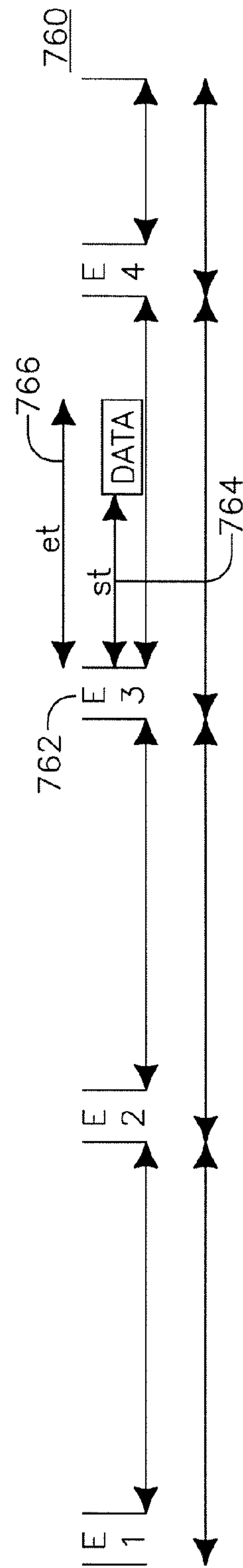
FIG. 7C
