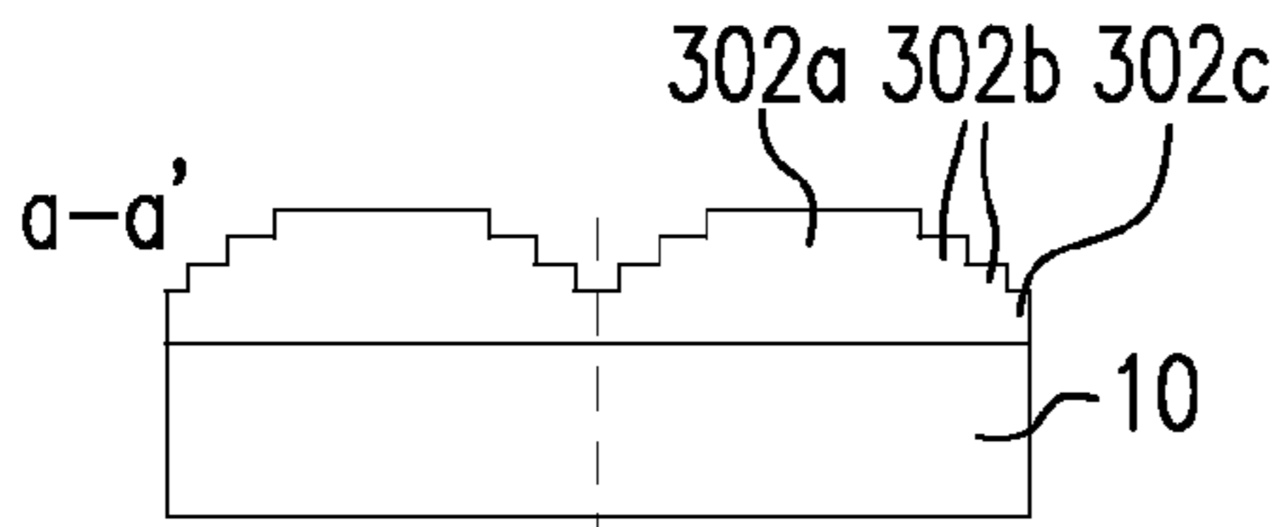
FIG. 5A-1
