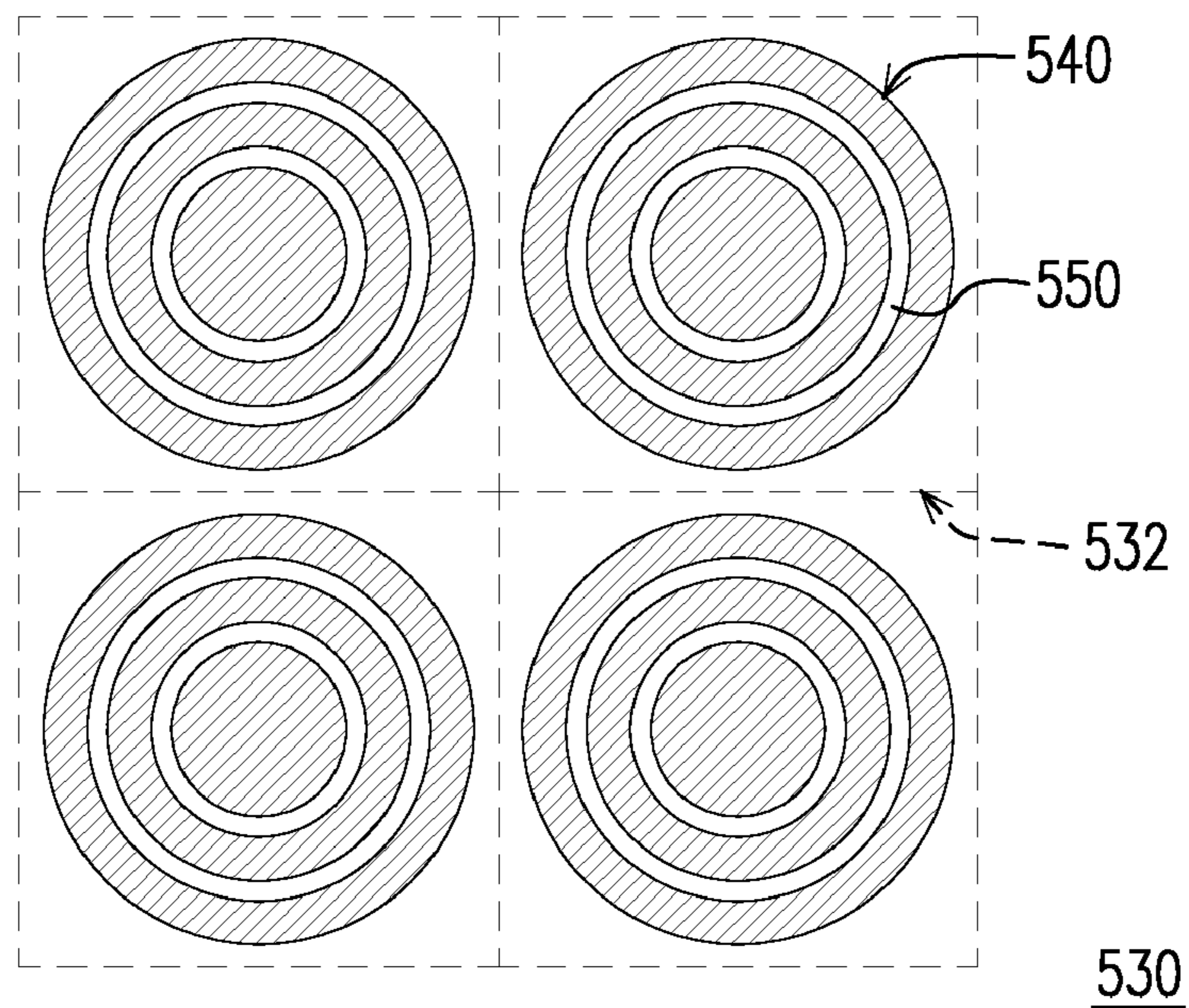
FIG. 6B
