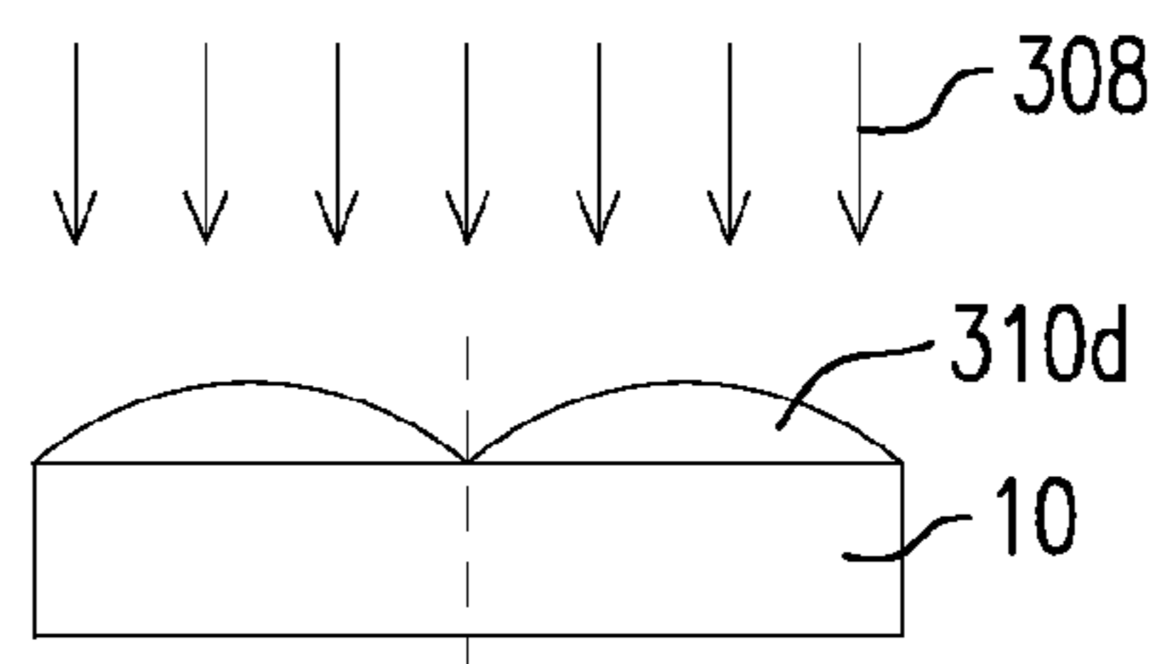
FIG. 5B-3
