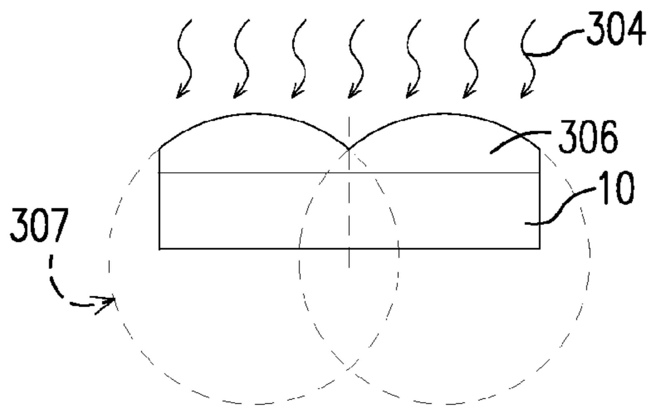
FIG. 5A-2
