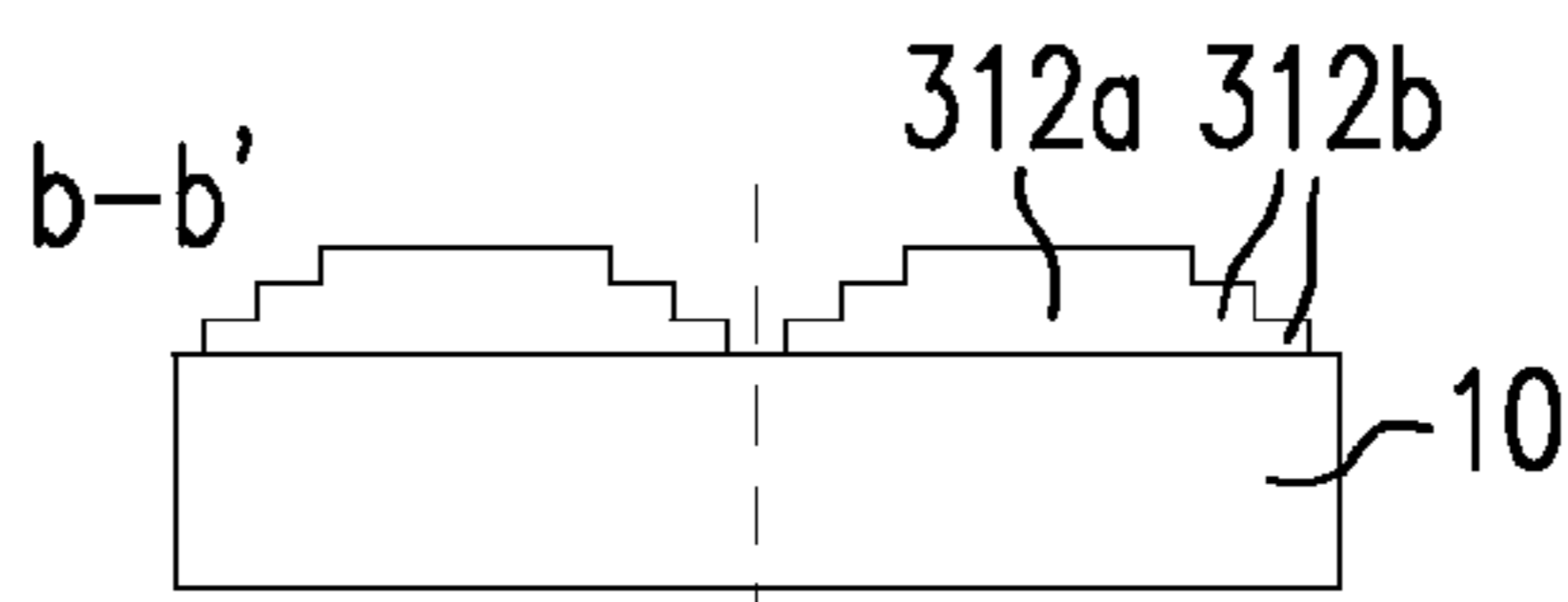
FIG. 5B-1
