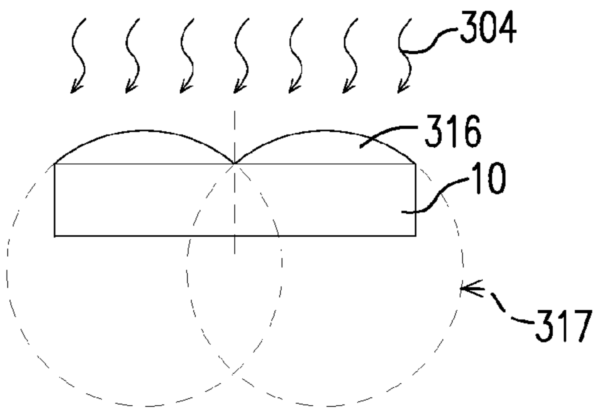
FIG. 5B-2
