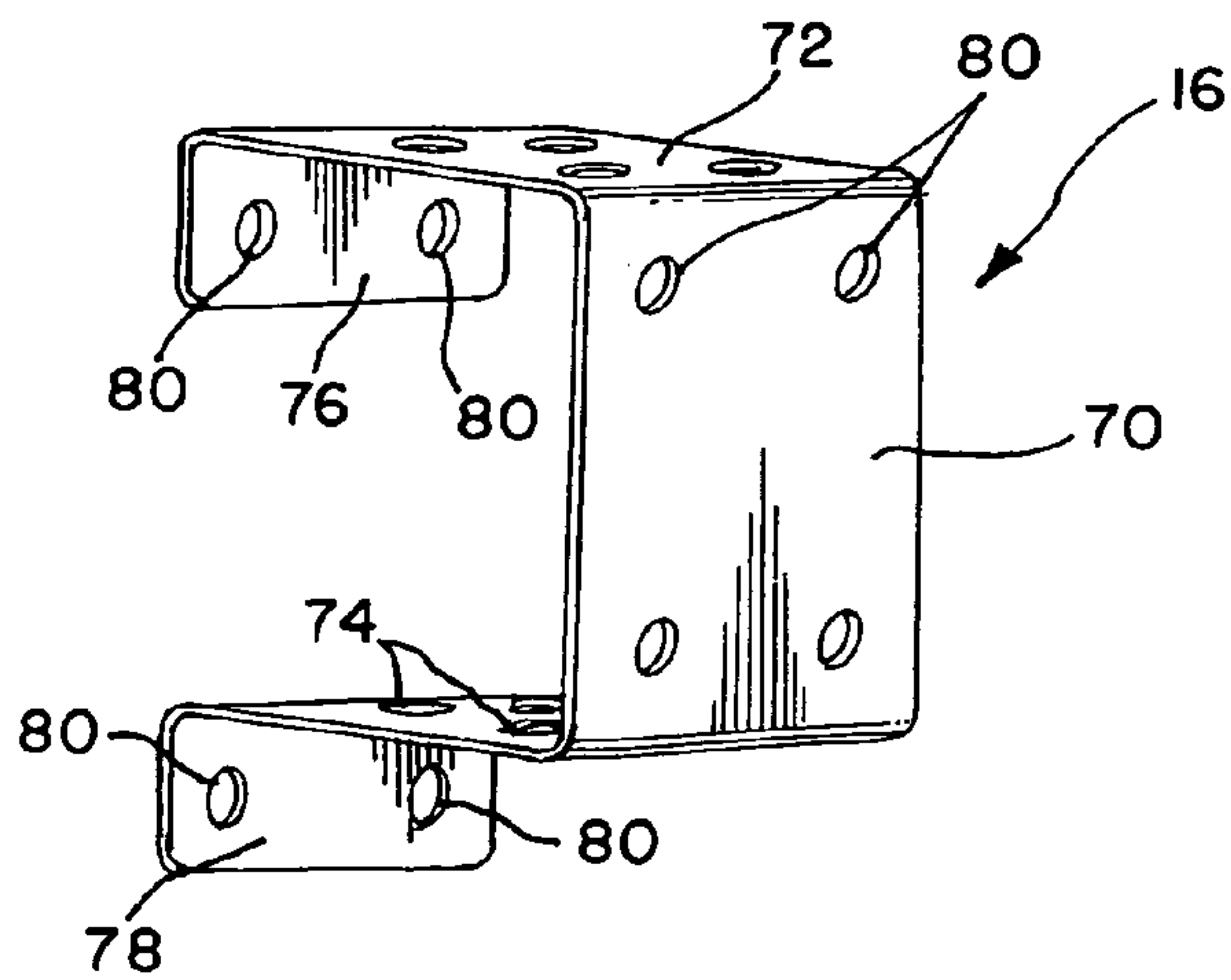
FIG. 4
