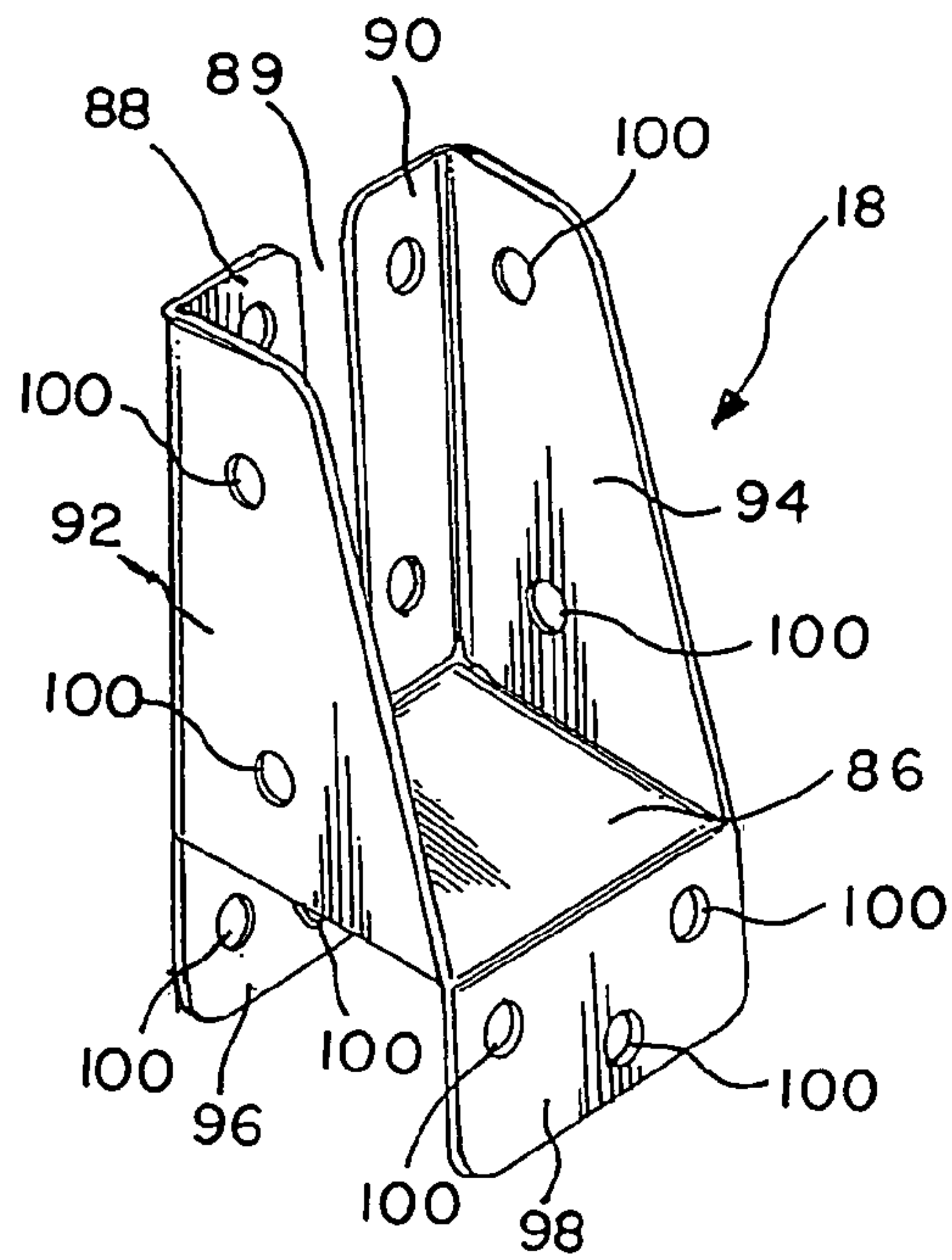
FIG. 5
