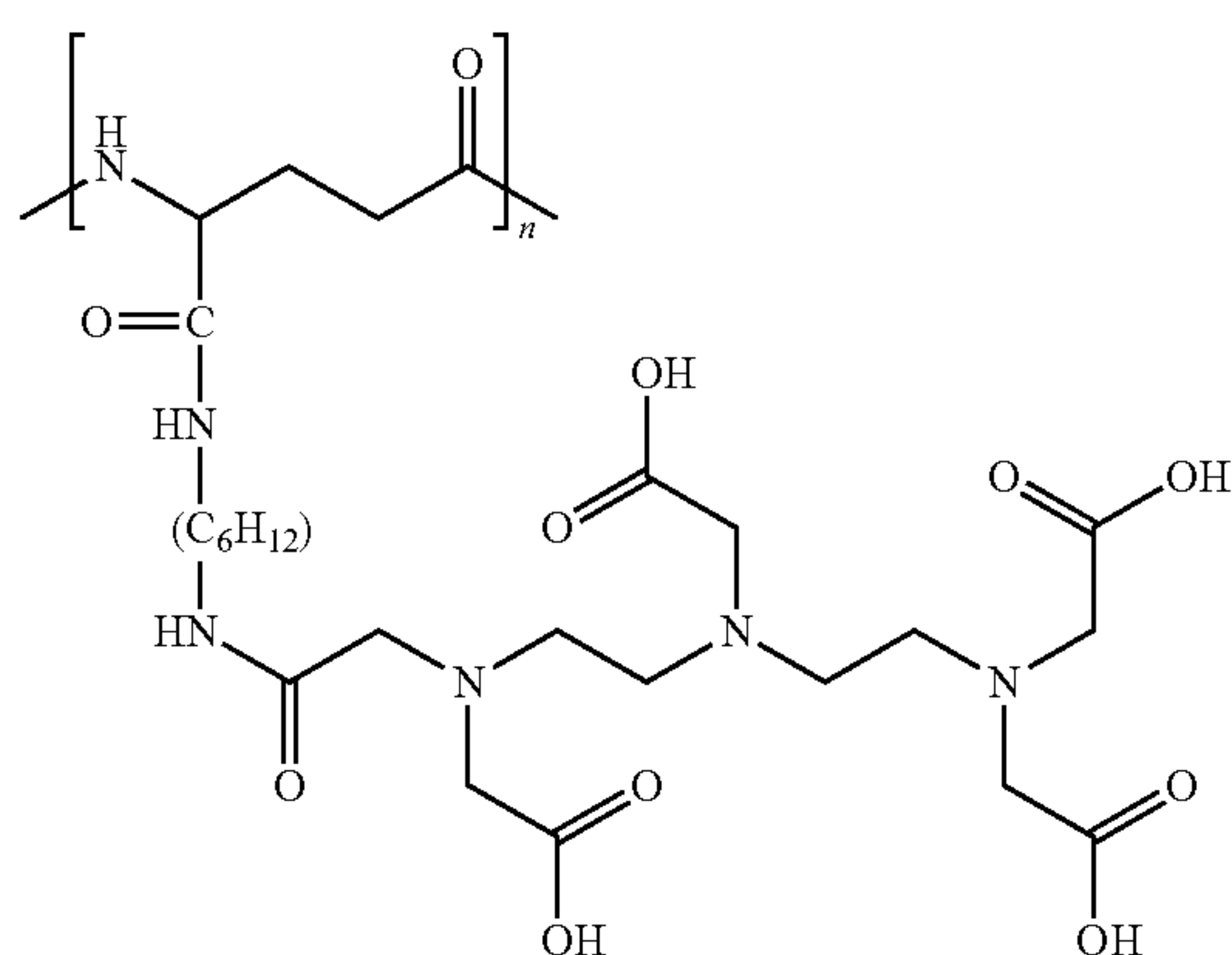
(γ-PGA)-DTPA
