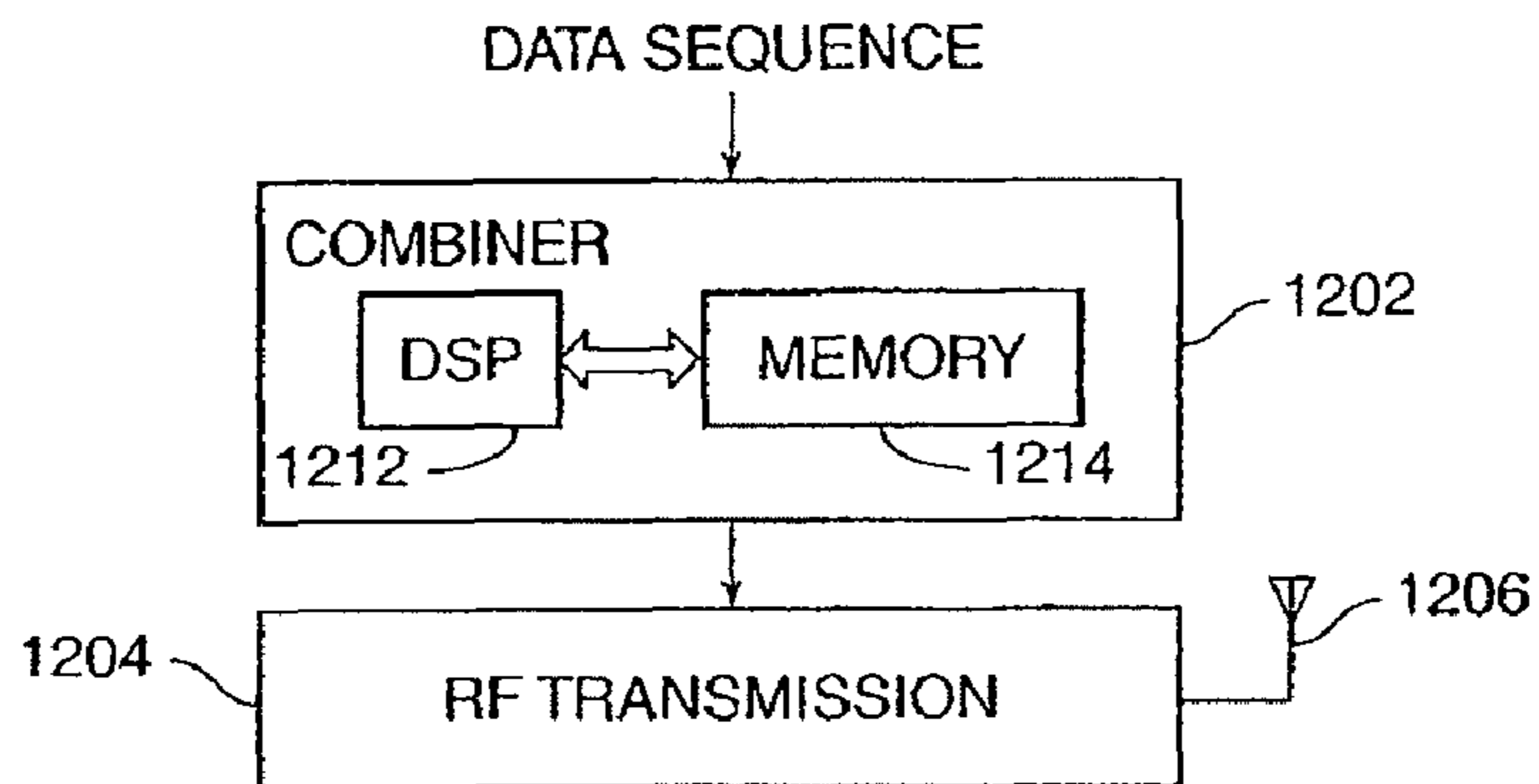
FIG. 12
