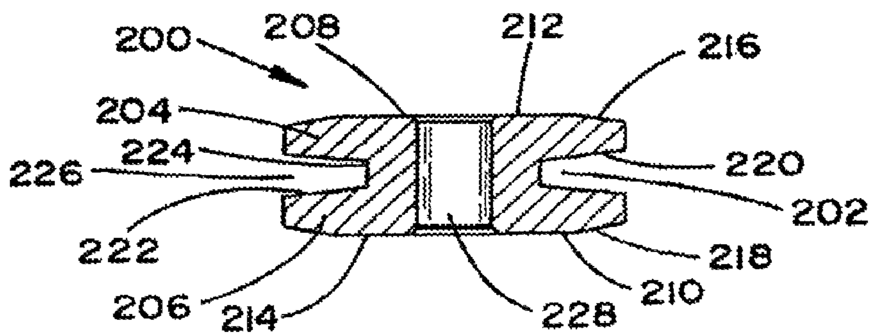
Section A-A
