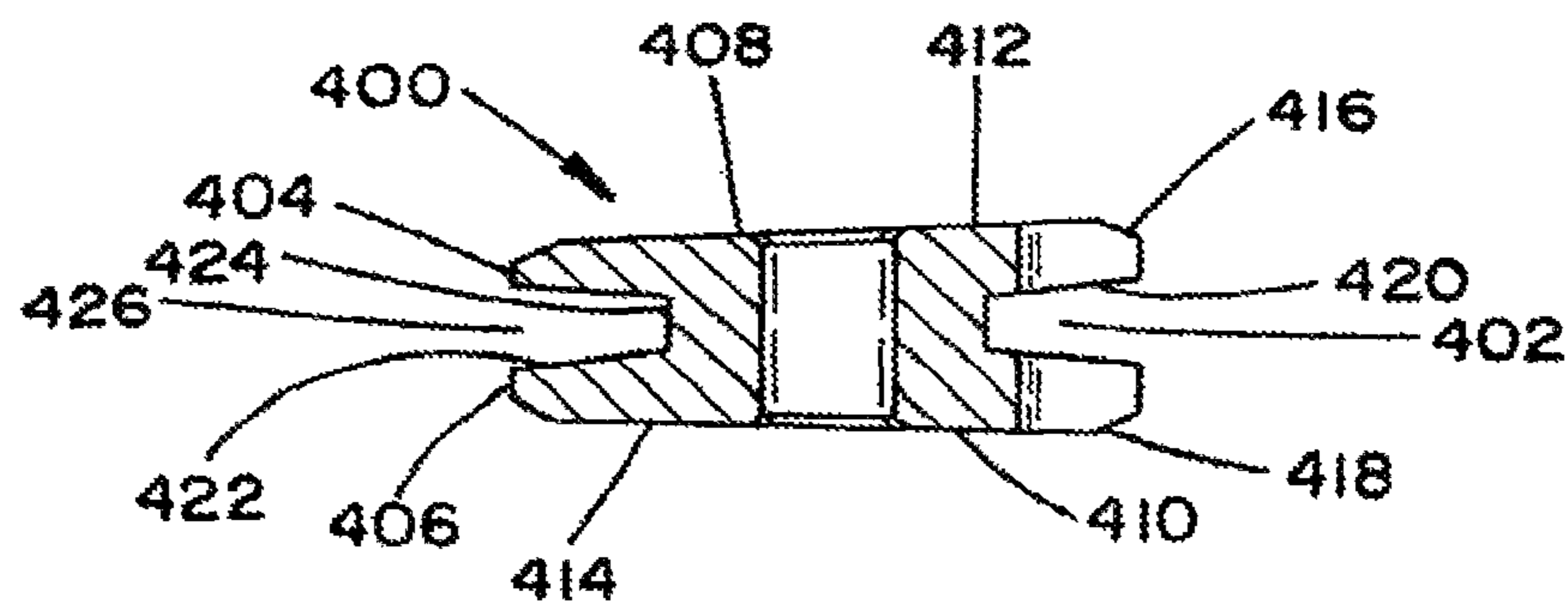
Section A-A
