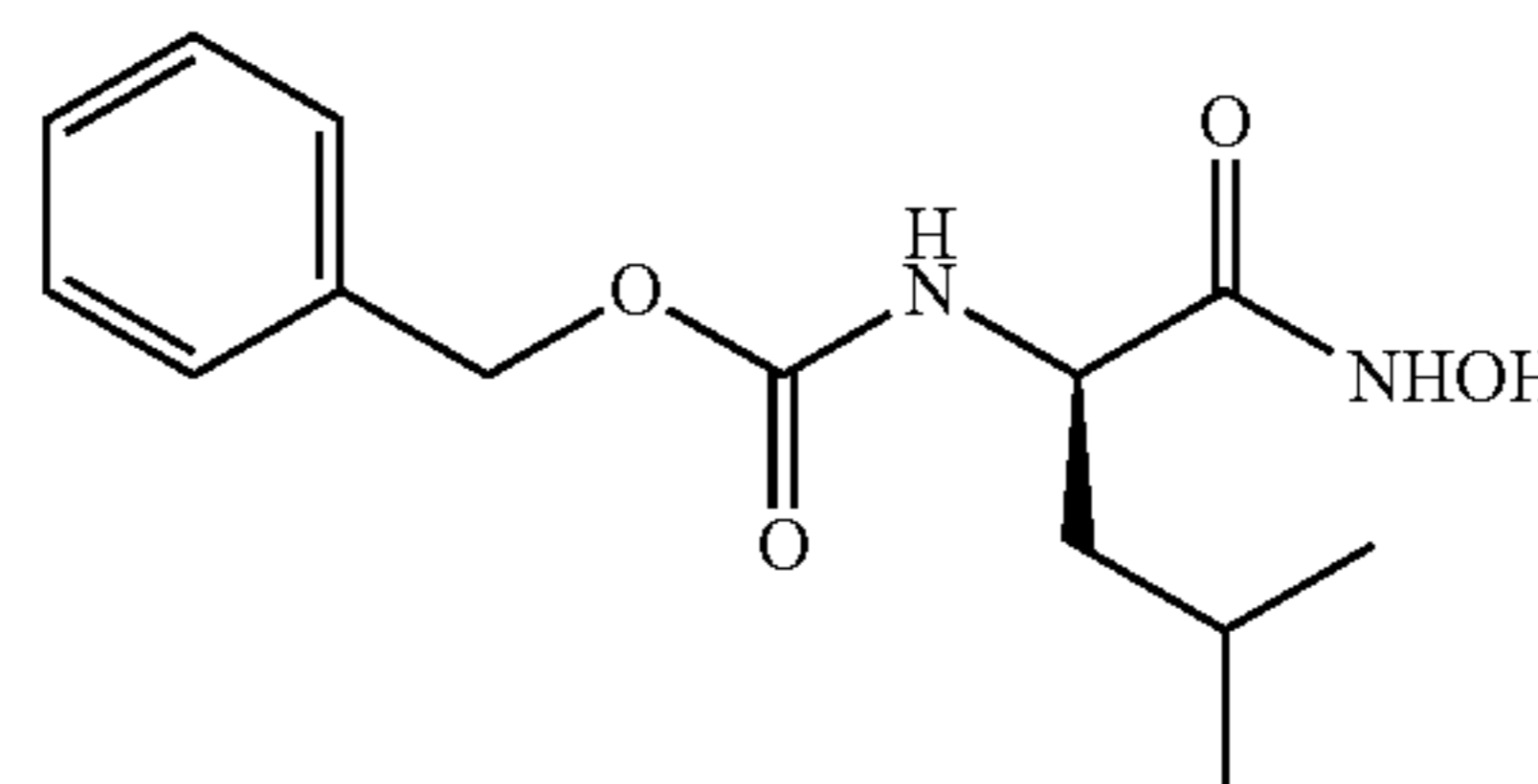
N-Cbz-Leu-NHOH
