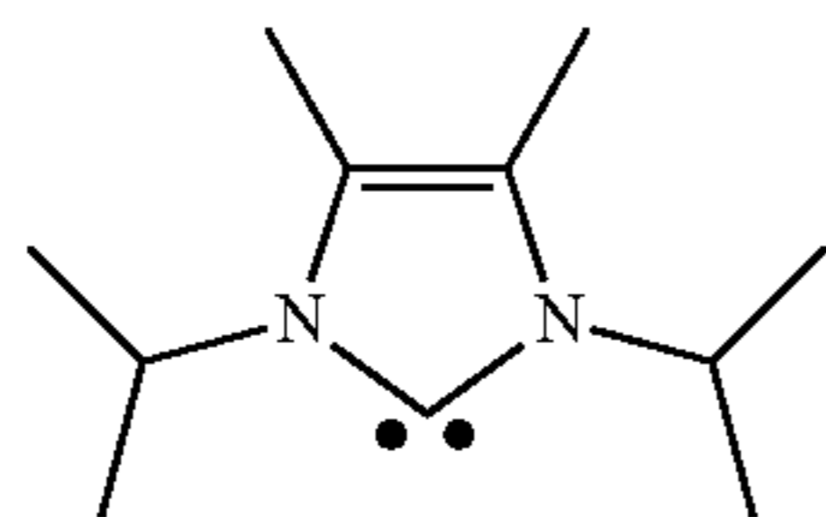
1,3-Bis(2-propyl)-4,5-dimethylimidazol-2-ylidene (Im-1)
