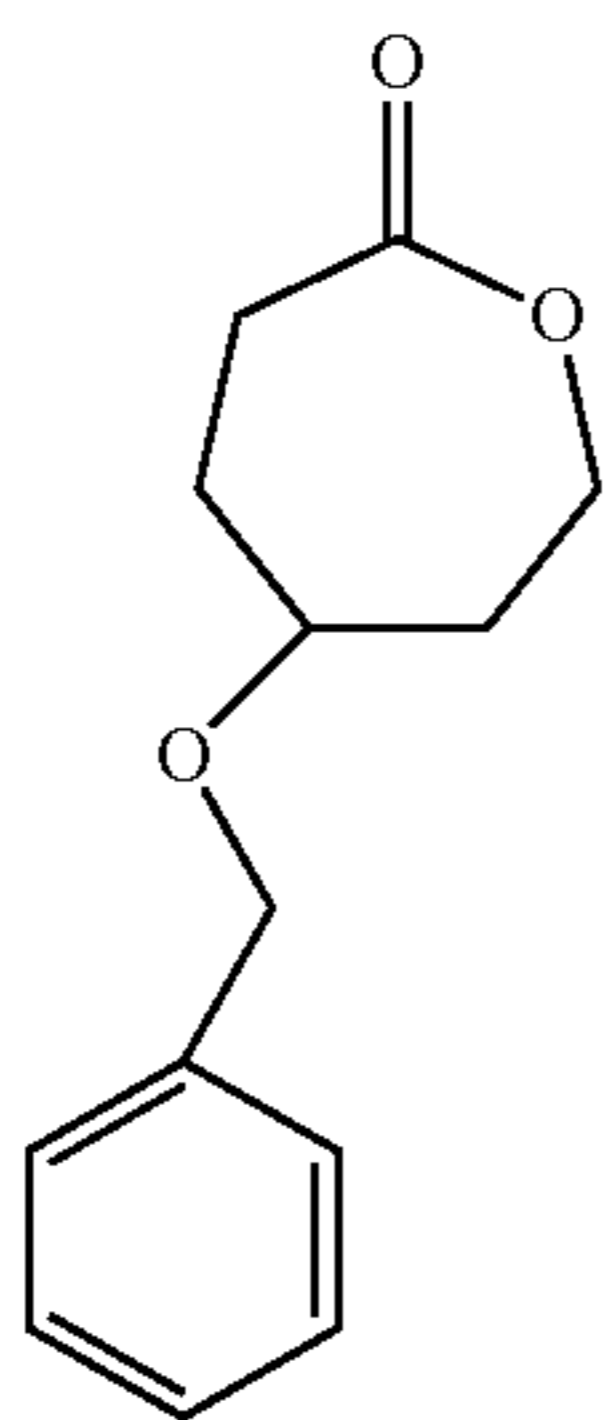
5-(Benzyloxy)oxepan-2-one (BXO)
