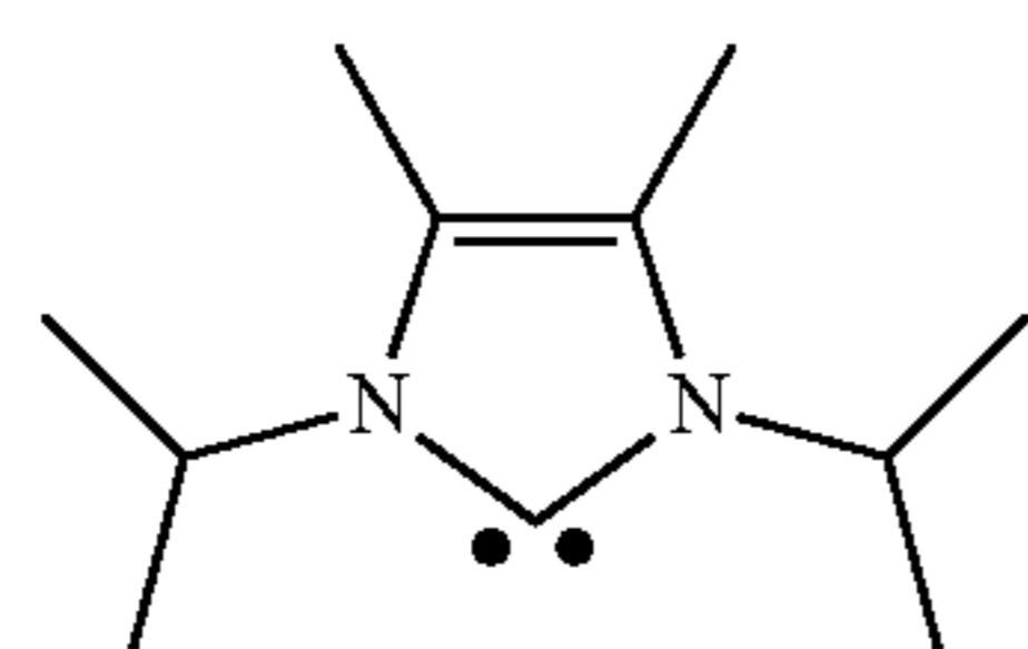
1,3-Bis(2-propyl)-4,5-dimethylimidazol-2-ylidene (Im-1)
