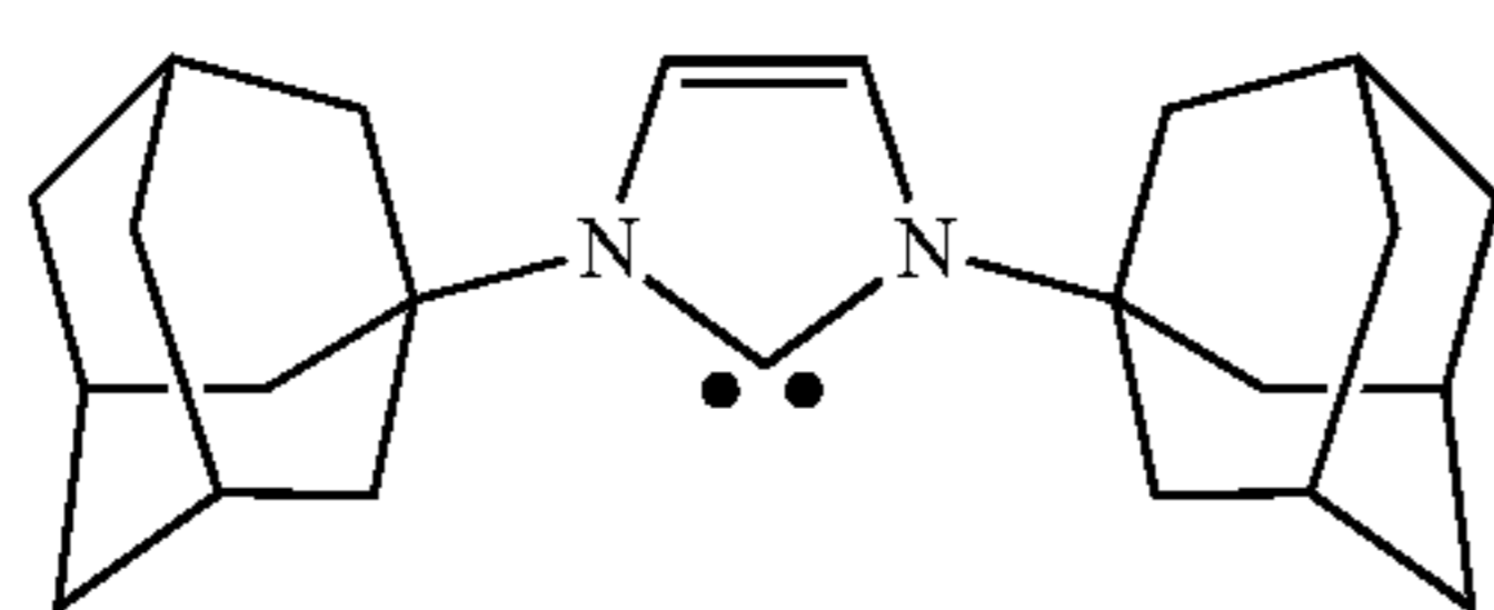
1,3-Bis(1-adamantyl)imidazol-2-ylidene (Im-4)
