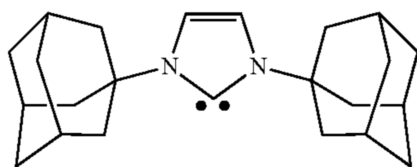
1,3-Bis(1-adamantyl)imidazol-2-ylidene (Im-4)
