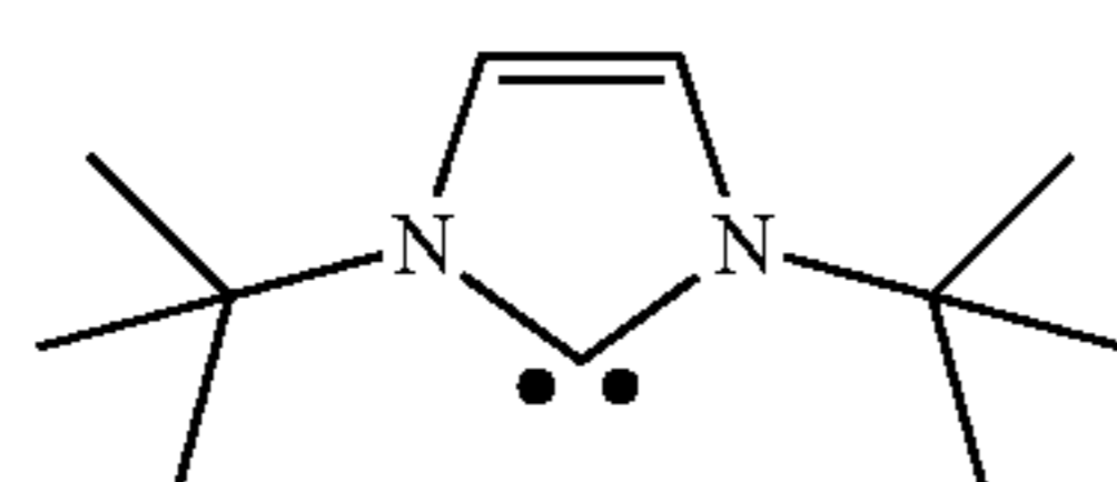
1,3-Di-t-butylimidazol-2-ylidene (Im-6)
