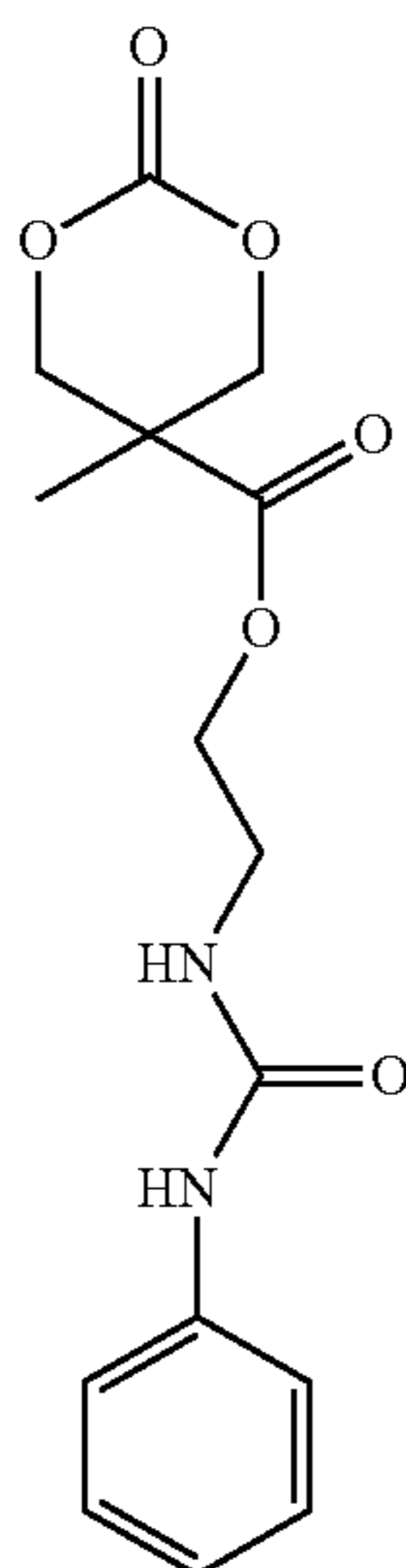
(MTCU)
