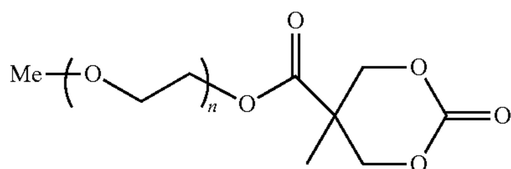
(MTCOMPEG)
