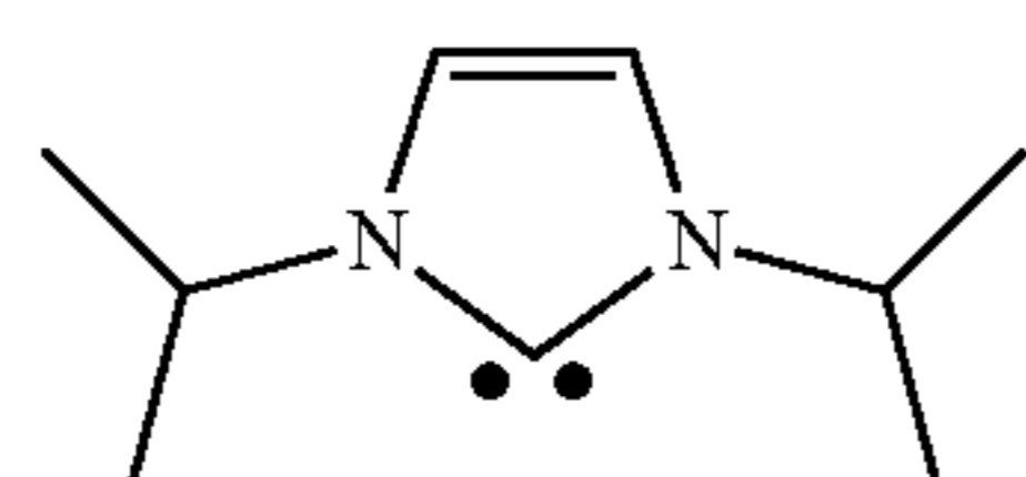
1,3-Di-i-propylimidazol-2-ylidene (Im-5)
