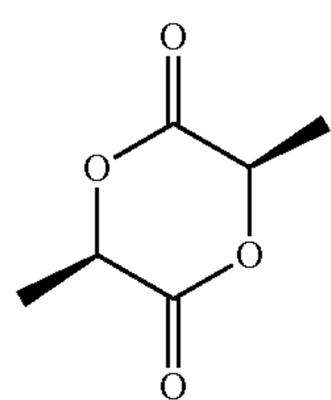
L-Lactide (LLA)
