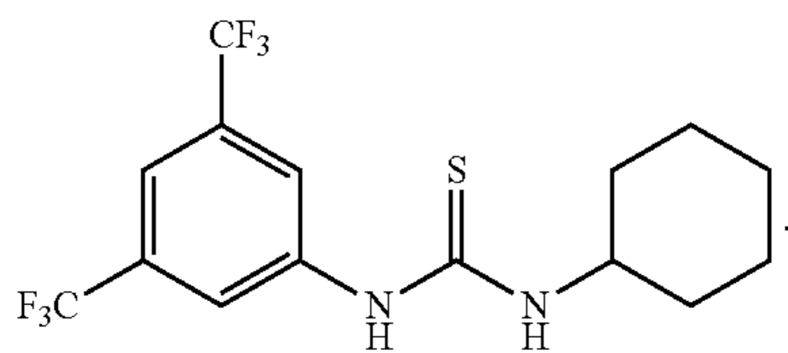
(TU)
