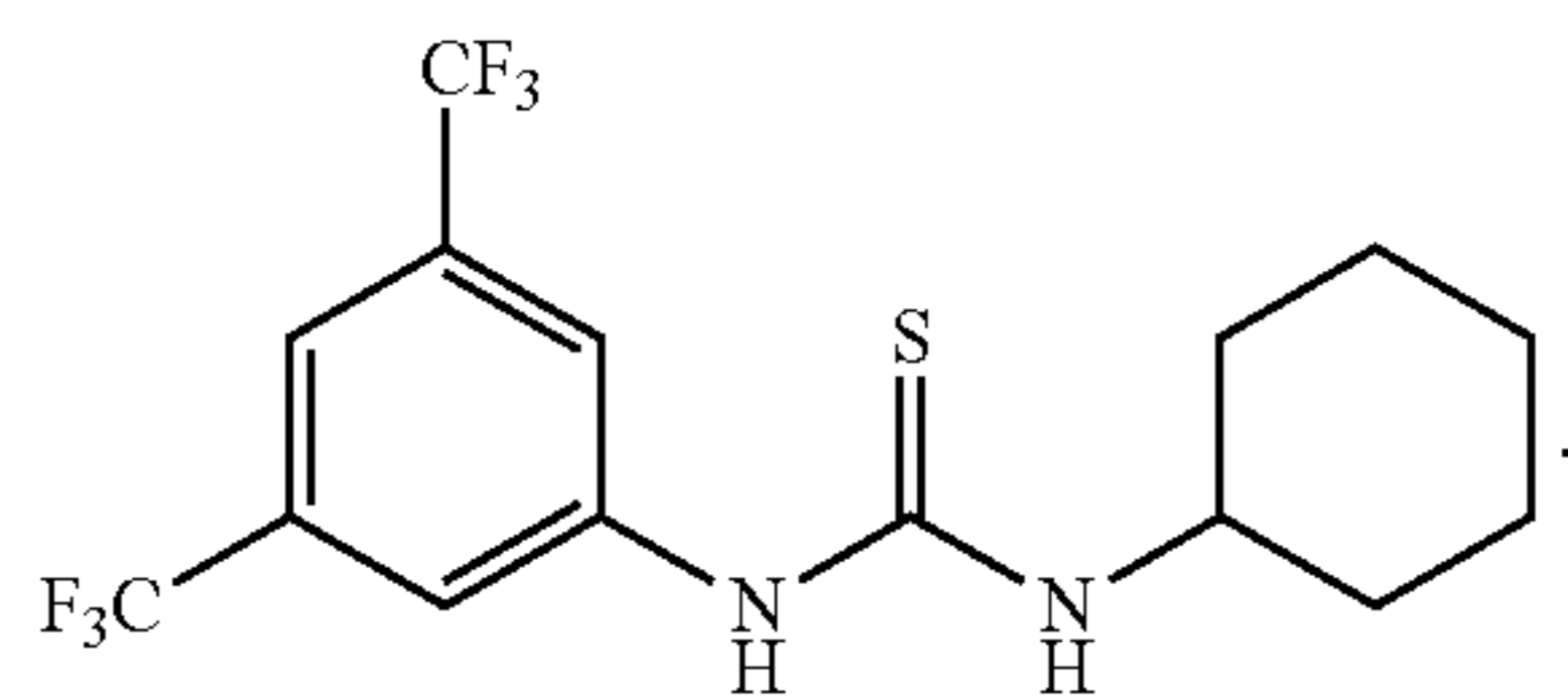
(TU)
