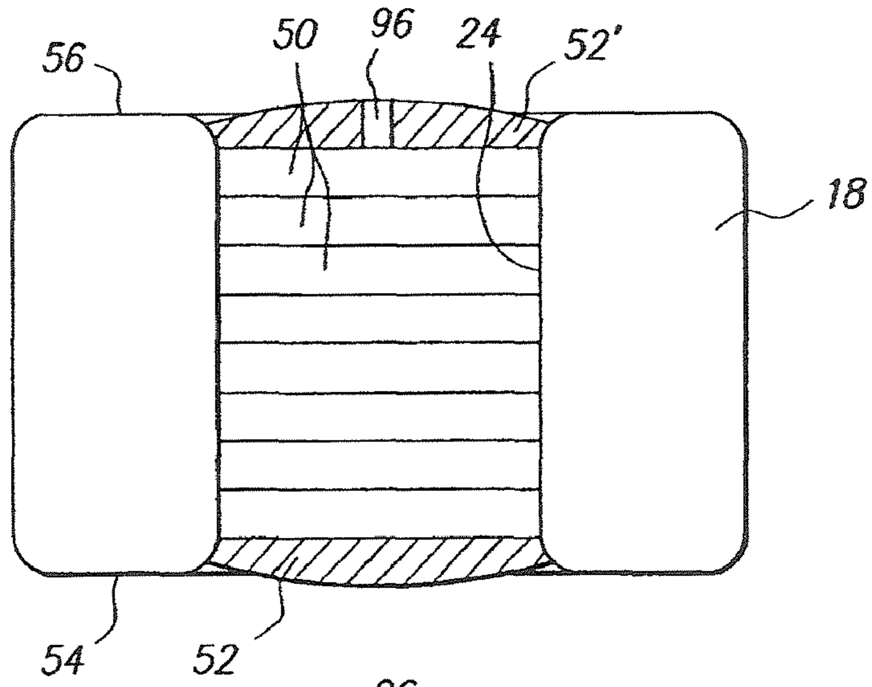
FIG. 18A
