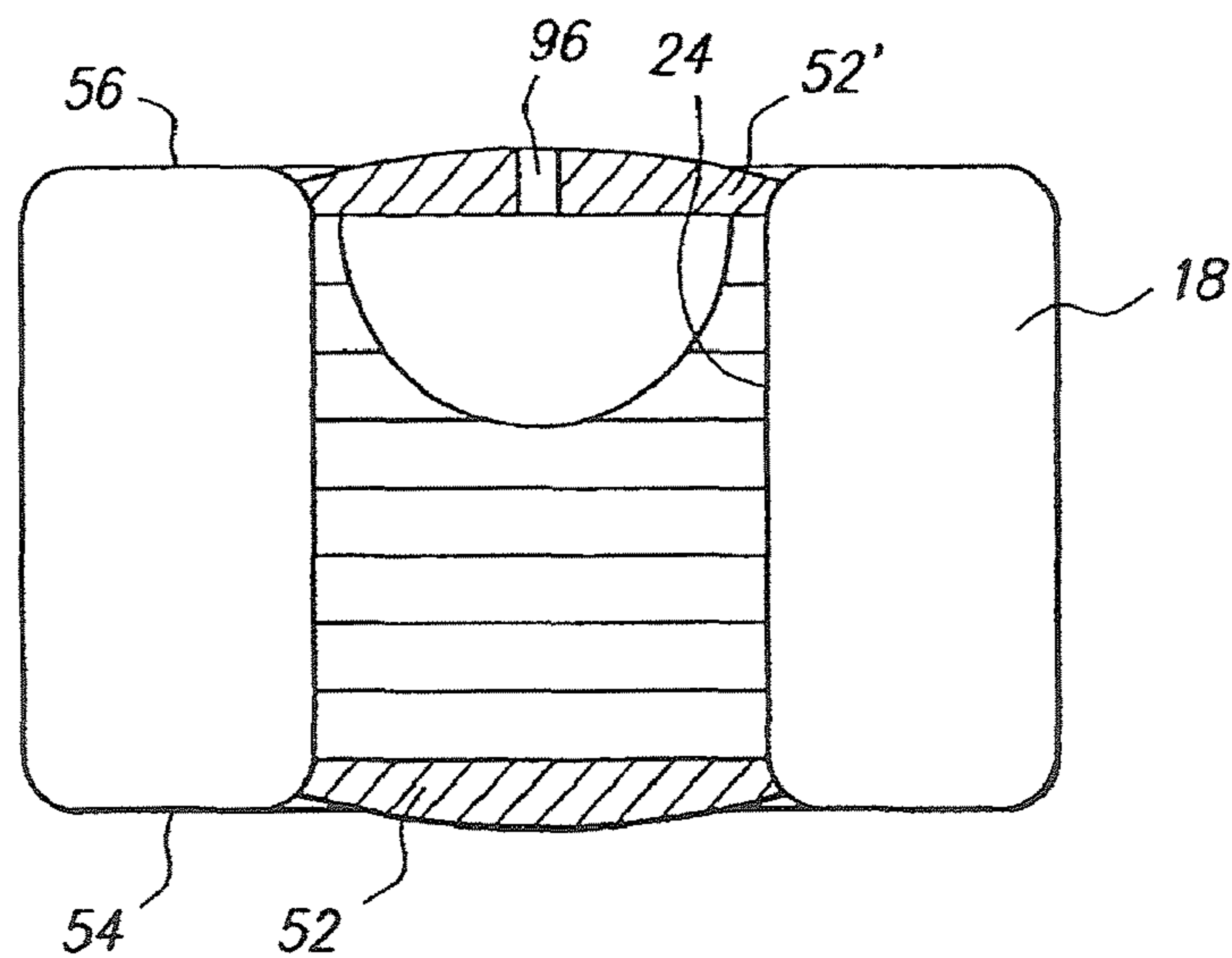
FIG. 18C
