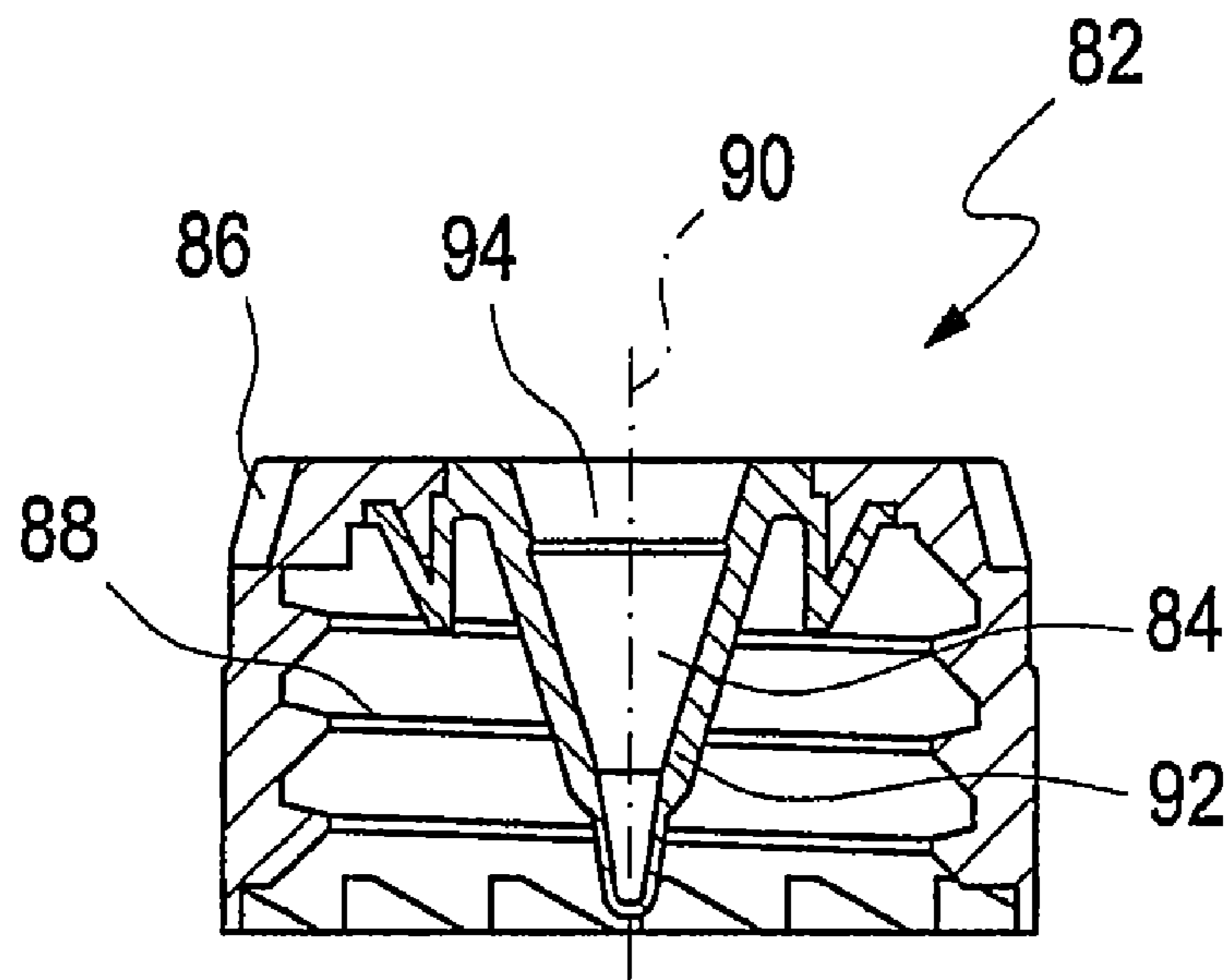
Fig. 8A
