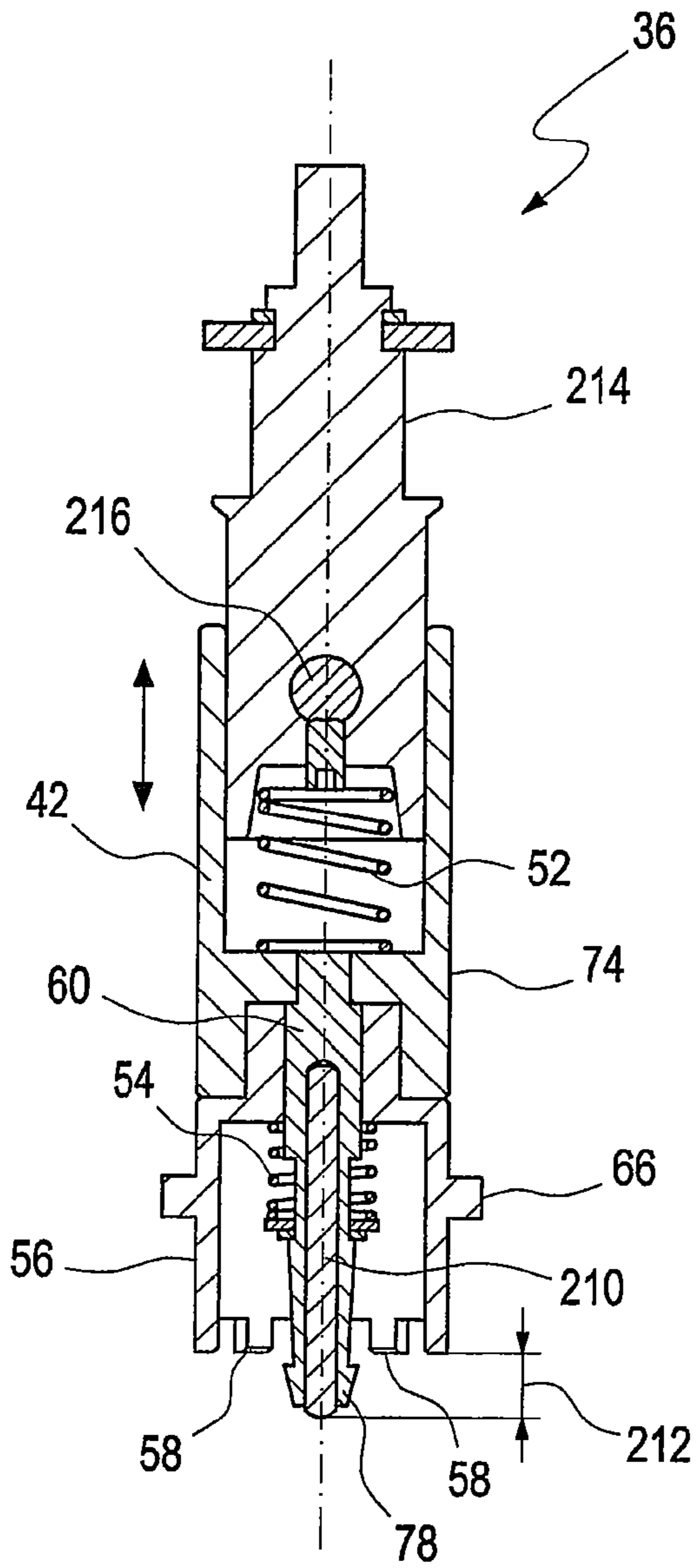
Fig. 12C
