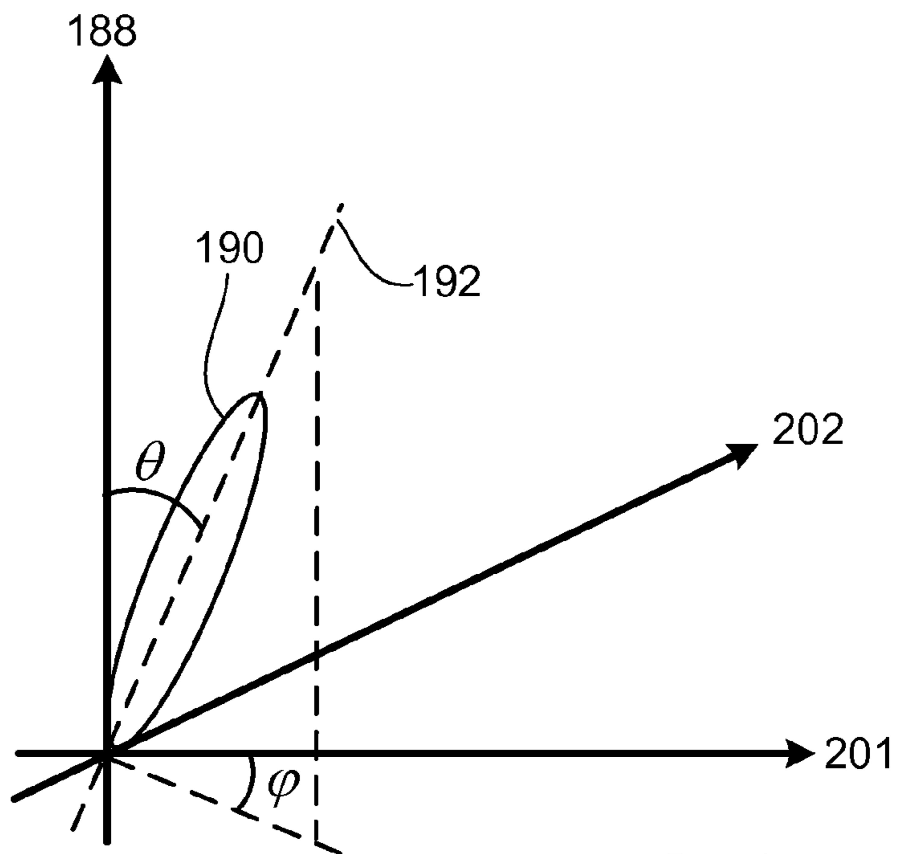
FIG. 2B
