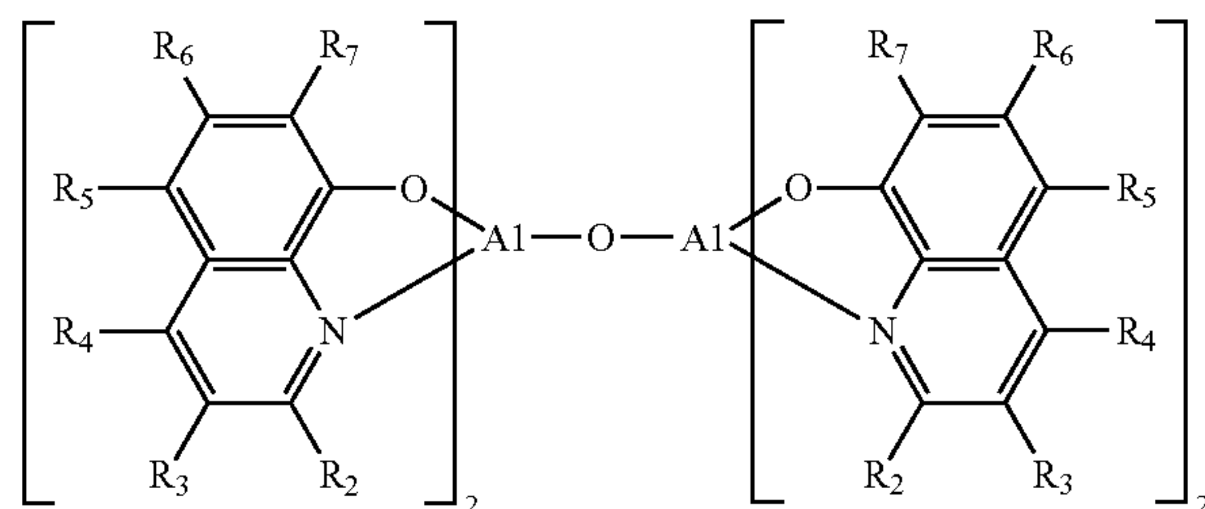
[Chem 3]
