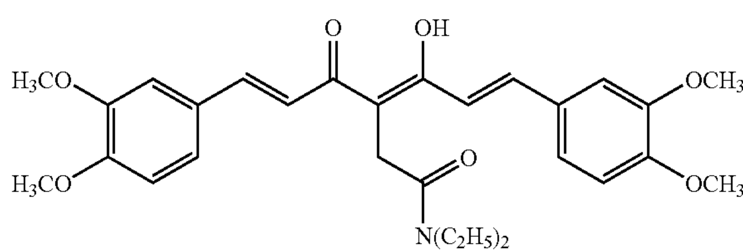
II-5
