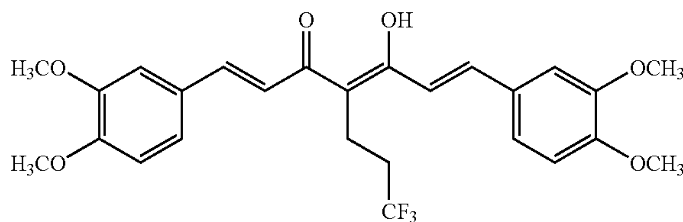
II-4
