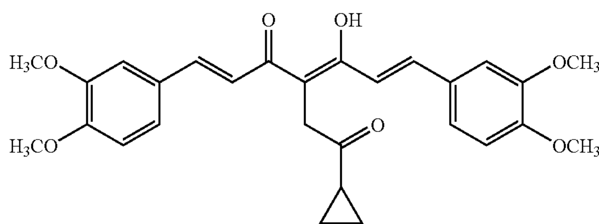
II-5
