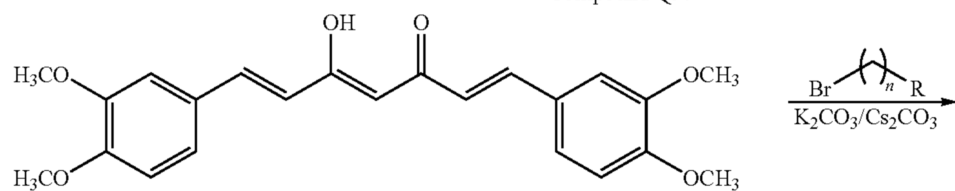
ASC-J9
