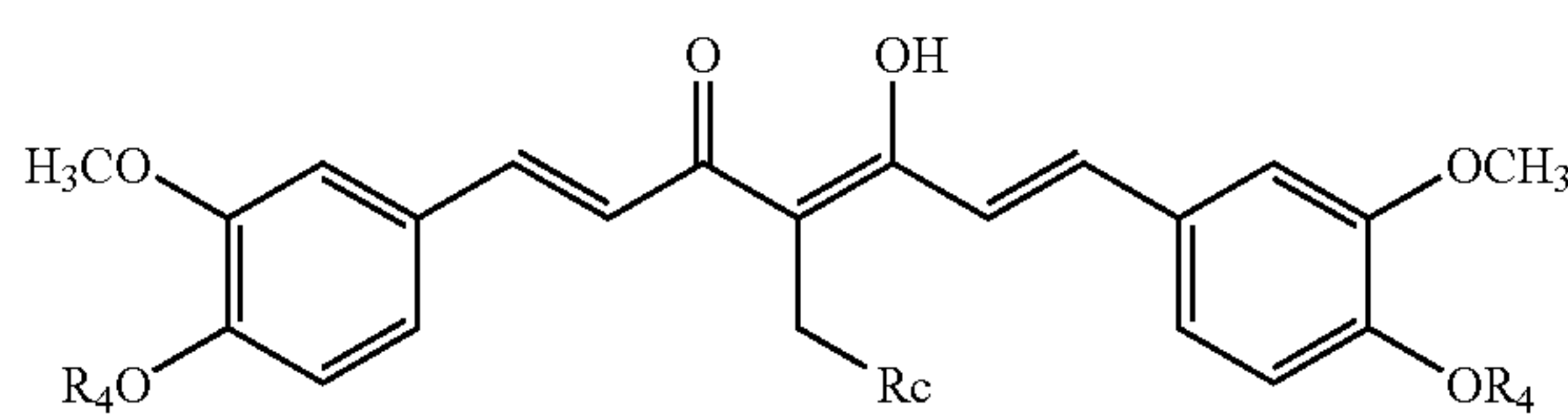
II-2
