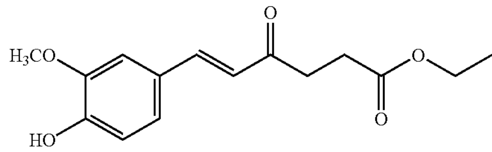
Monomer-7
