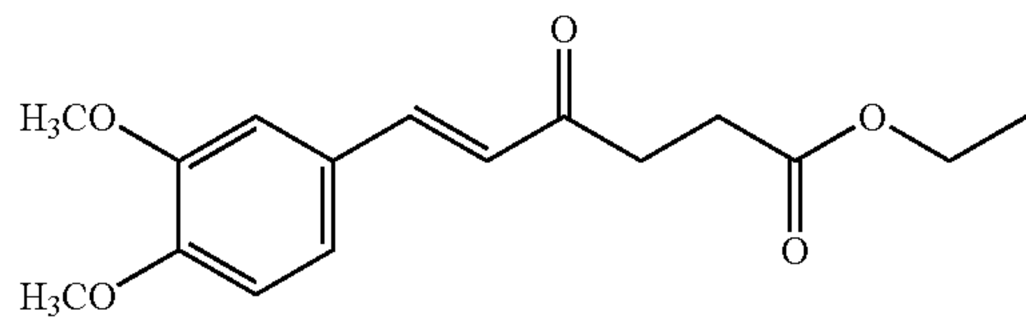
Monomer-6
