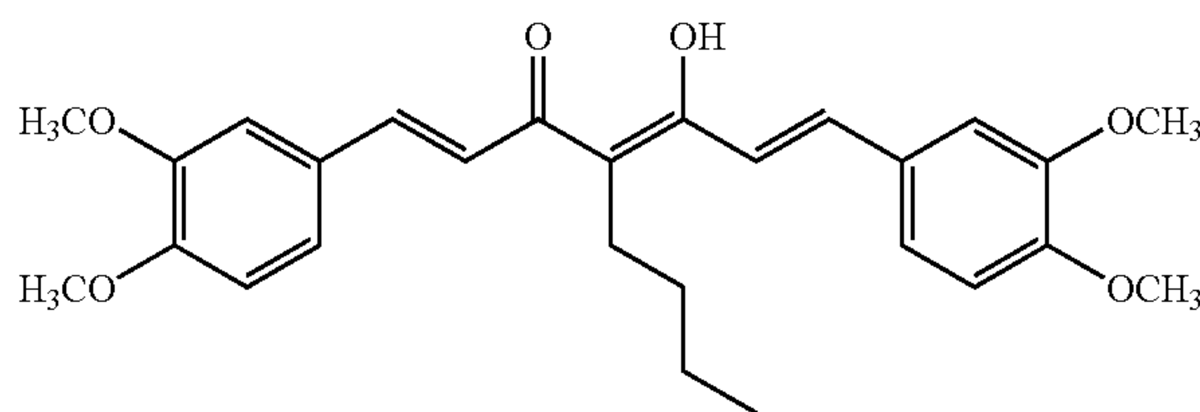
II-2
