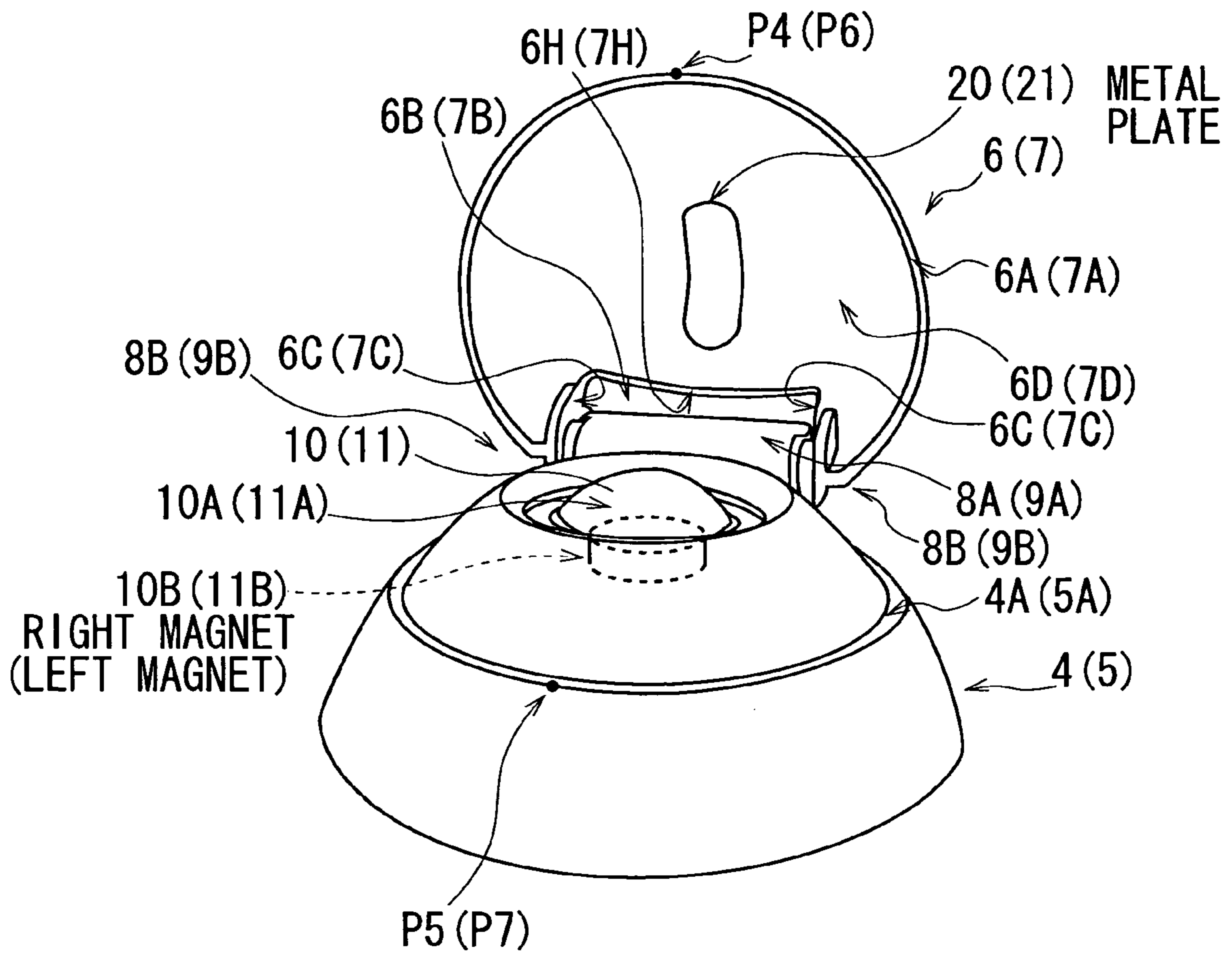
FIG. 5A
