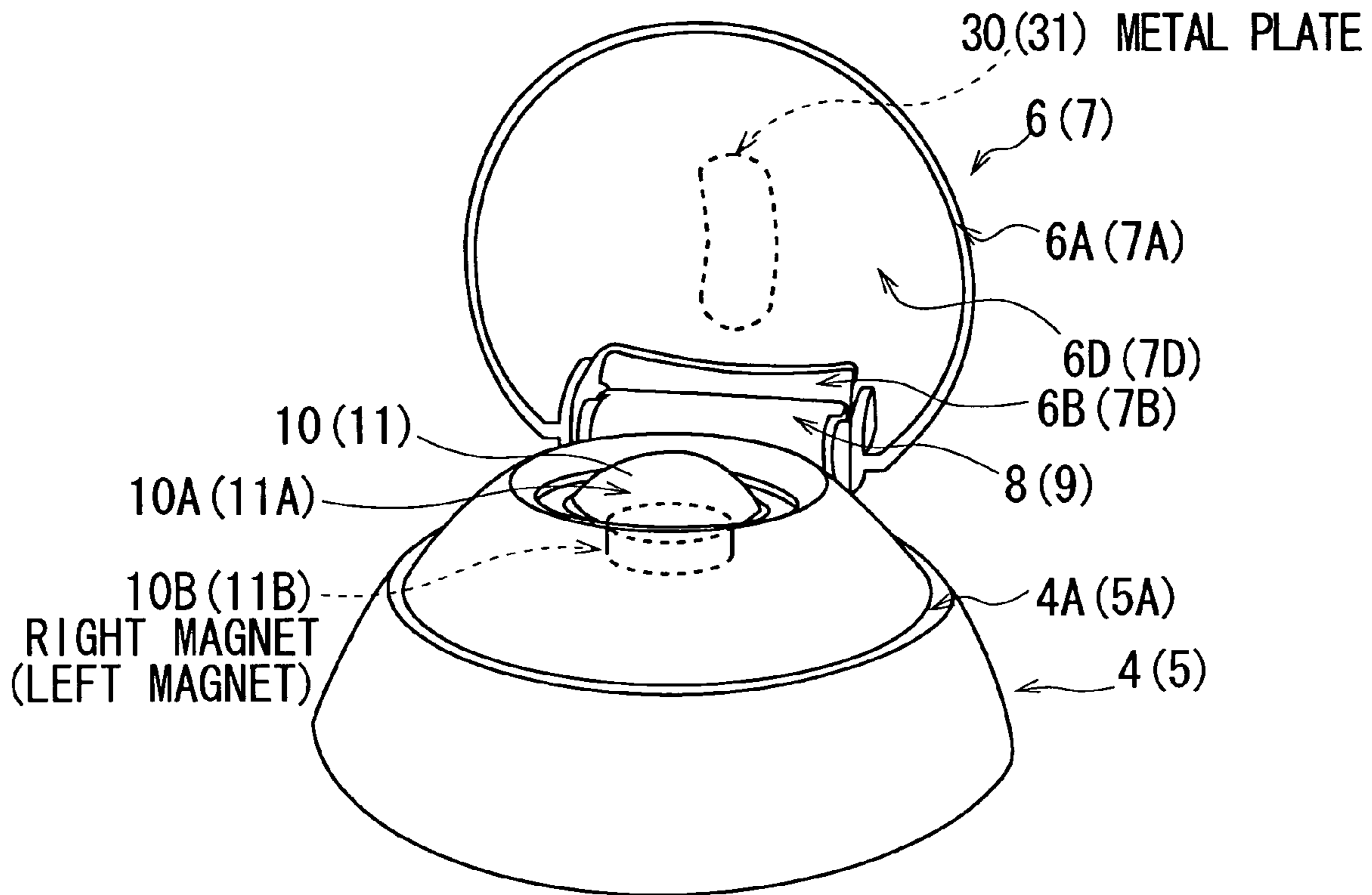
FIG. 8A
