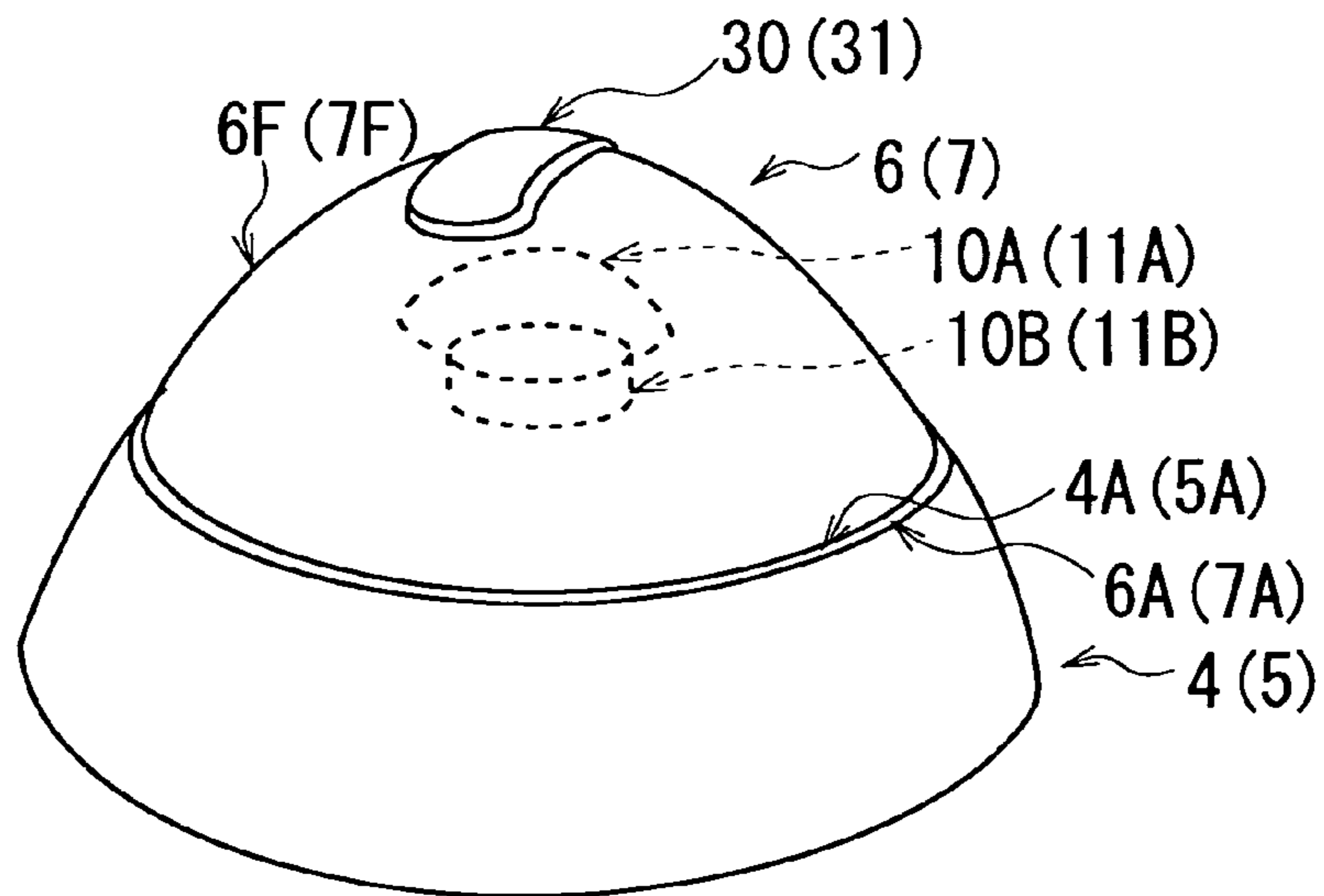
FIG. 8B
