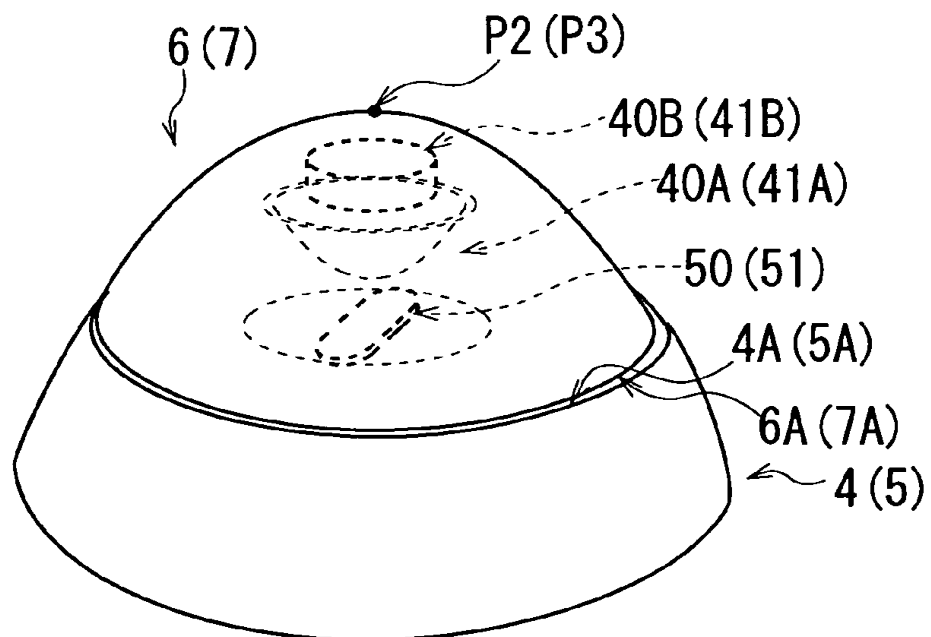
FIG. 10B
