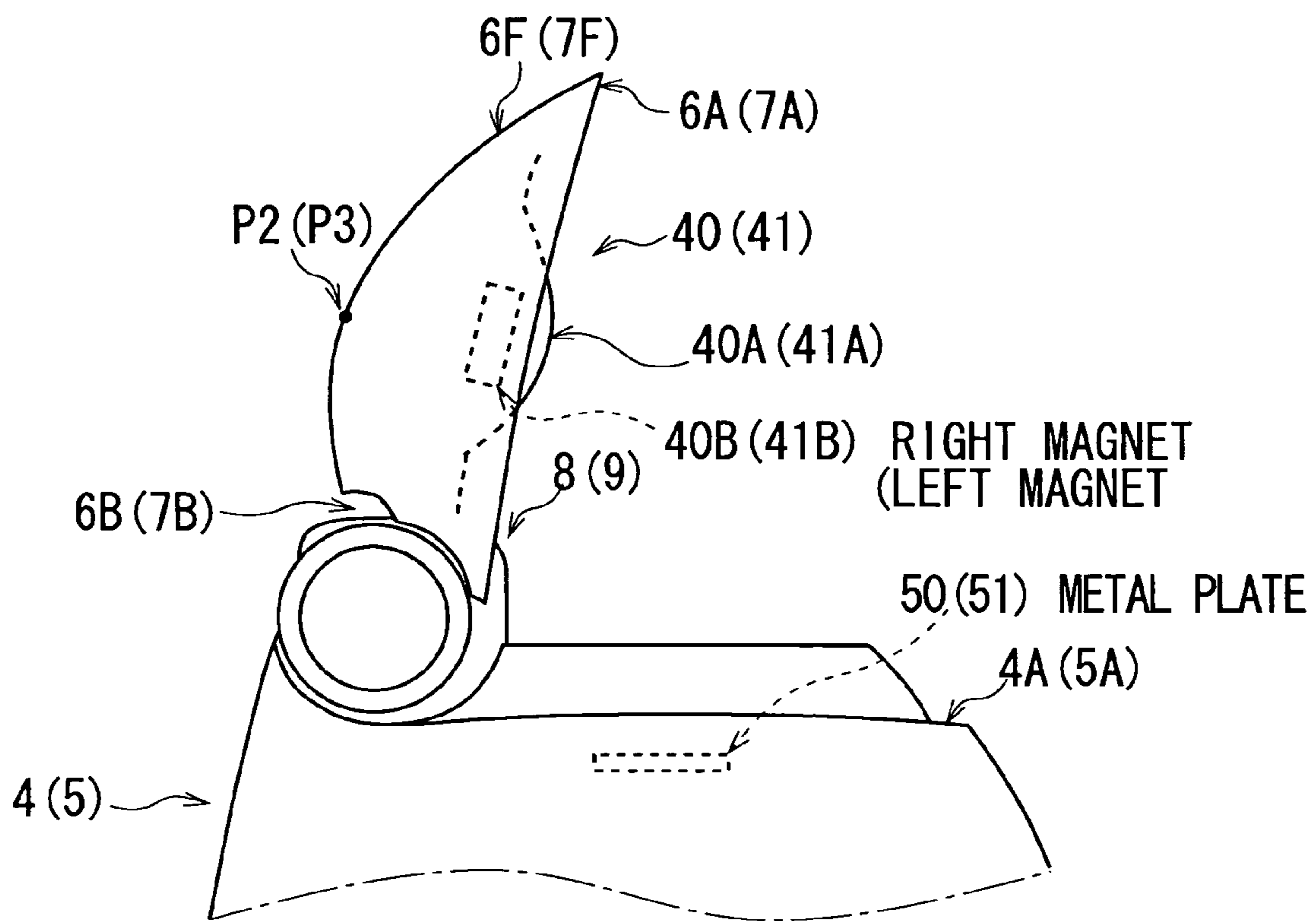
FIG. 11A
