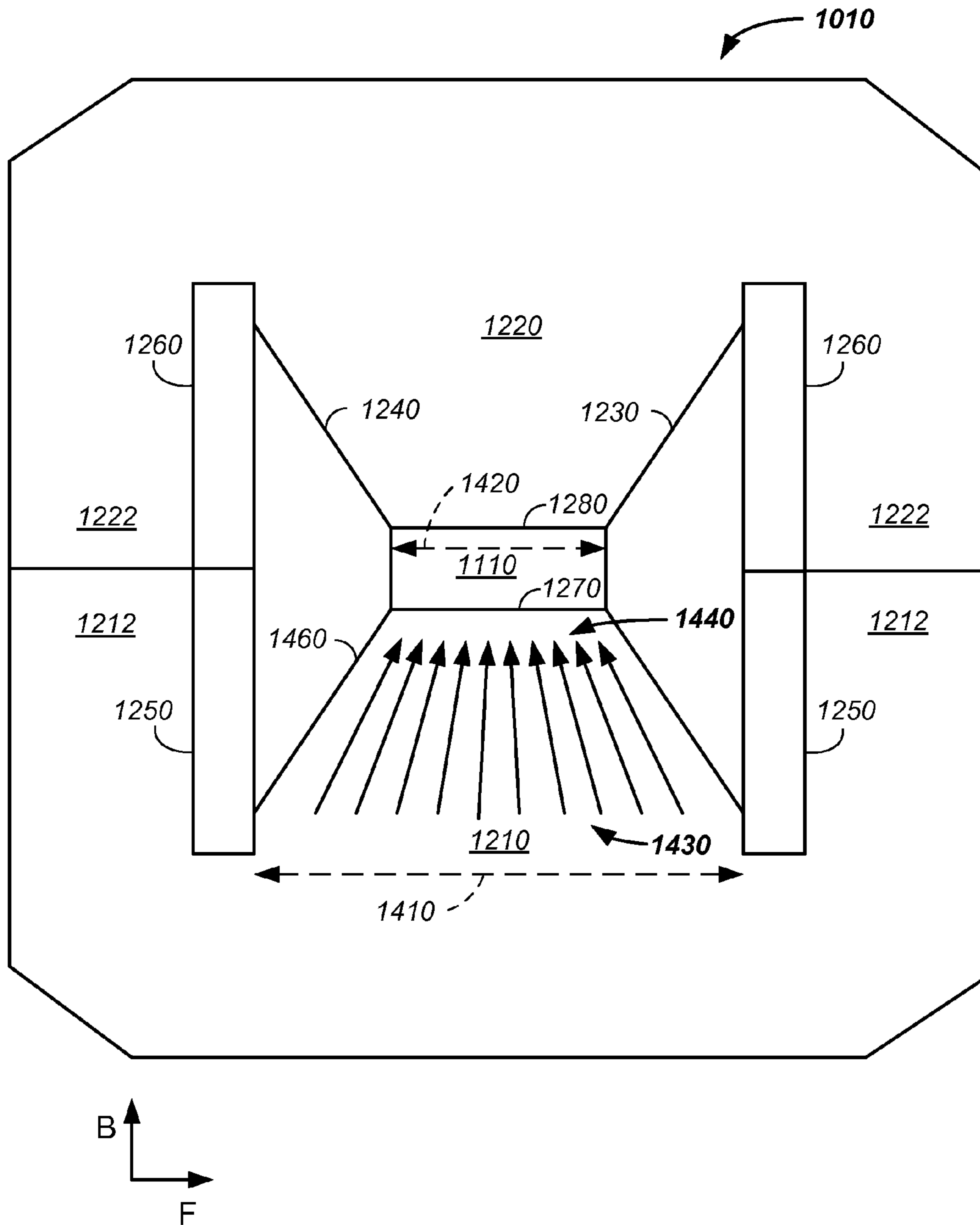
FIG. 14
