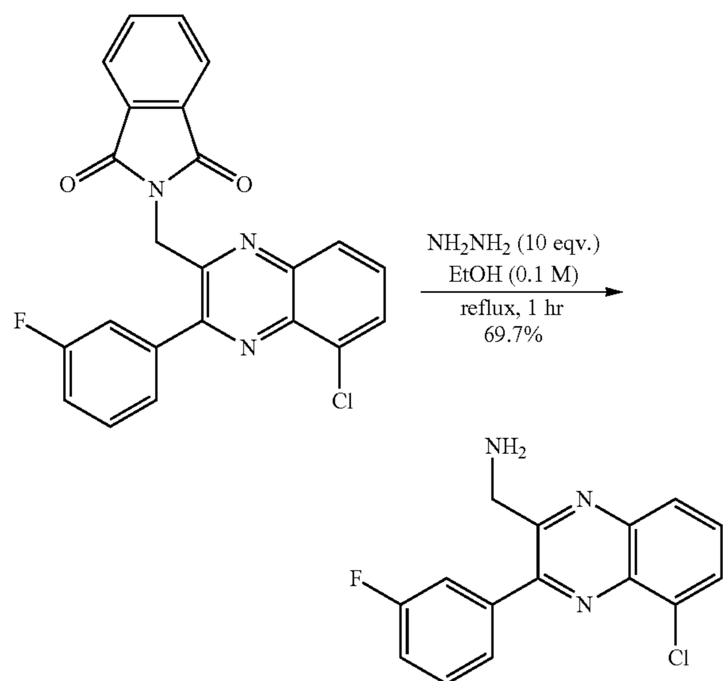
(5-Chloro-3-(3-fluorophenyl)quinoxalin-2-yl)methanamine
