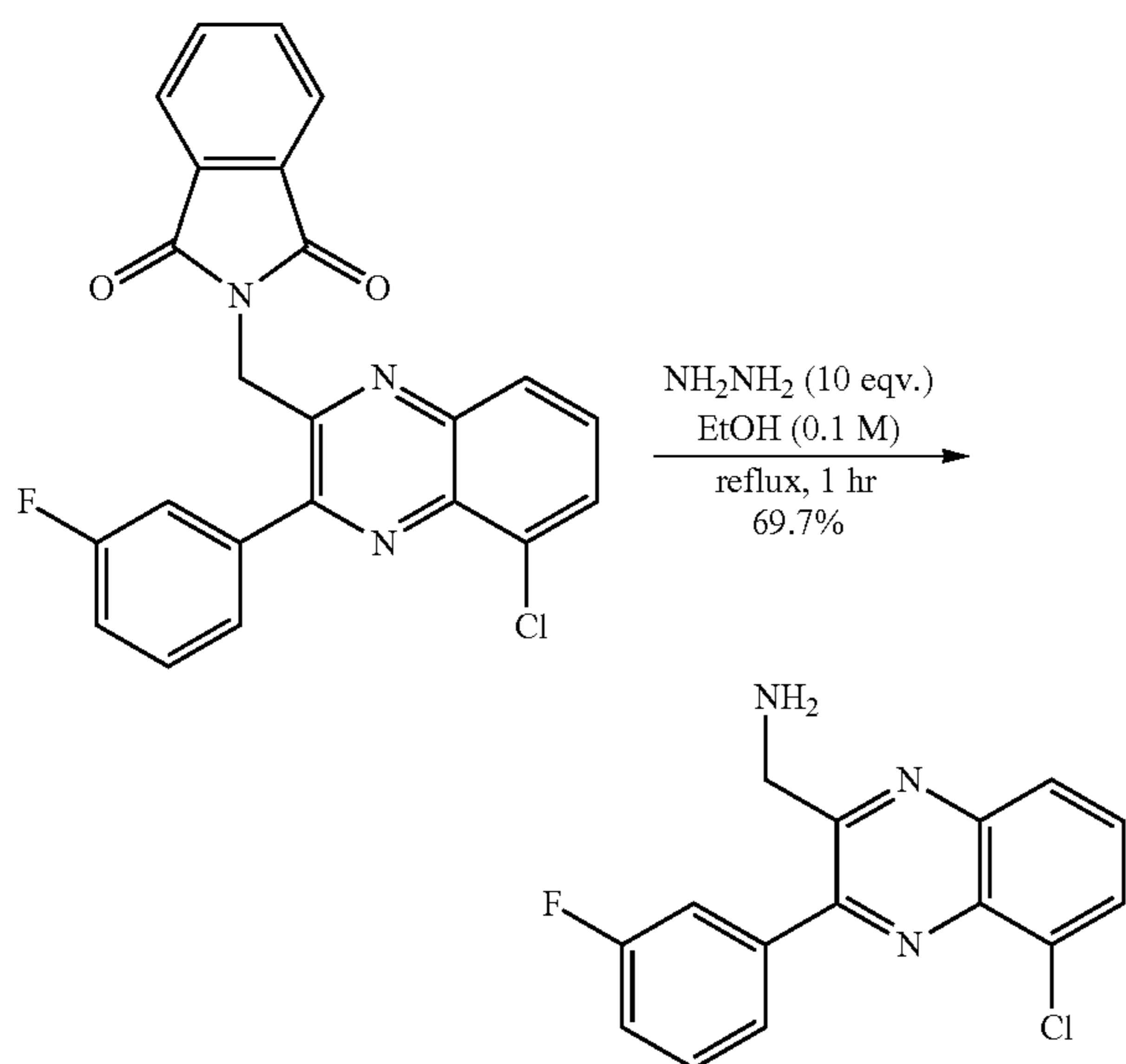
(5-Chloro-3-(3-fluorophenyl)quinoxalin-2-yl)methanamine
