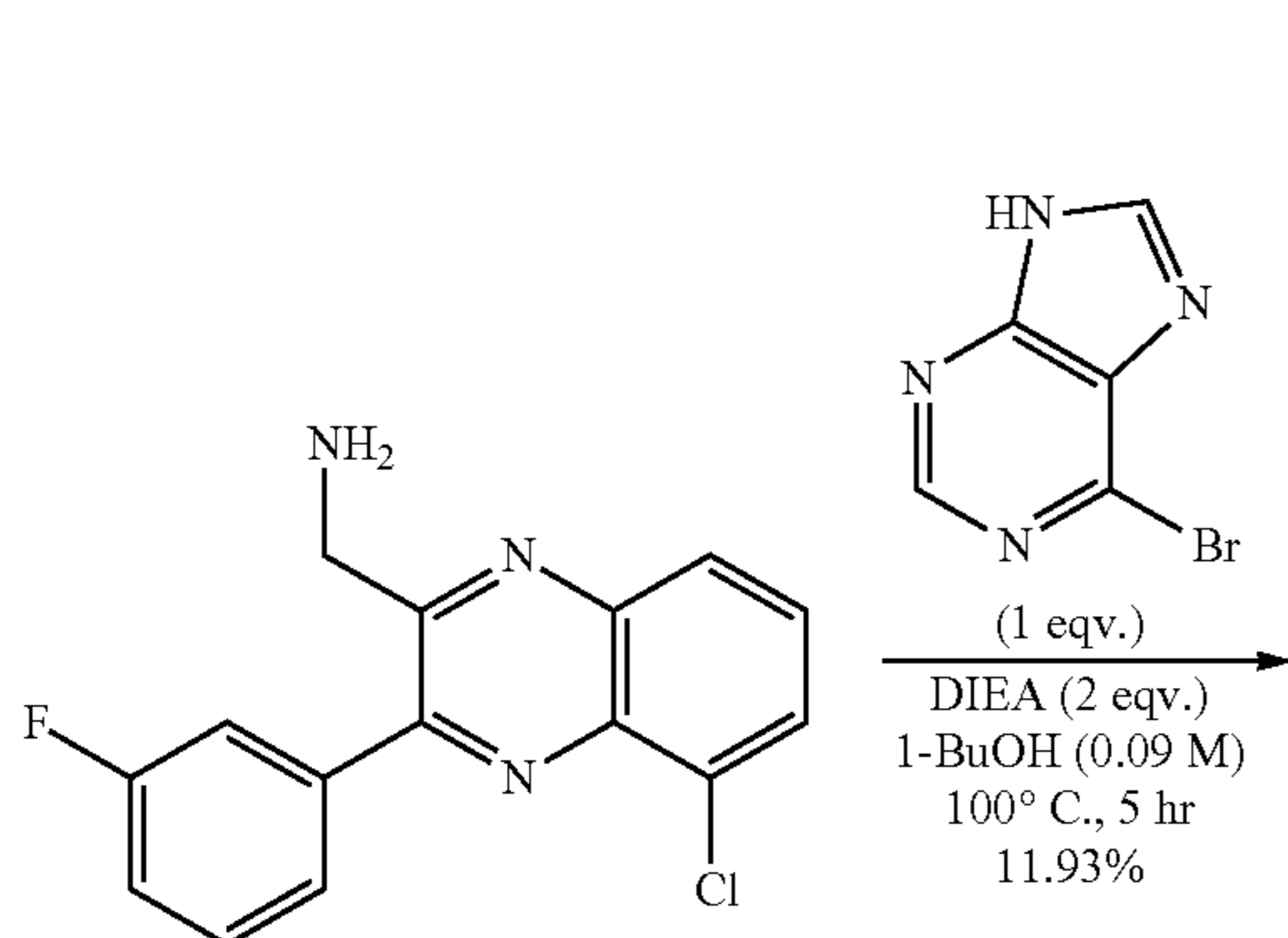
N-((5-Chloro-3-(3-fluorophenyl)quinoxalin-2-yl)methyl)-9H-purin-6-amine
