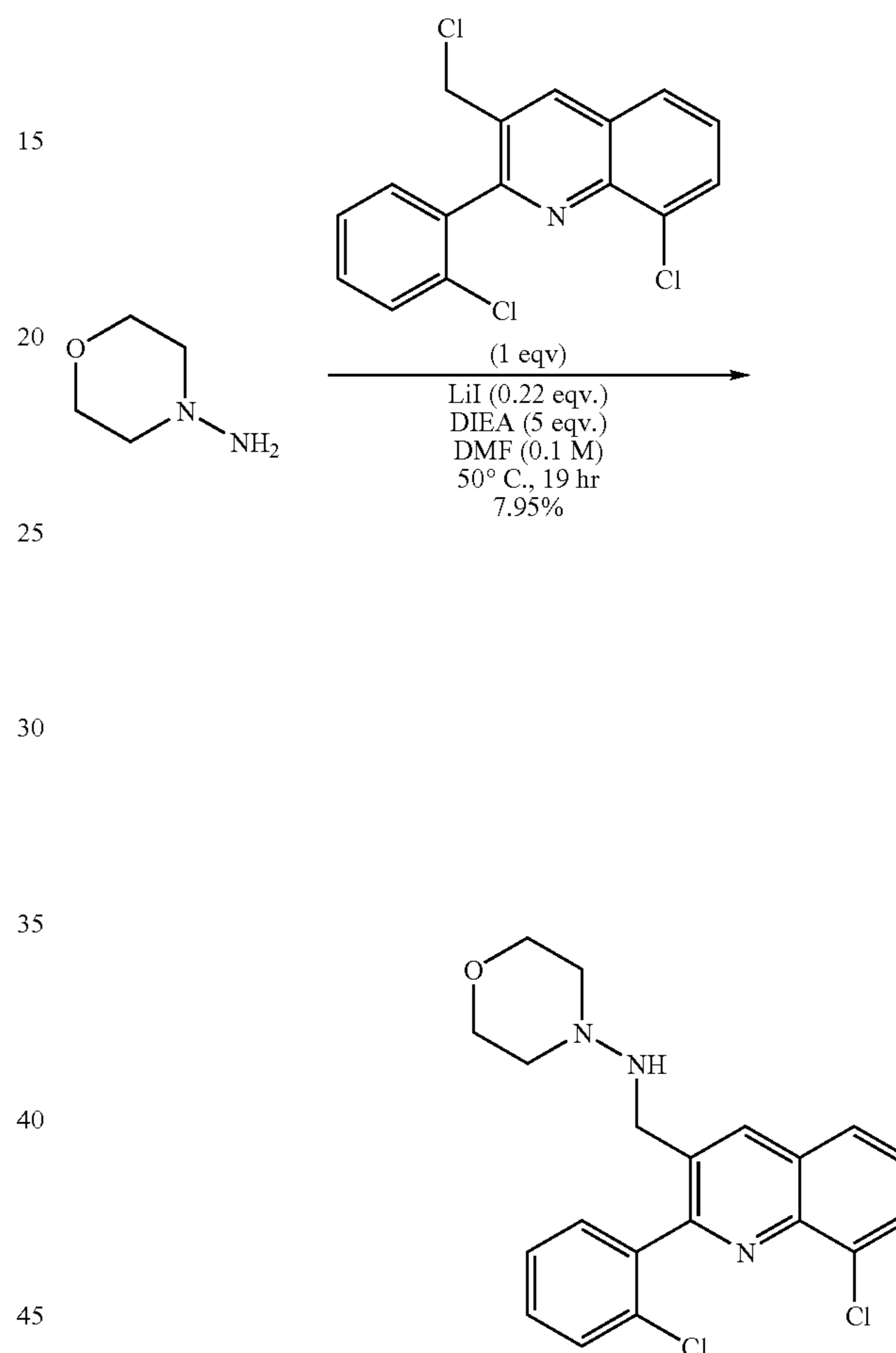
N-((5-Chloro-3-(2-chlorophenyl)quinoxalin-2-yl)methyl)-9H-purin-6-amine
