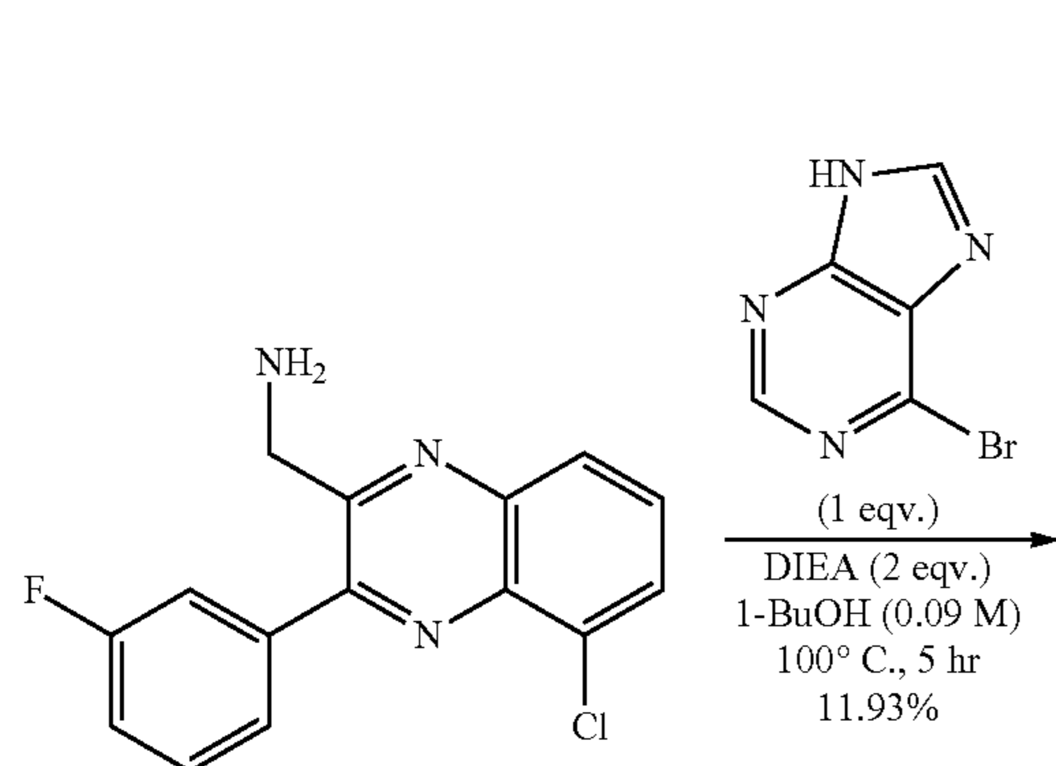
N-((5-Chloro-3-(3-fluorophenyl)quinoxalin-2-yl)methyl)-9H-purin-6-amine
