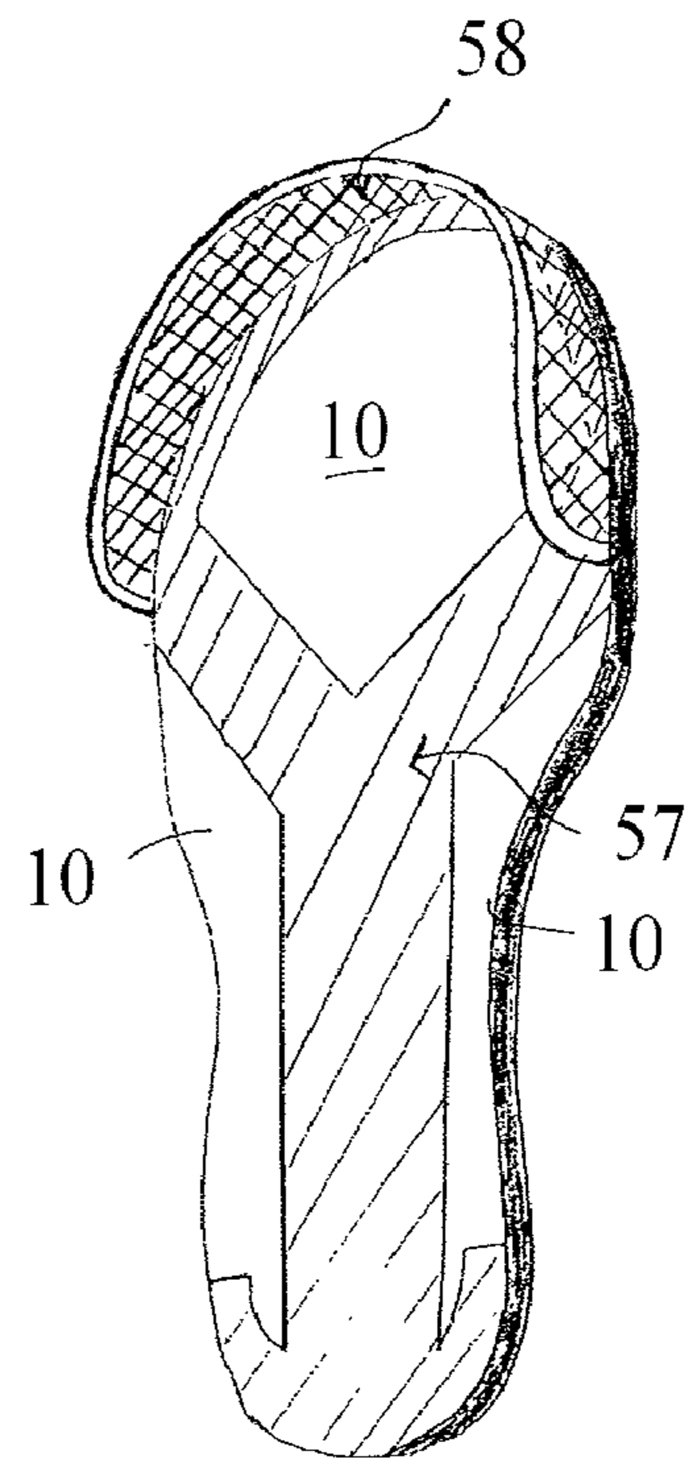
FIG. 8
