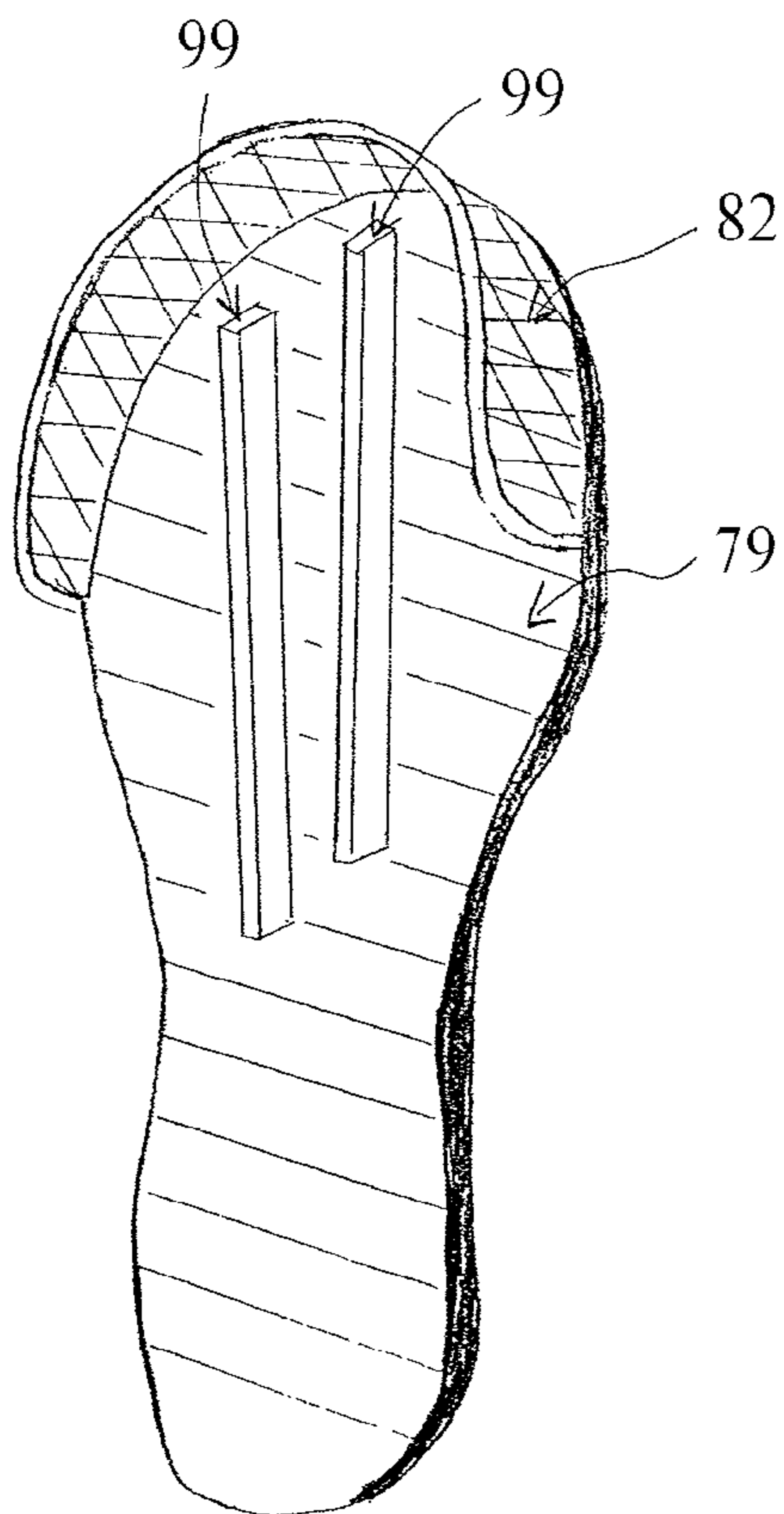
FIG. 15
