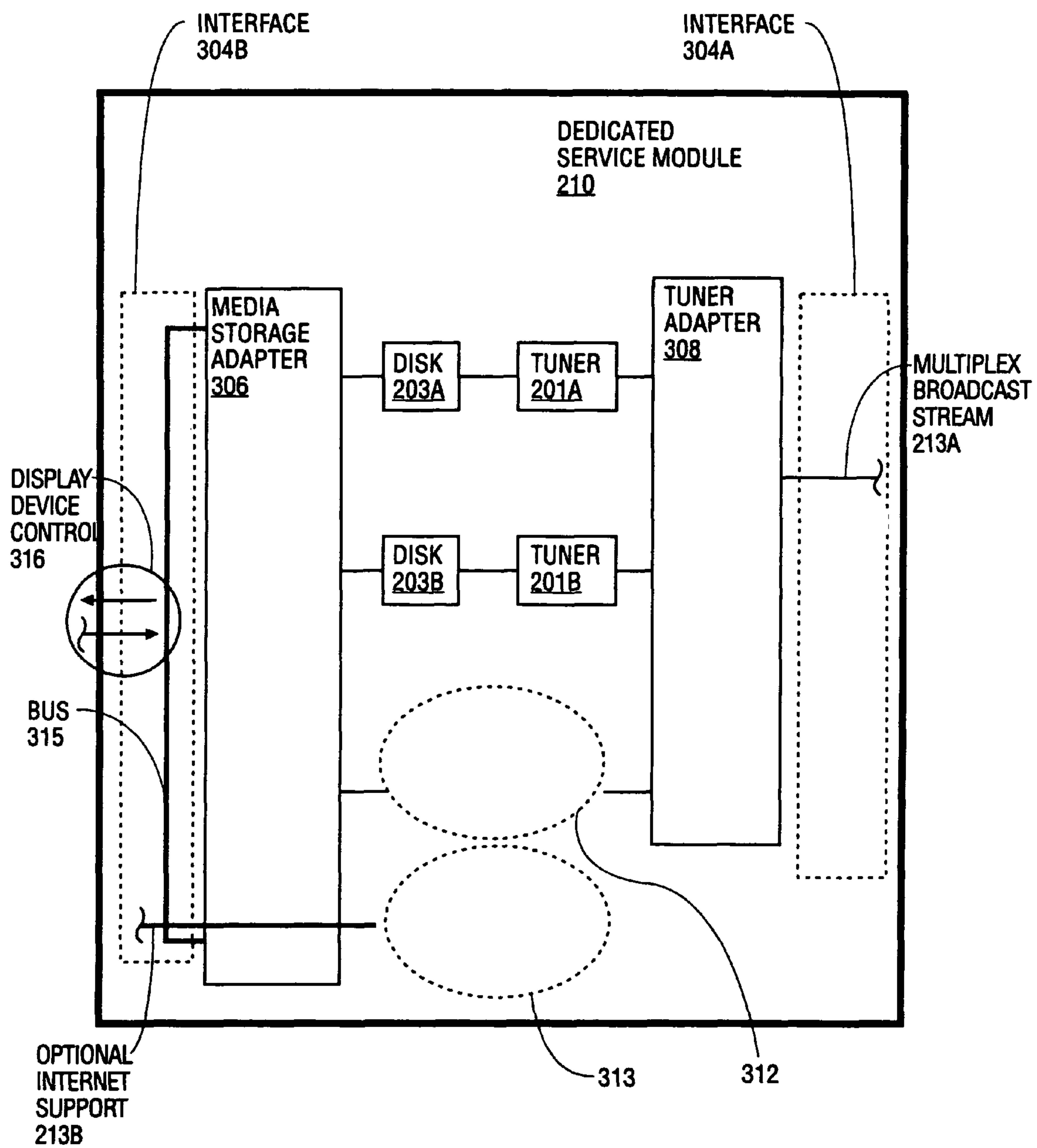
FIG. 3A
