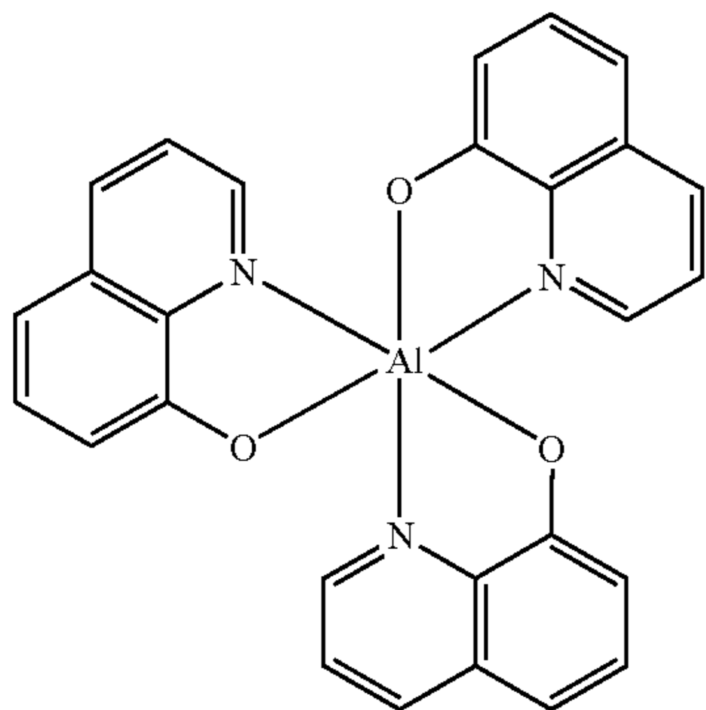
Alq
