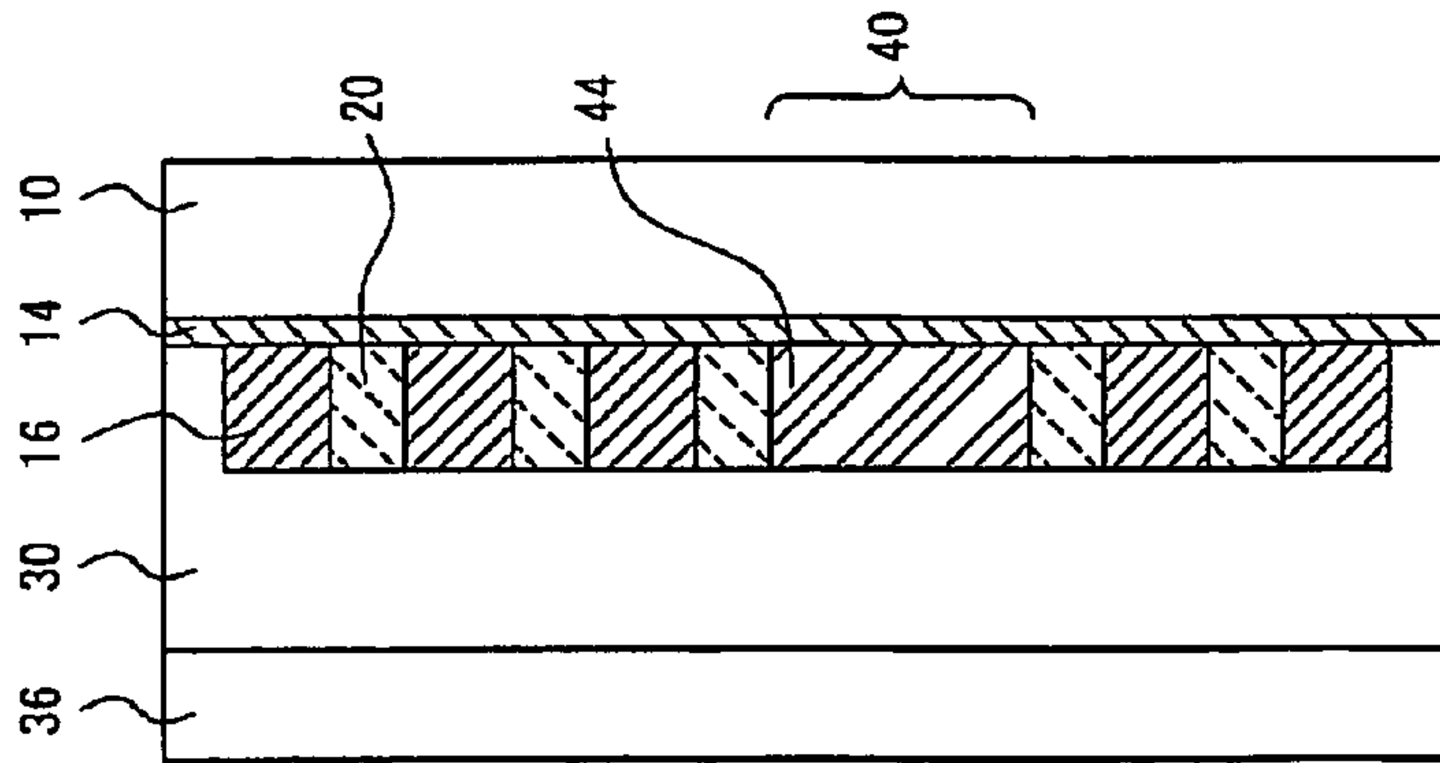
FIG. 10C
