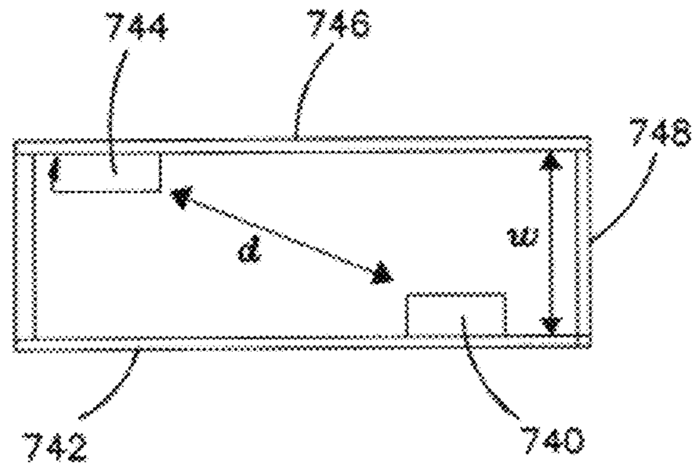
FIG. 27
