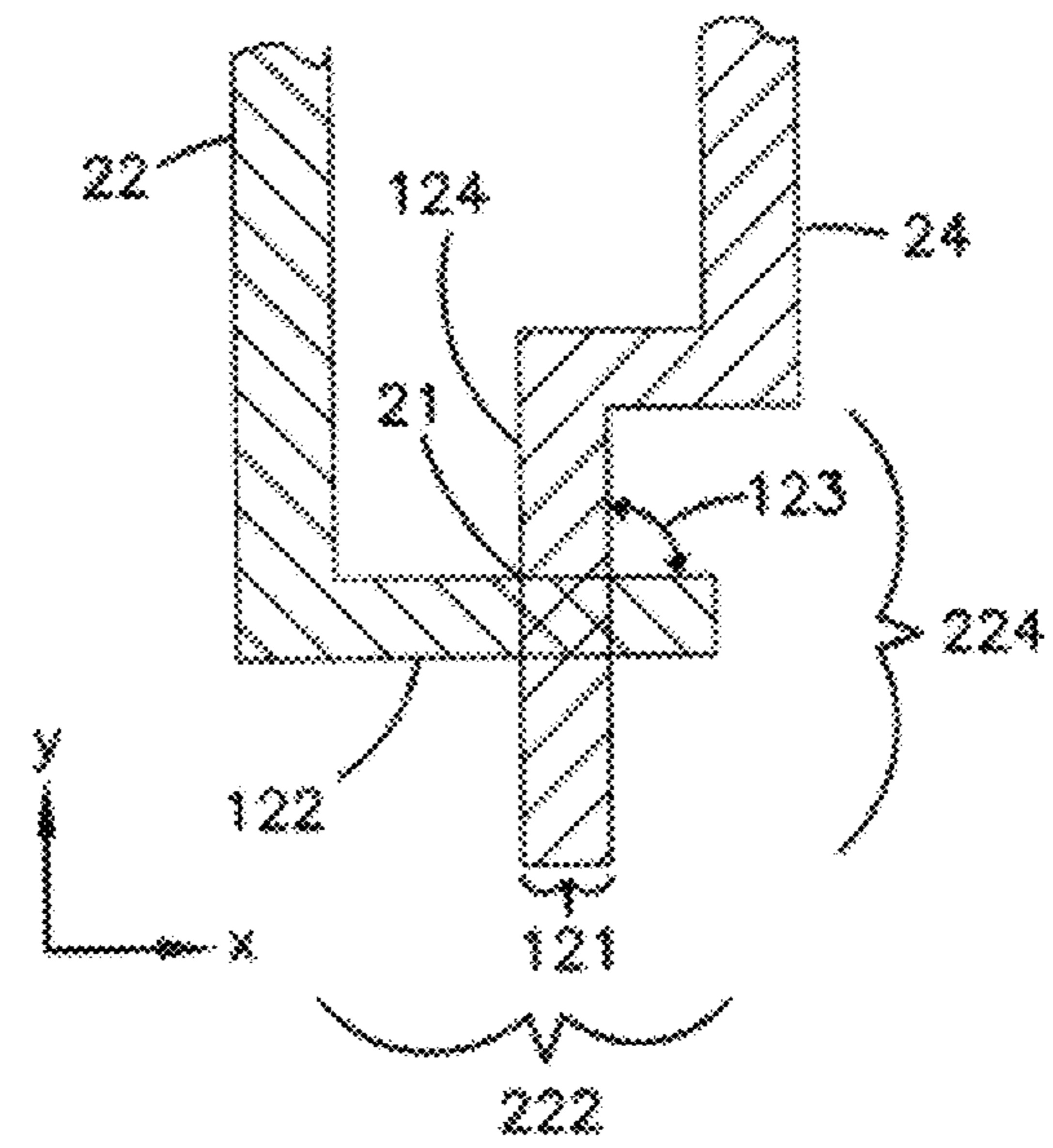
FIG. 11B
