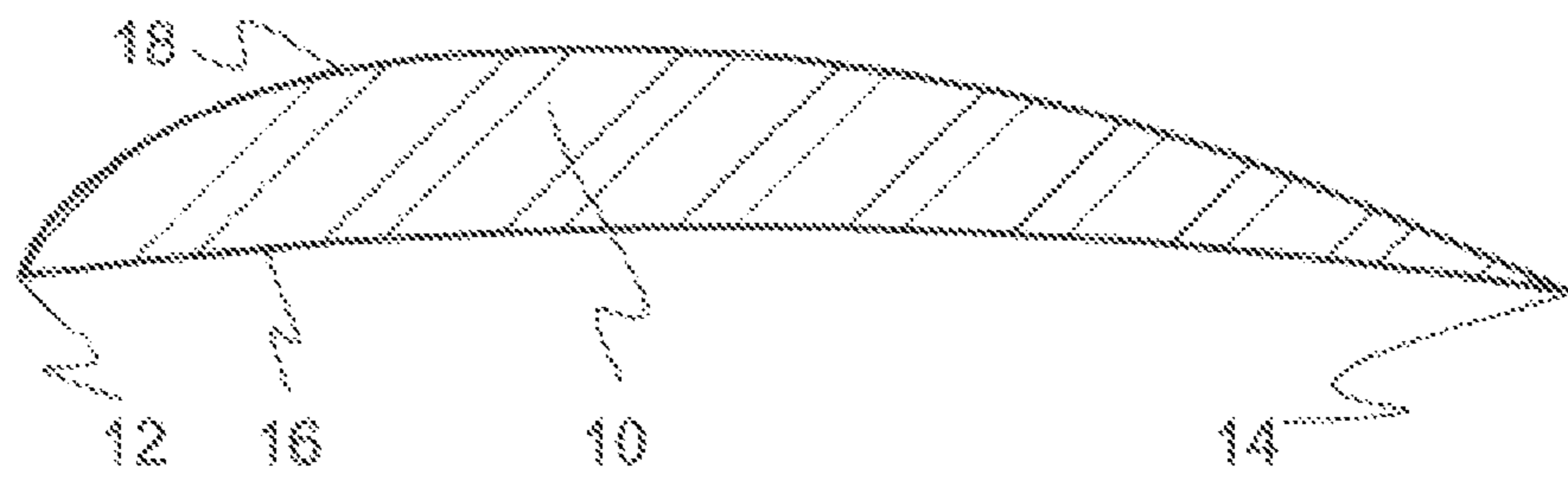
Fig. 1c (B - B)
