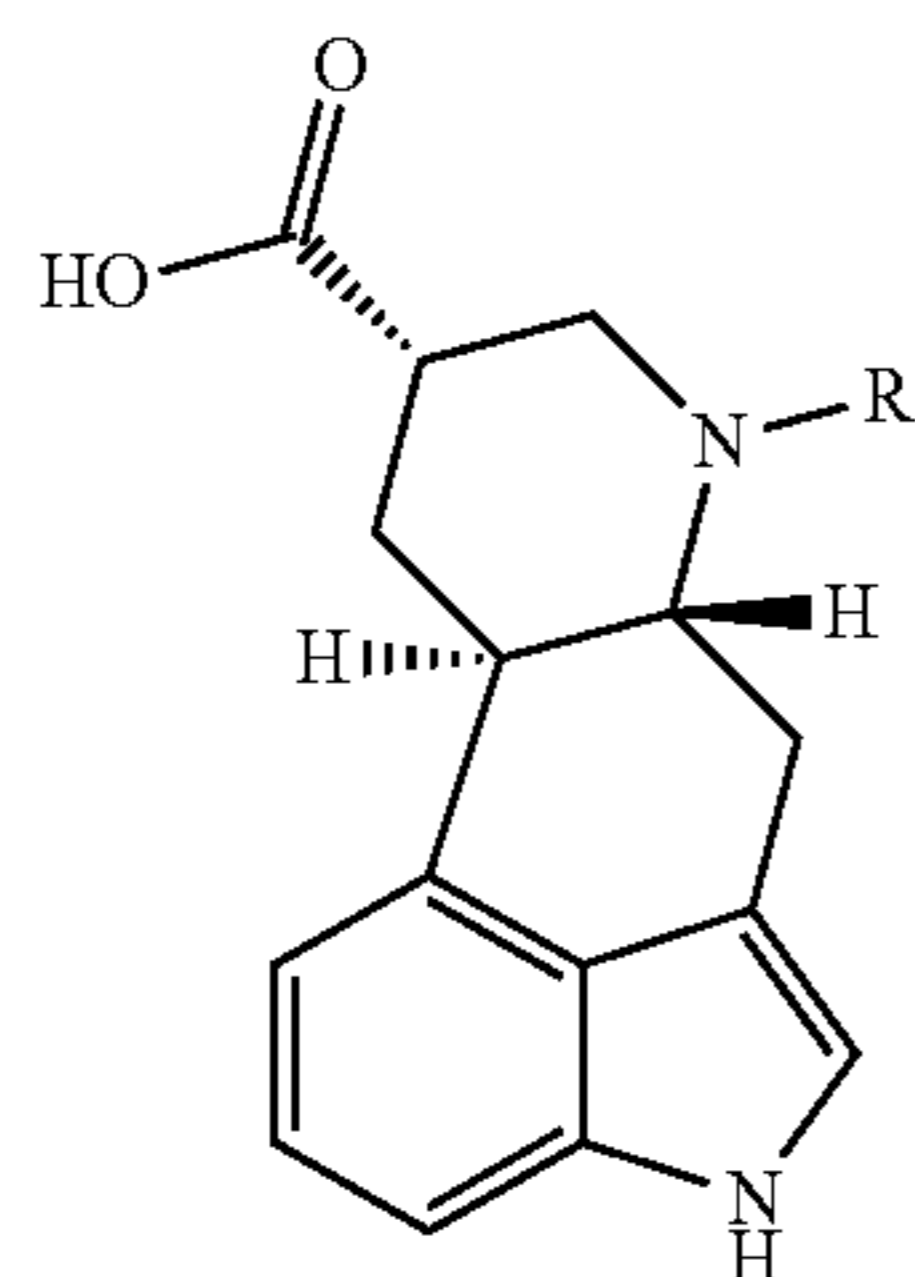
Scheme VI
