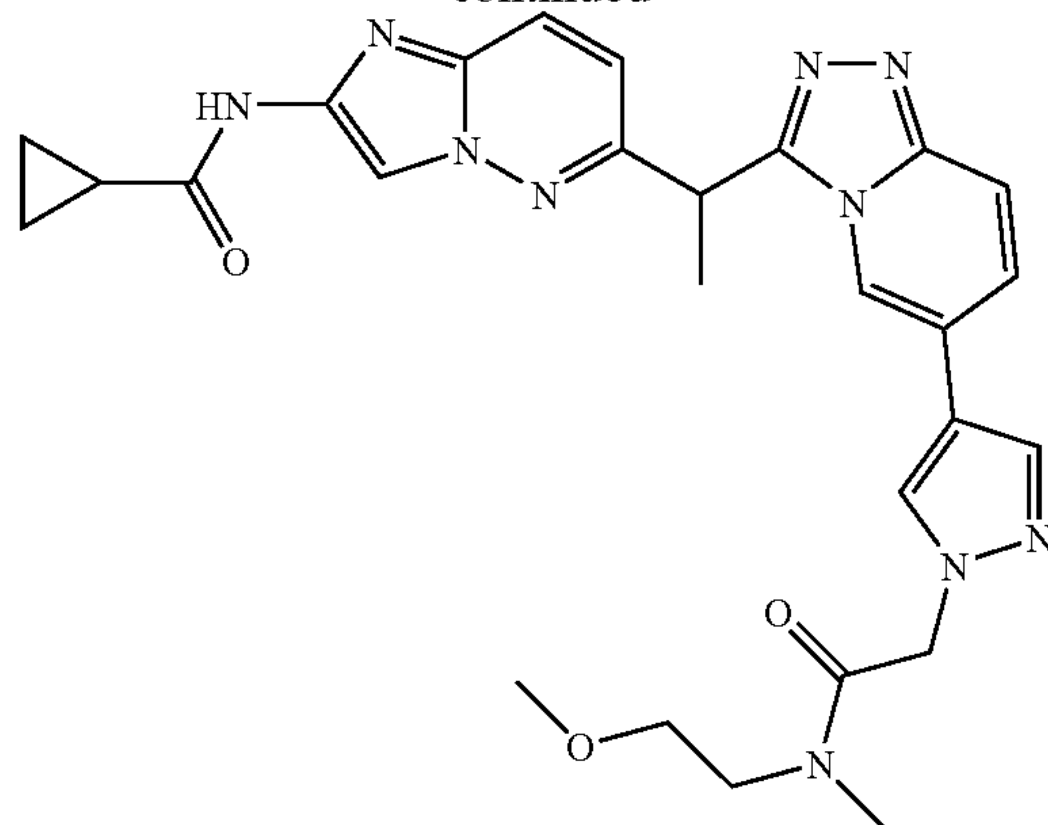
N-(6-(1-(6-(1-(2-((2-methoxyethyl)(methyl)amino)-2-oxoethyl)-1H-pyrazol-4-yl)-[1,2,4]triazolo[4,3-a]pyridin-3-yl)ethyl)imidazo[1,2-b]pyridazin-2-yl)cyclopropanecarboxamide
