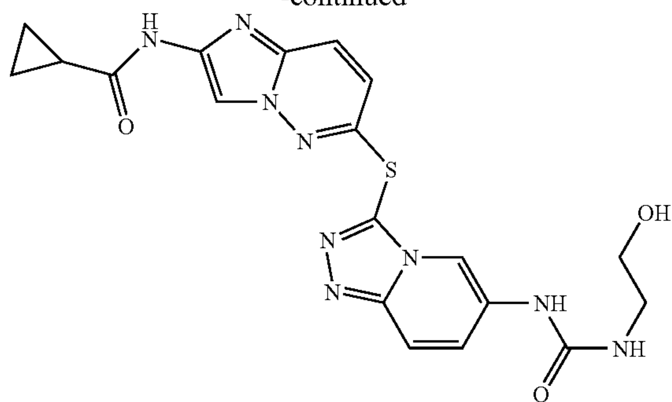
N-(6-(6-(3-(2-hydroxyethyl)ureido)-[1,2,4]triazolo[4,3-a]pyridin-3-ylthio)imidazo[1,2-b]pyridazin-2-yl)cyclopropanecarboxamide
