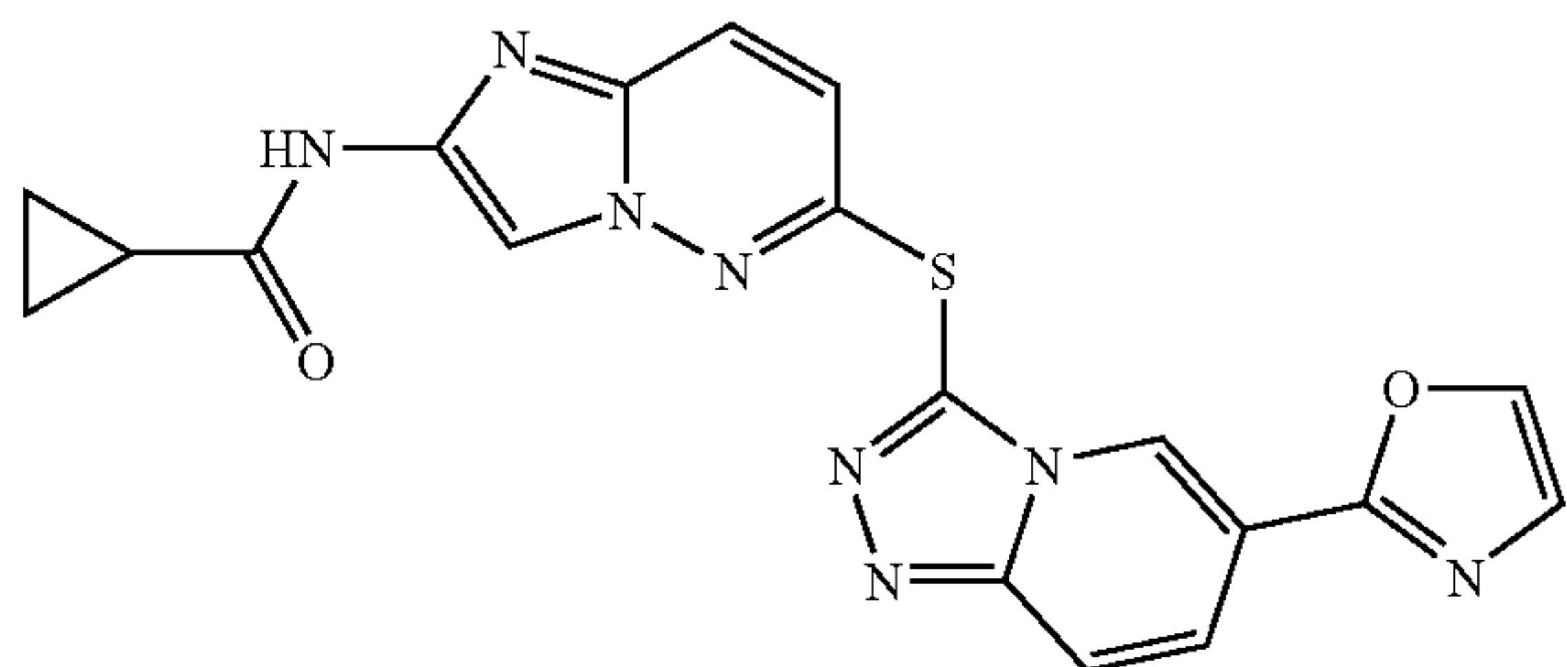
N-(6-(6-(oxazol-2-yl)-[1,2,4]triazolo[4,3-a]pyridin-3-ylthio)imidazo[1,2-b]pyridazin-2-yl)cyclopropanecarboxamide
