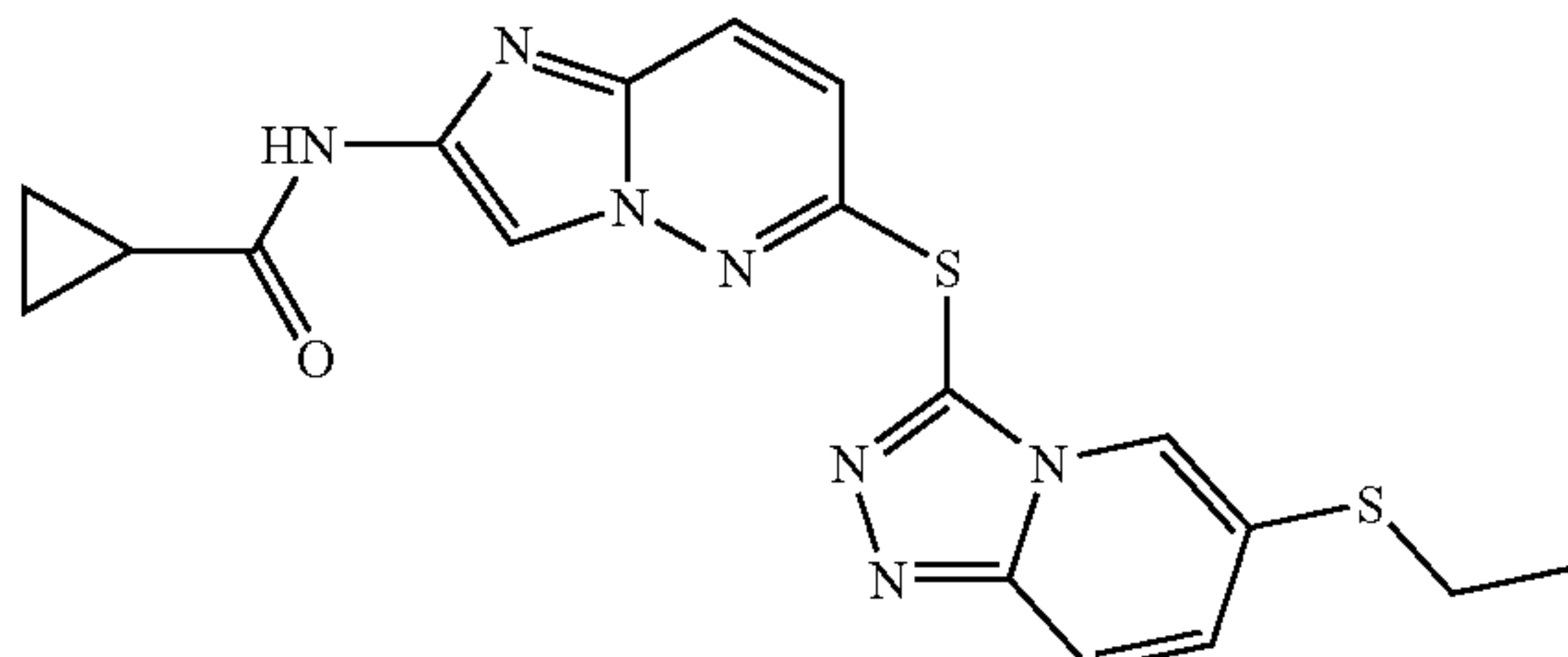
N-(6-(6-ethylthio)-[1,2,4]triazolo[4,3-a]pyridin-3-ylthio)imidazo[1,2-b]pyridazin-2-yl)cyclopropanecarboxamide
