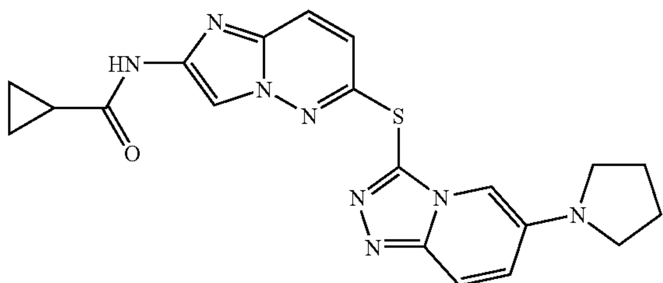
N-(6-(6-(pyrrolidin-1-yl)-[1,2,4]triazolo[4,3-a]pyridin-3-ylthio)imidazo[1,2-b]pyridazin-2-yl)cyclopropanecarboxamide
