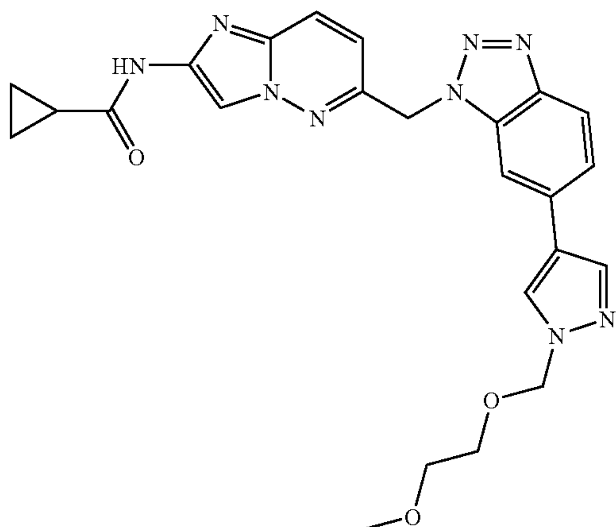
N-(6-(((6-((2-methoxyethoxy)methyl)-1H-pyrazol-4-yl)-1H-benzo[d][1,2,3]triazol-1-yl)methyl)imidazo[1,2-b]pyridazin-2-yl)cyclopropanecarboxamide
