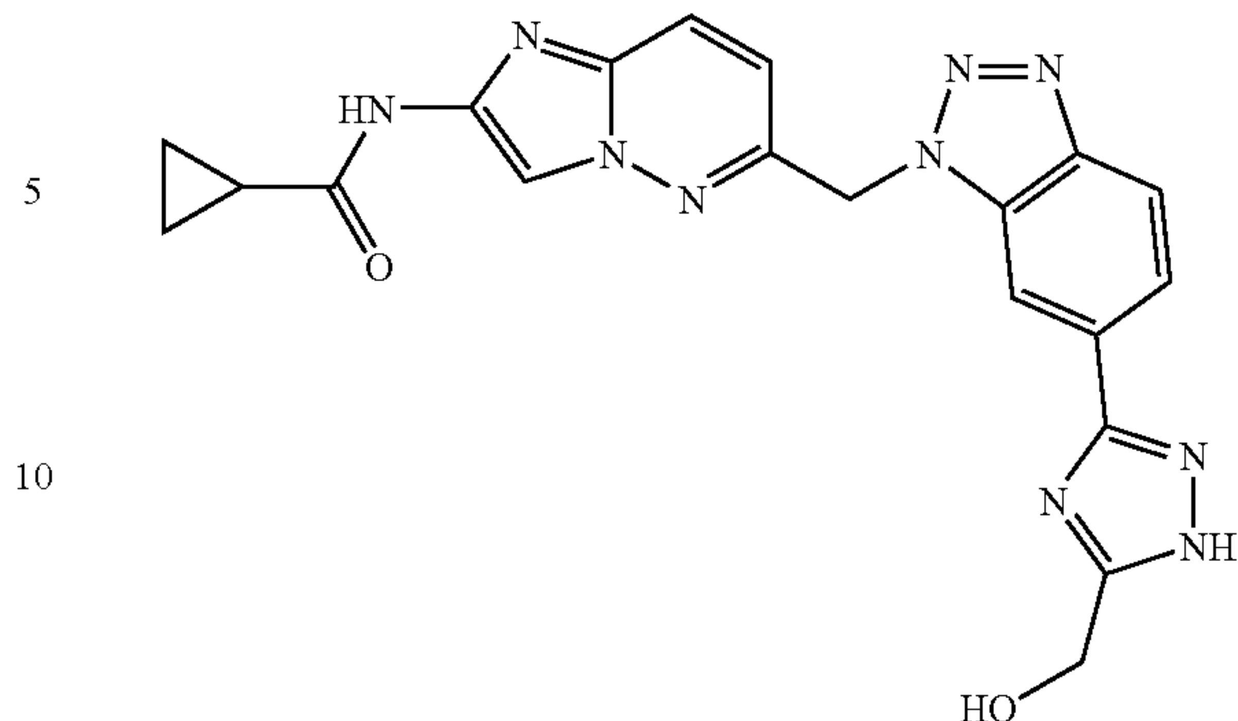
N-(6-((6-(5-(hydroxymethyl)-1H-1,2,4-triazol-3-yl)-1H-benzo[d][1,2,3]triazol-1-yl)methyl)imidazo[1,2-b]pyridazin-2-yl)cyclopropanecarboxamide
