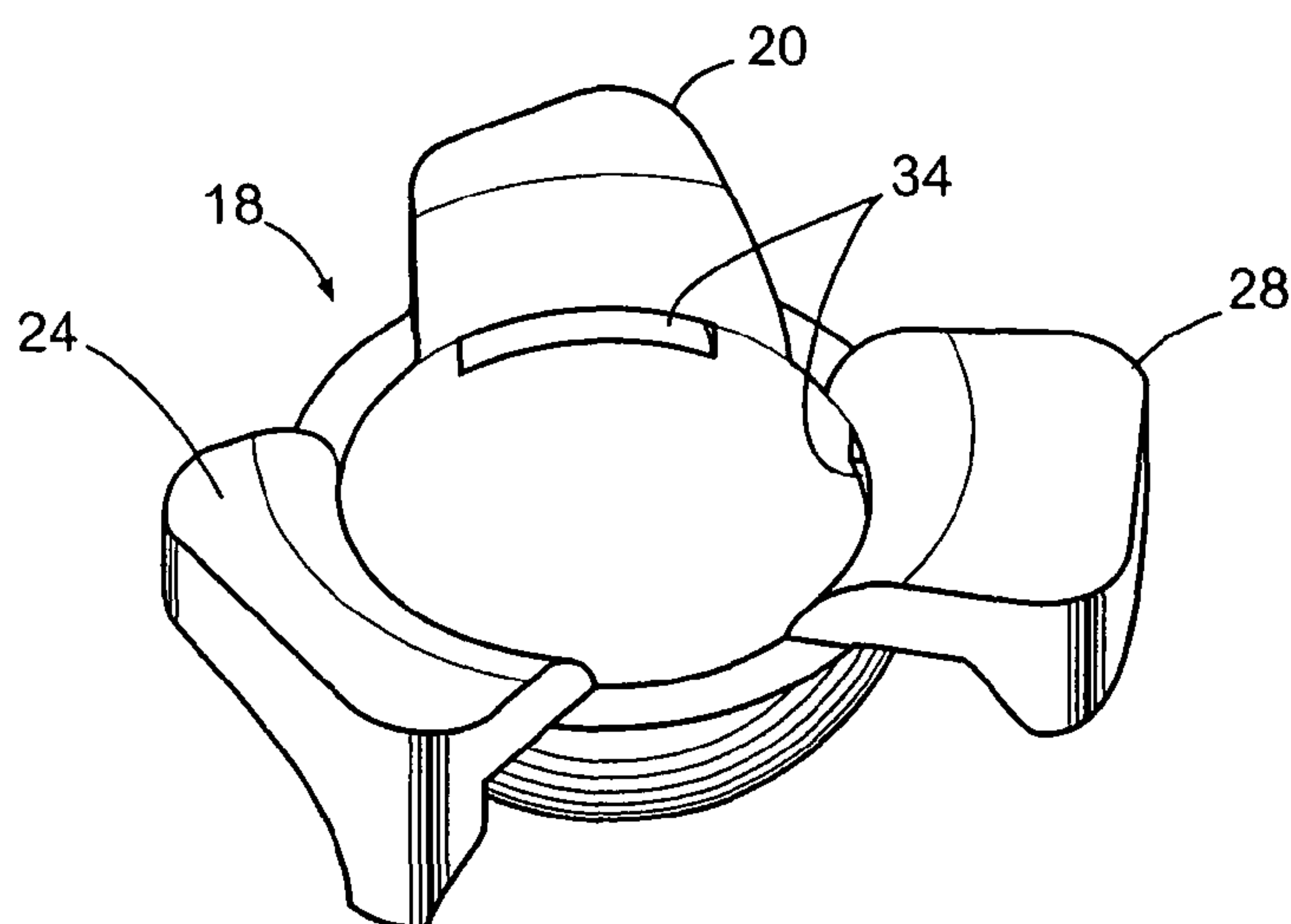
FIG. 4c
