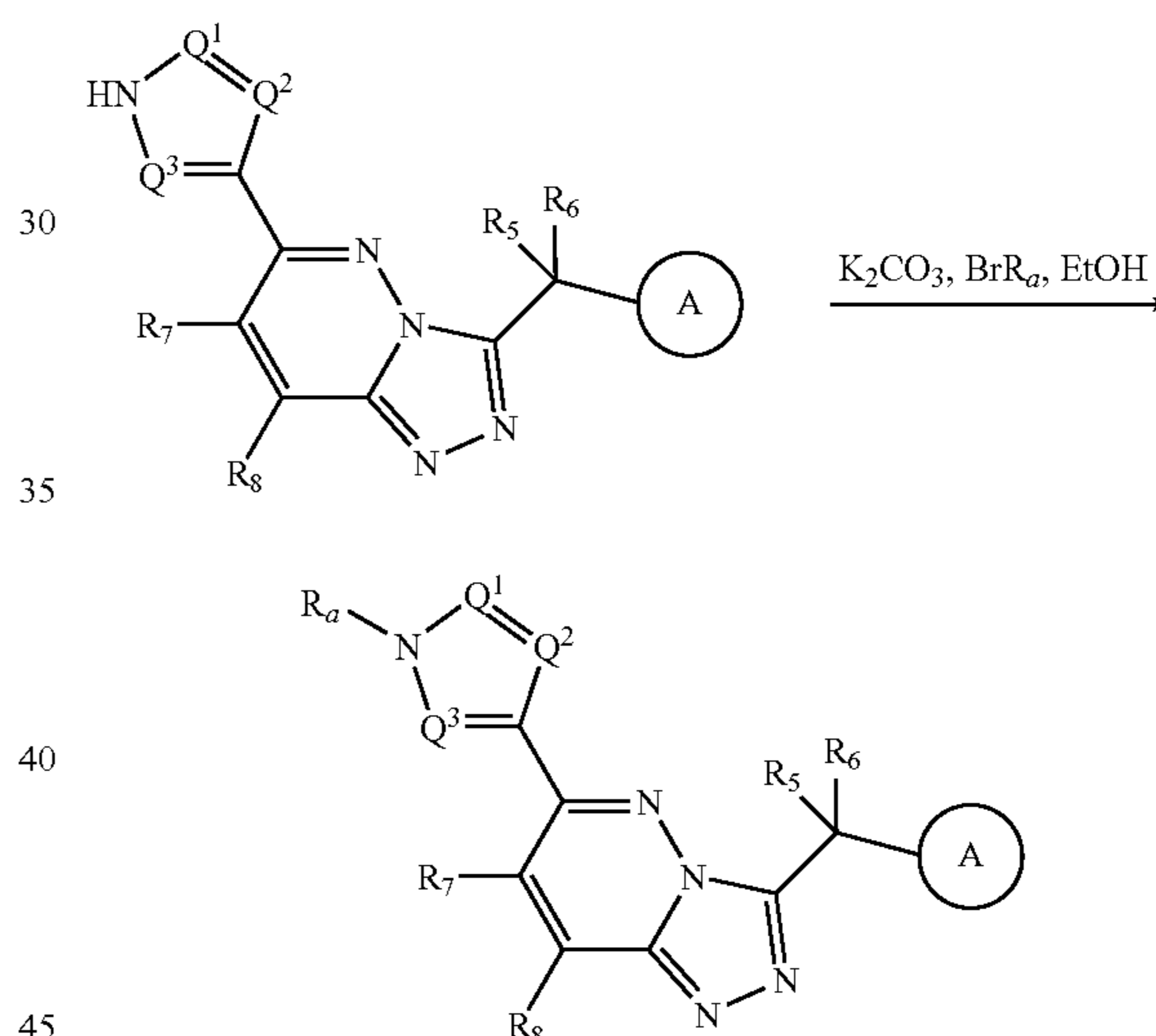
Scheme 5e
