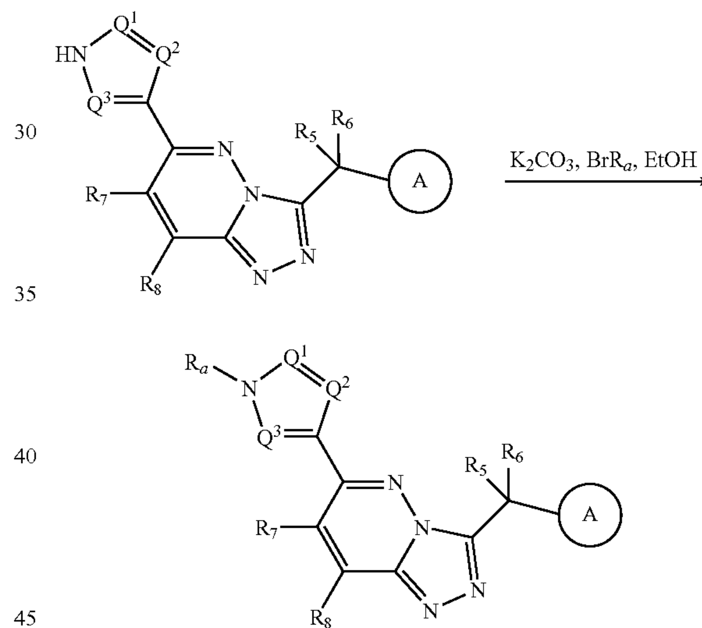
Scheme 5e
